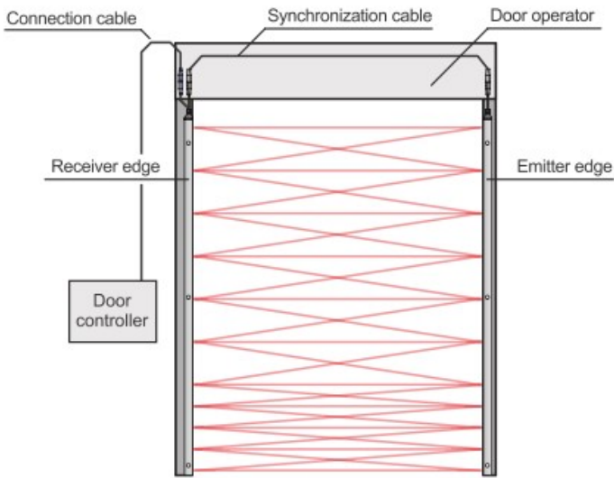
Figura 1. Esquema de la cortina de fotocèl·lules
