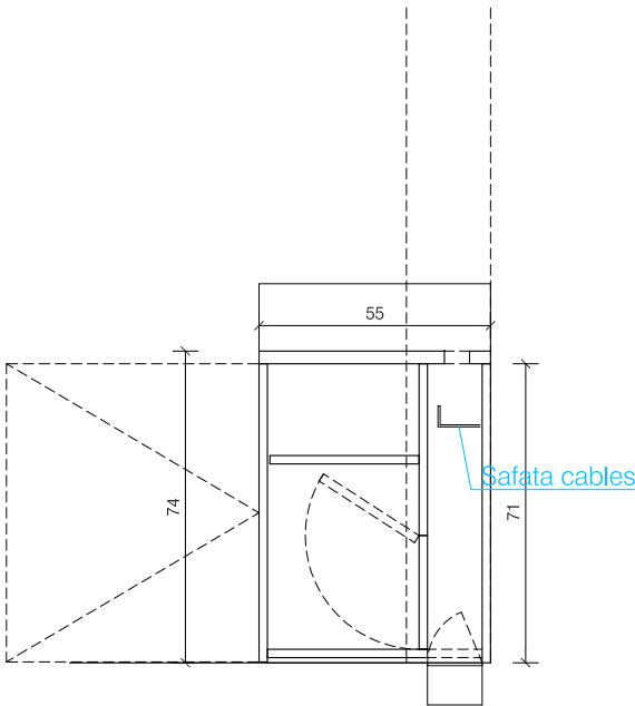
SECCIÓ MOBLE C
