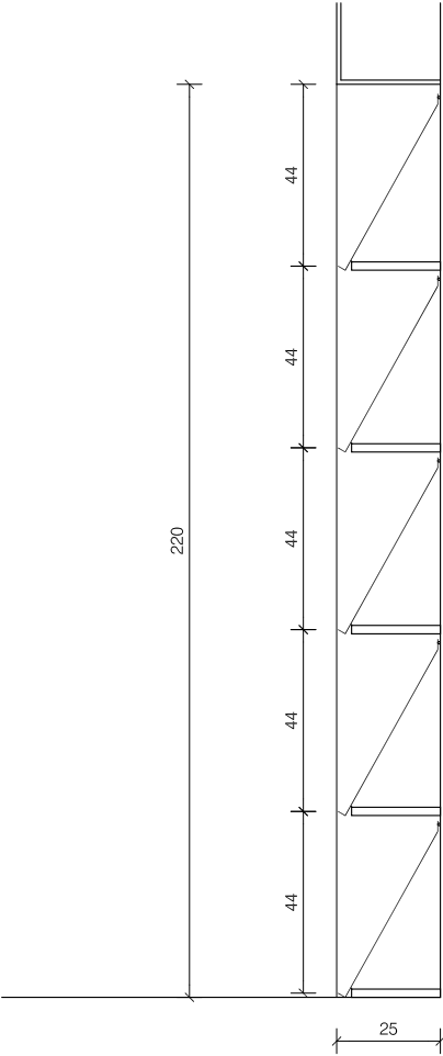
SECCIÓ
