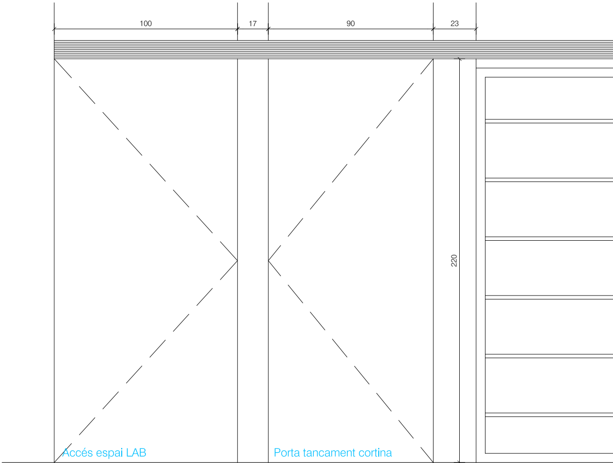
ALÇAT
