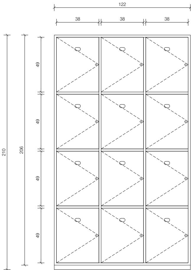
ALÇAT
