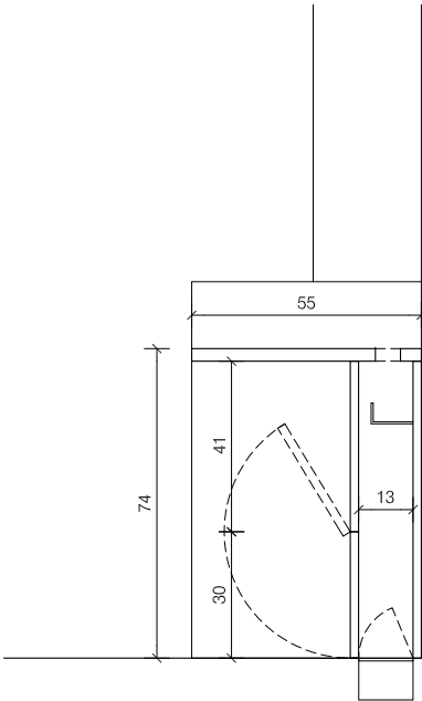
SECCIÓ MOBLE B
