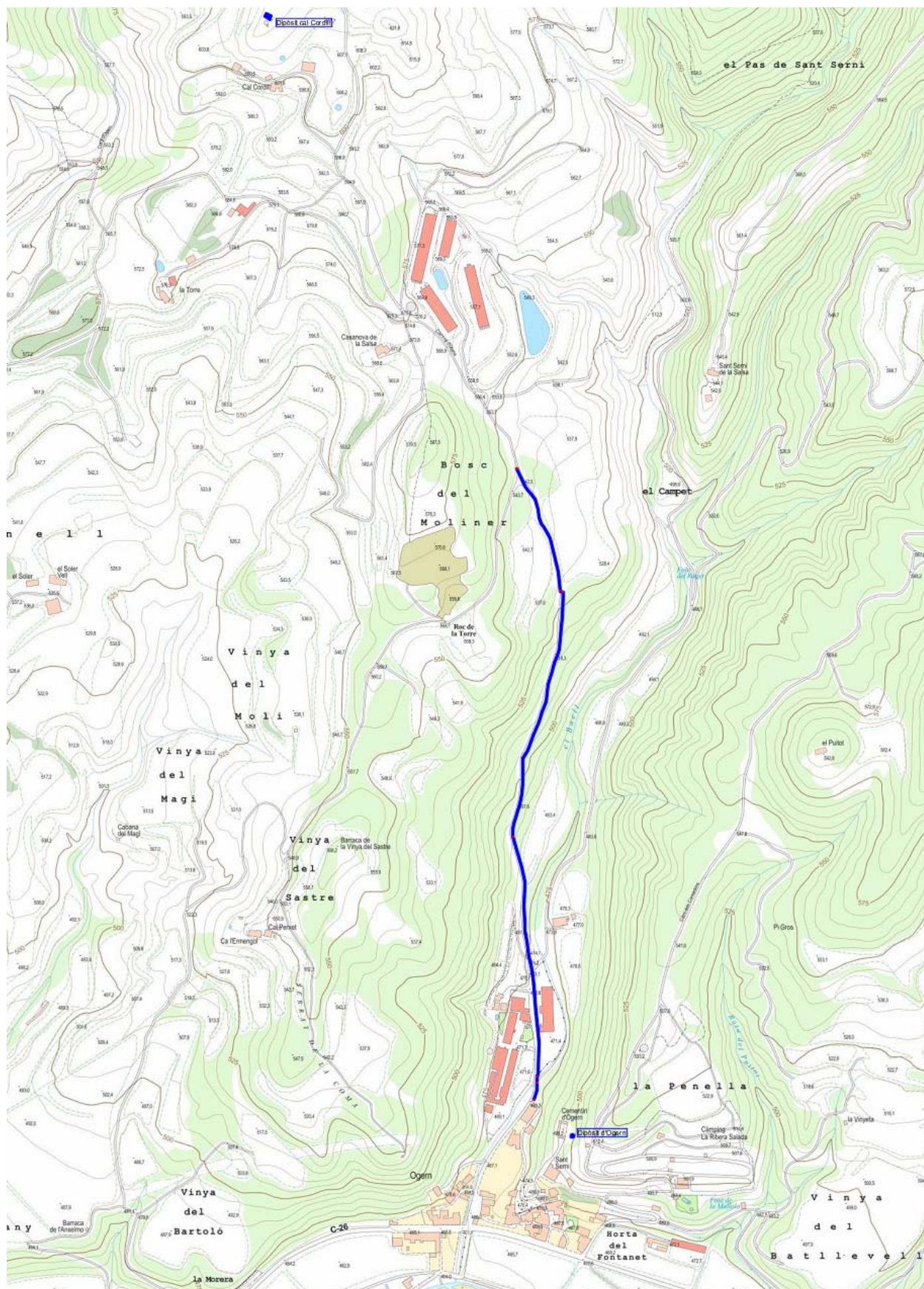
Emplaçament i traçat de la canonada rehabilitada
