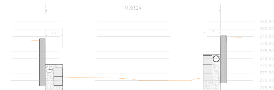
SECCIÓ TRANSVERSAL S3. PROPOSTA
