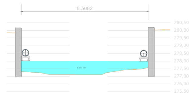
SECCIÓ TRANSVERSAL S2. ESTAT ACTUAL
