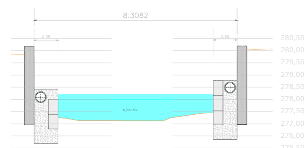
SECCIÓ TRANSVERSAL S2. PROPOSTA
