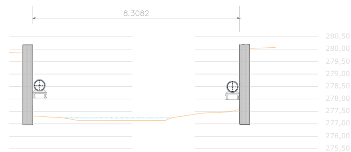
SECCIÓ TRANSVERSAL S2. ESTAT ACTUAL
