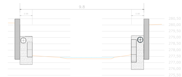
SECCIÓ TRANSVERSAL S1. PROPOSTA
