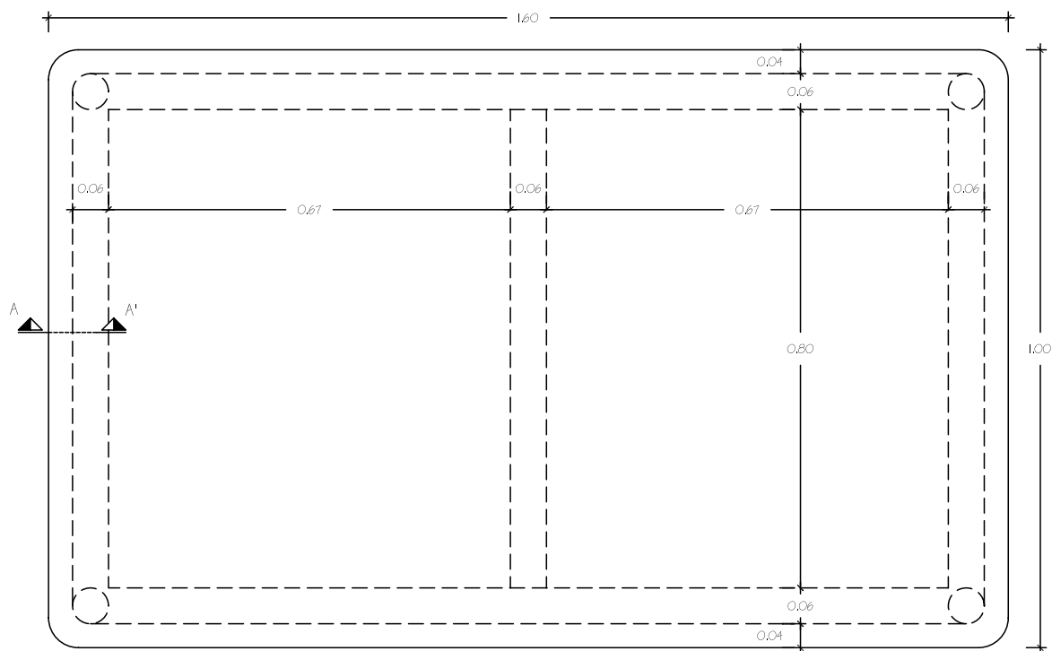
PLANTA
