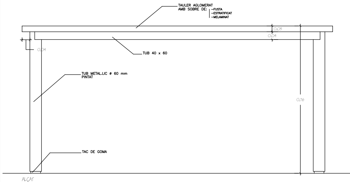
ALÇAT
