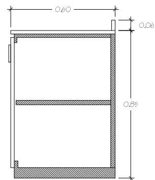
SECCIÓ A-A'
