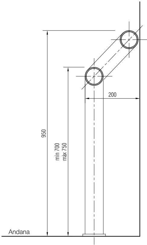
Secc. transversal
