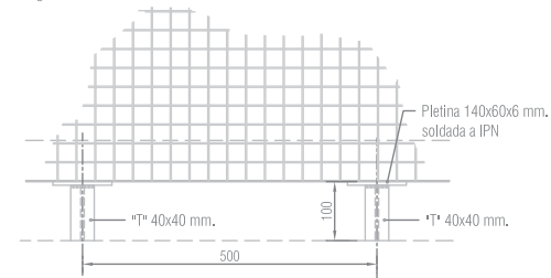
Planta
