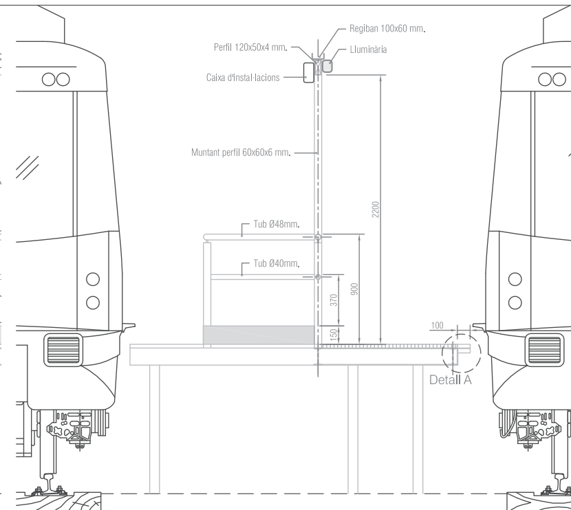
Secció transversal
