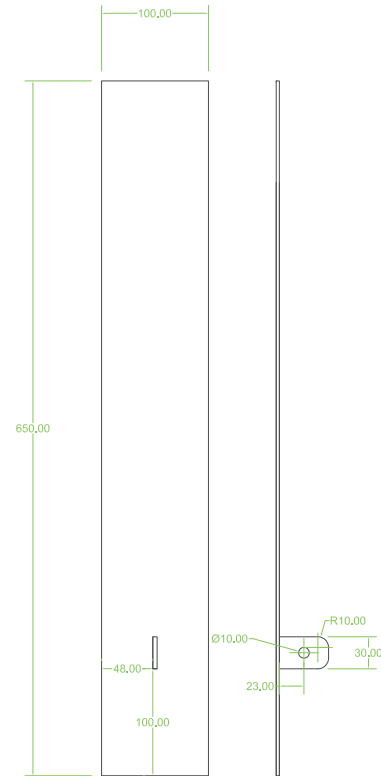
Detall guia cablejat. Cotes en mm.
