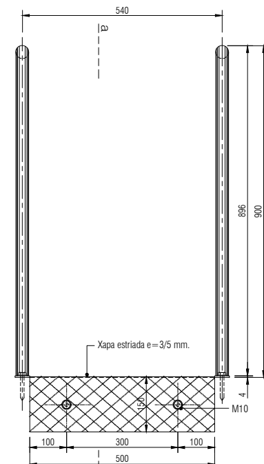
Alçat
