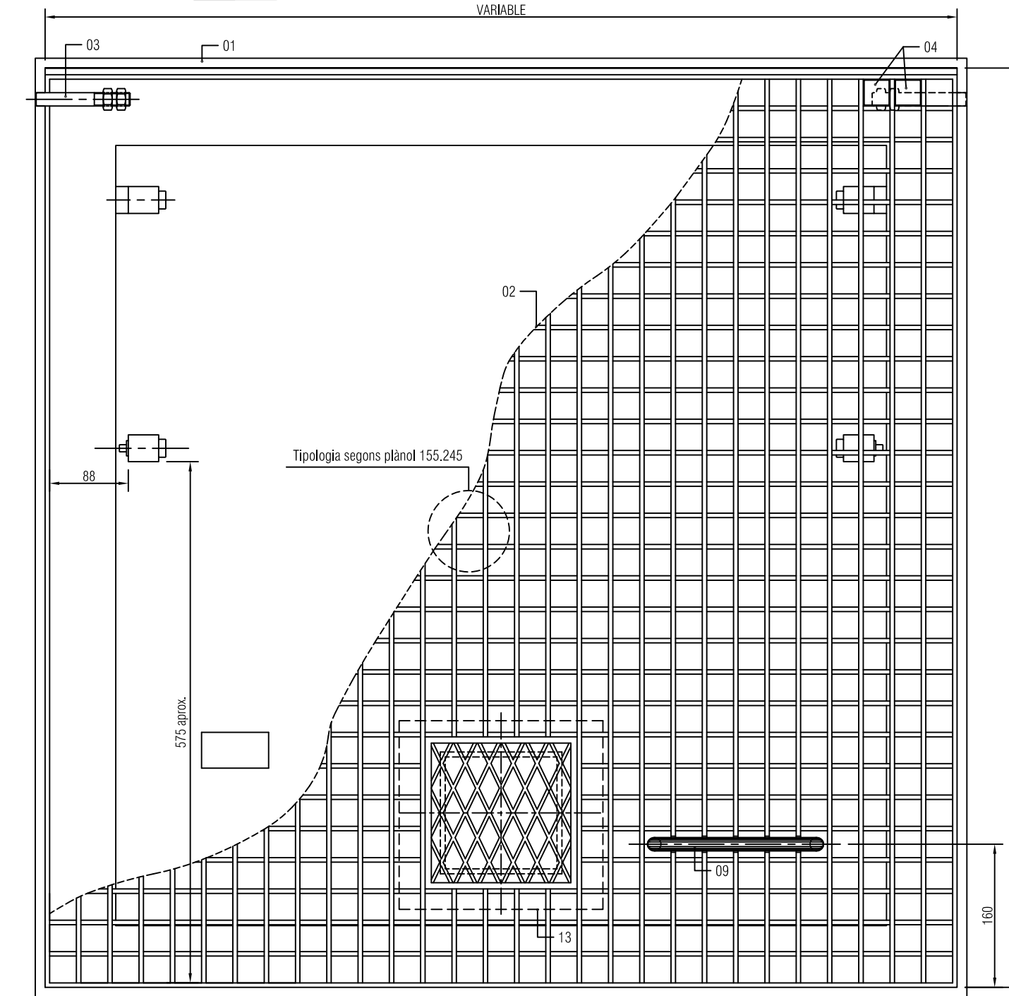
Planta Escala 1:6
