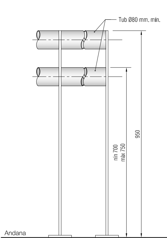
Alçat Recolçament isquiàtic Escala 1:10
