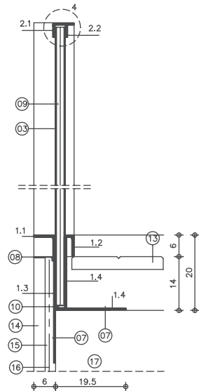
SECCIÓ ESCALA: 1/10. COTES EN cm.
