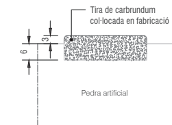
Detall carborundum
