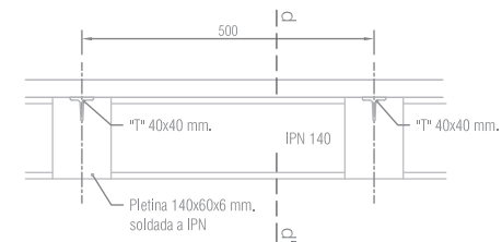
Alçat
