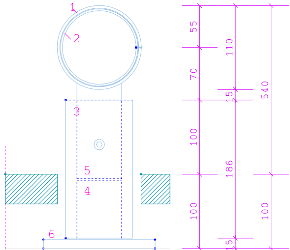
SECCIÓ BARANA
