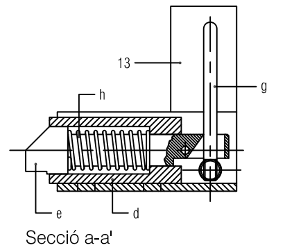
D2. Detall muntatge eix Escala 1:2
