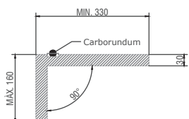
Secció transversal
