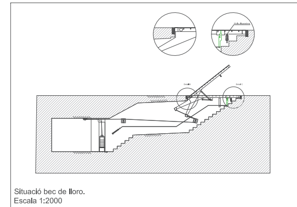
Situació bec de lloro. Escala 1:2000
