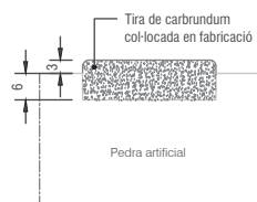
Detall carborundum
