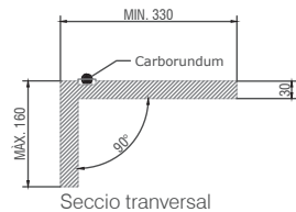
Seccio transversal
