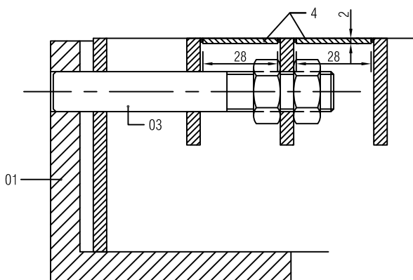
D1. Detall muntatge eix Escala 1:2
