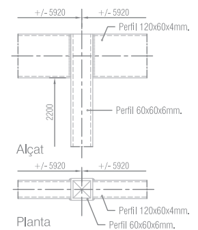
Detall B Escala 1:10 Nota: cotes en mm.
