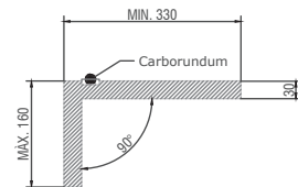
Seccio transversal
