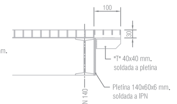
Secció d-d'
