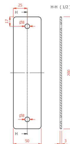
PLETINA BASE UNIÓ PAVIMENT
