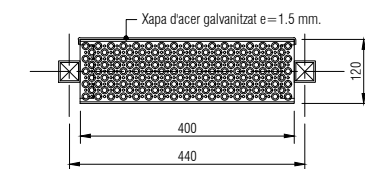
Secció c-c'
