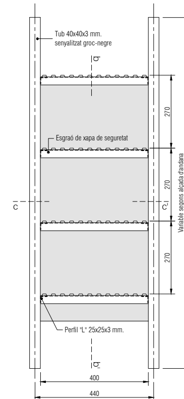
Alçat
