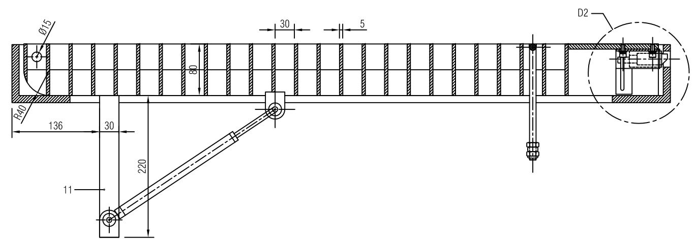
Alçat lateral esquerra Escala 1:6
