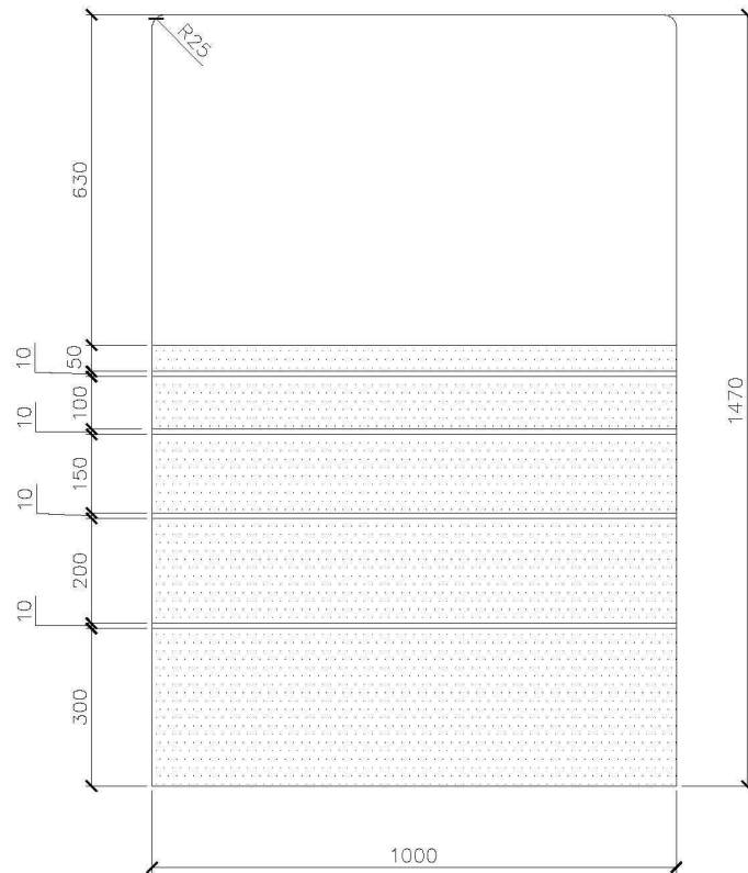
MODULO STANDARD PUERTA 6+6
