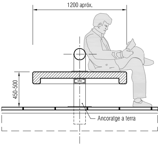
Andana central Escala 1:30
