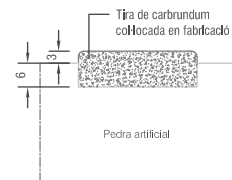
Detall carborundum
