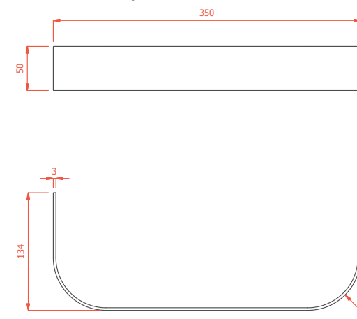
PLETINA DE REFORÇ ESTRUCTURA
