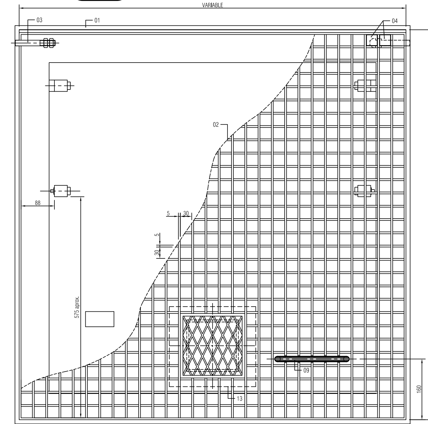
Secció A-A' Escala 1:6
