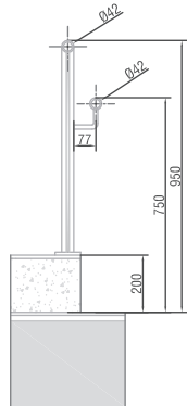
Barana Escala. 1:20
