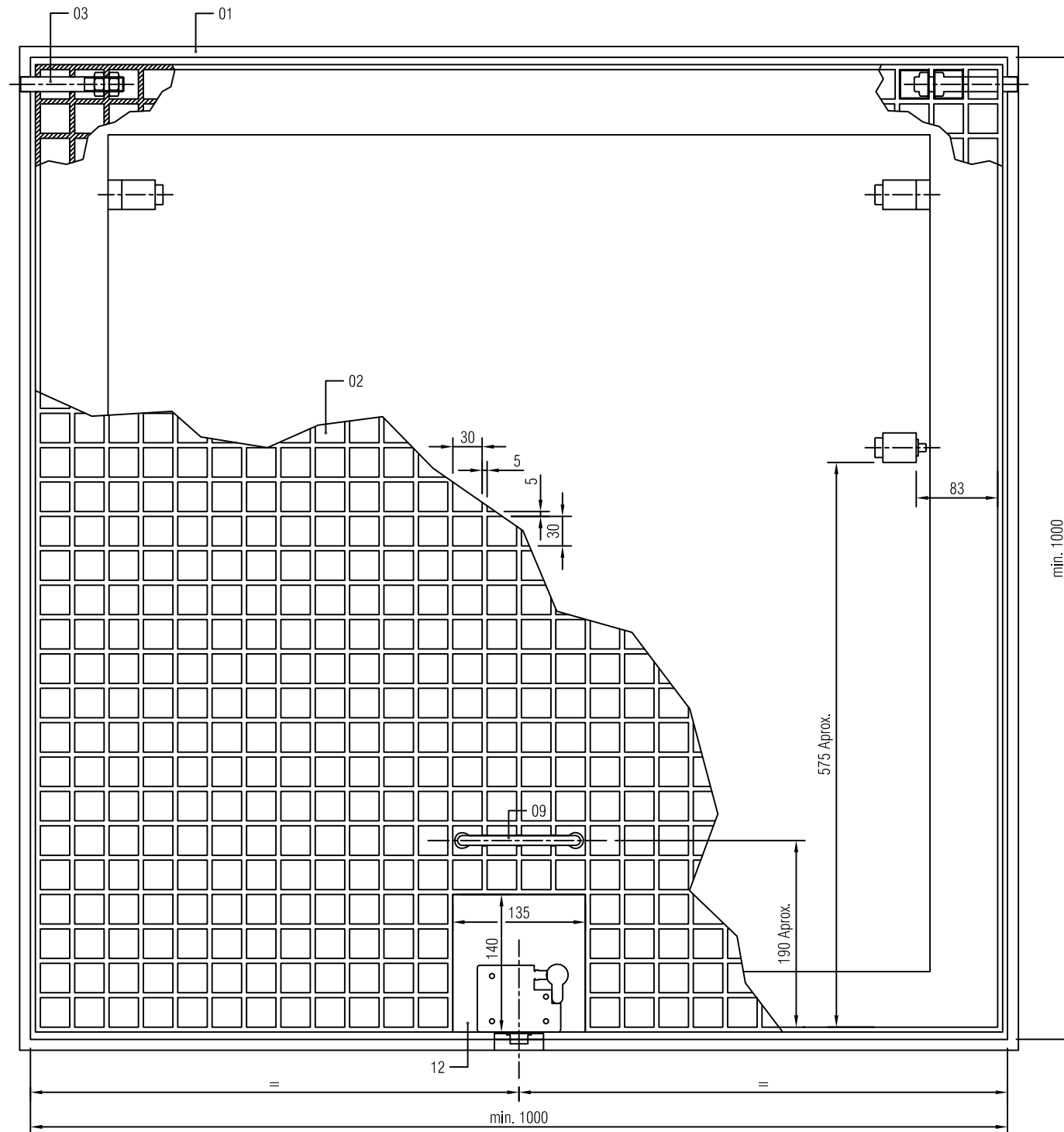
Planta Escala 1:6
