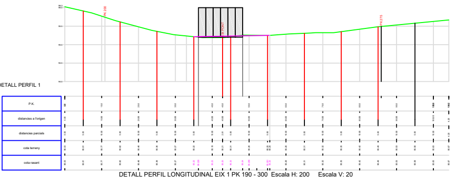
DETALL PERFIL LONGITUDINAL EIX 1 PK 190 - 300 Escala H: 200 Escala V: 20
