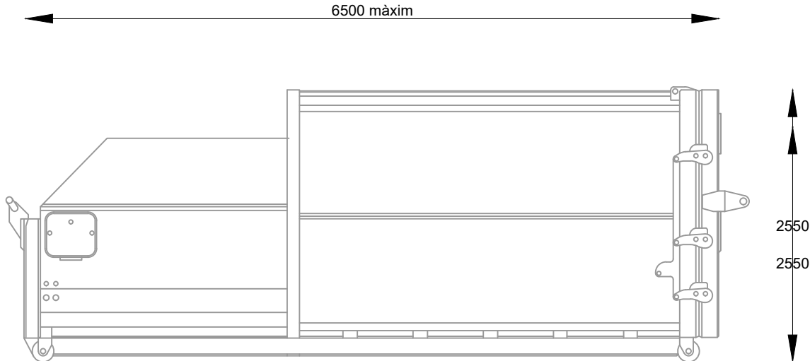
ALÇAT LATERAL
