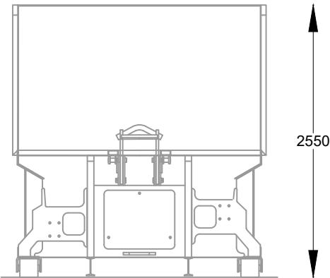
ALÇAT FRONTAL DETALL COMPACTADOR cotes màximes en mm
