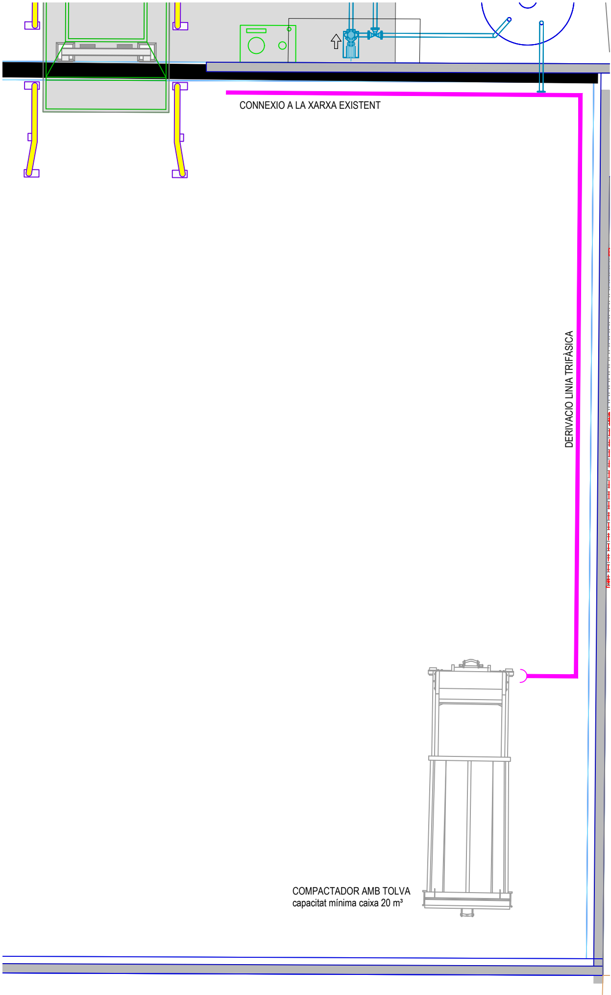
PLANTA EMPLAÇAMENT COMPACTADOR
