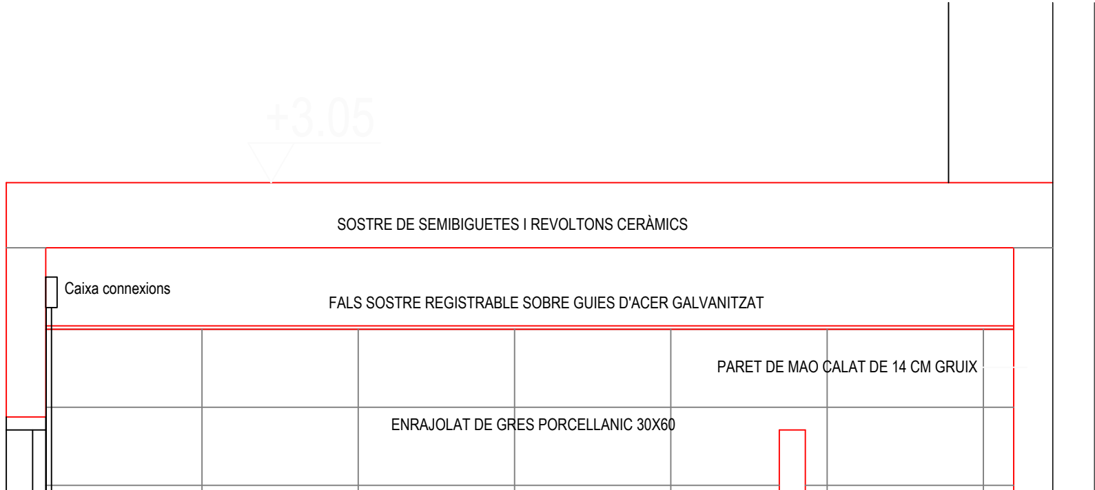
SECCIO A-A
