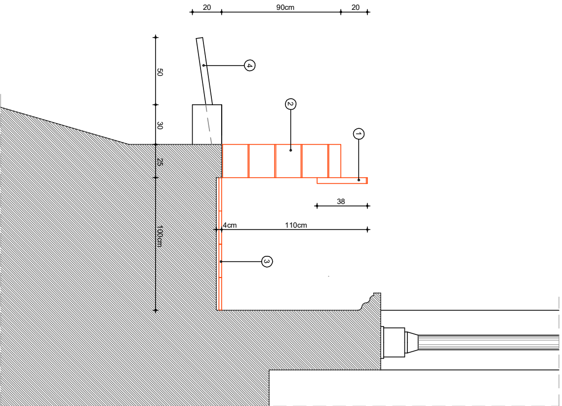
SECCIÓ BARANA CAMÍ DE RONDA E 1:20
