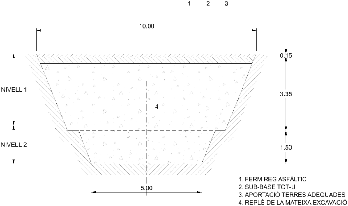
SECCIÓ S-S - REPLÈ
