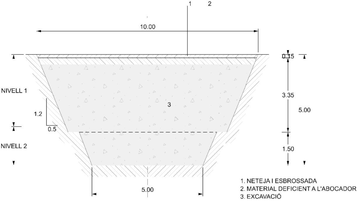
SECCIÓ S-S - EXCAVACIÓ
