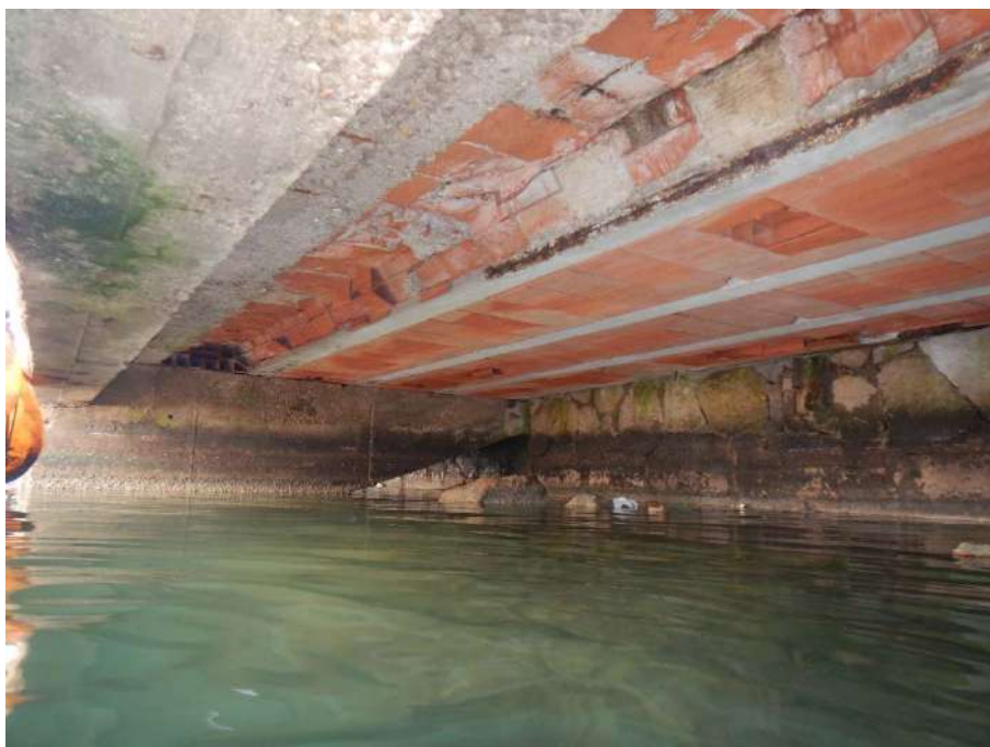
Imatge 3.5. Vista de la part inferior del forjat on s'aprecia la degradació per oxidació de les biguetes.
