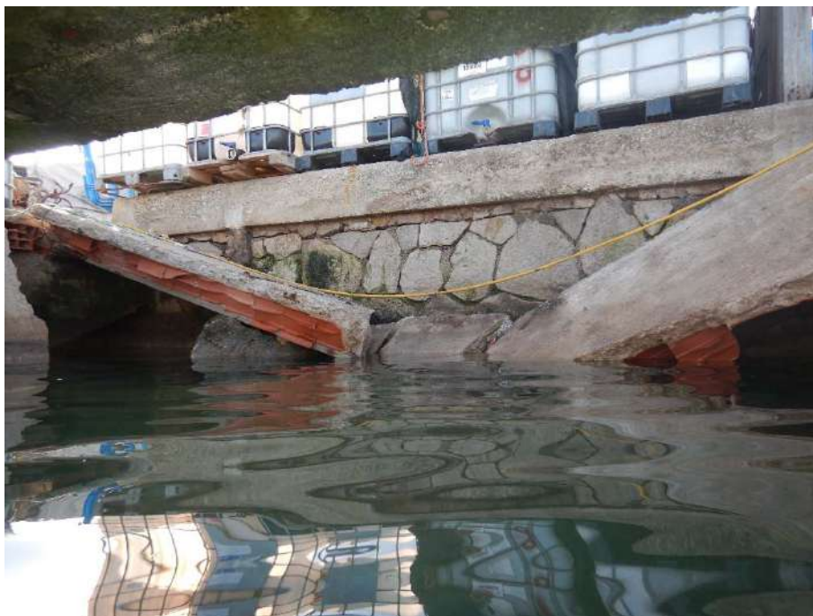
Imatge 3.11. Vista del forjat col·lapsat en data 25.09.2023.
