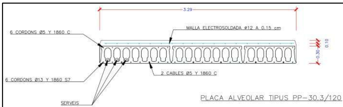
Figura 2.1. Secció de les plaques alveolars a instal·lar
