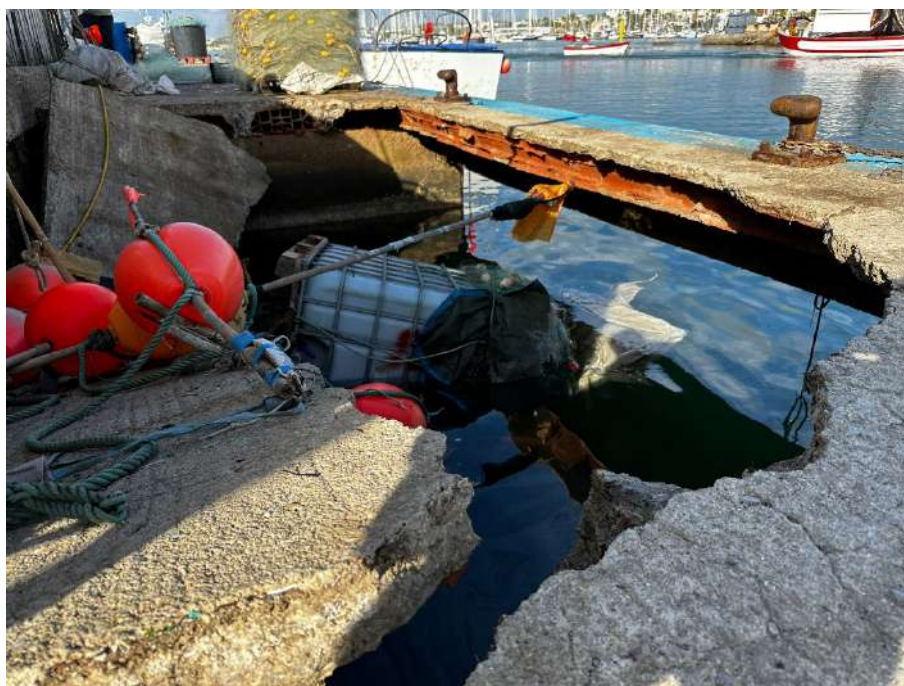
Imatge 3.2. Col·lapse de part del moll claraboia de l'espigó transversal.
