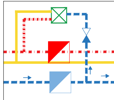
ESQUEMA CONNEXIÓ SERVEIS A TORRETA
