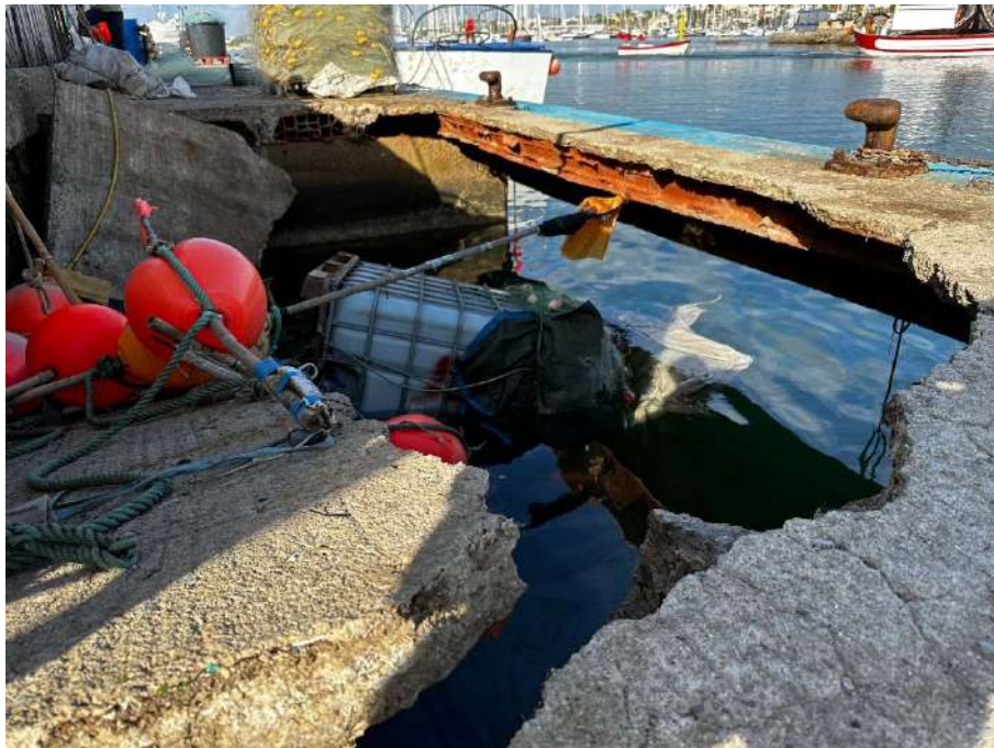
Imatge 1.1. Col·lapse de part del moll claraboia de l'espigó transversal
