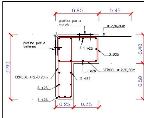
Figura 5.1. Secció tipus biga cantell
