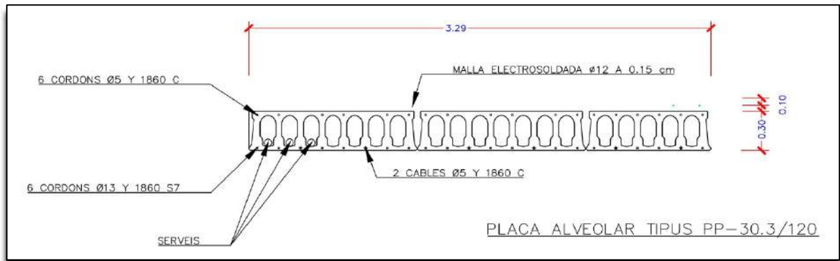
Figura 4.1. Secció de les plaques alveolars a col·locar.
