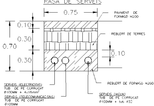
DETALL B – SECCIÓ RASA TIPUS E: 1/25
