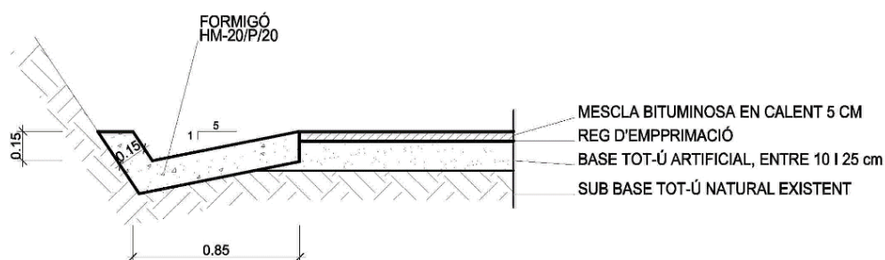
Figura 1. Detall cuneta.
