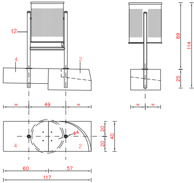
D6 PAPERERA CIRCULAR DE 70l
