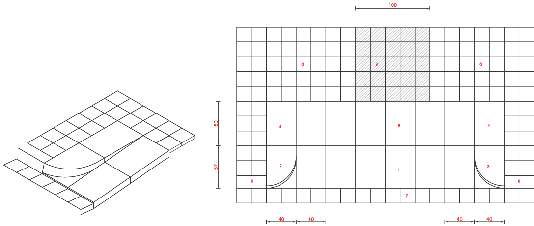
D01 GUAL DE VIANANTS DE FORMIGÓ PREFABRICAT
