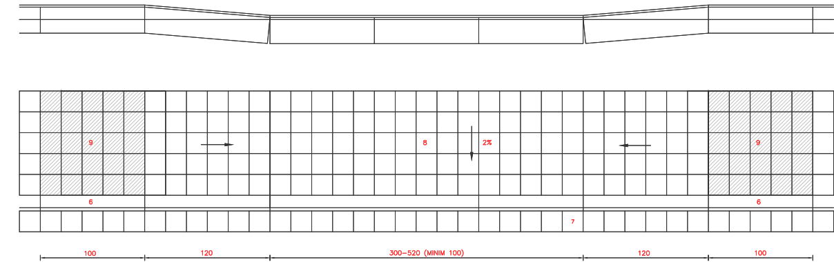
D03 DETALL GUAL DE VIANANTS AMB PENDENTS EN VORERA DE PANOT
