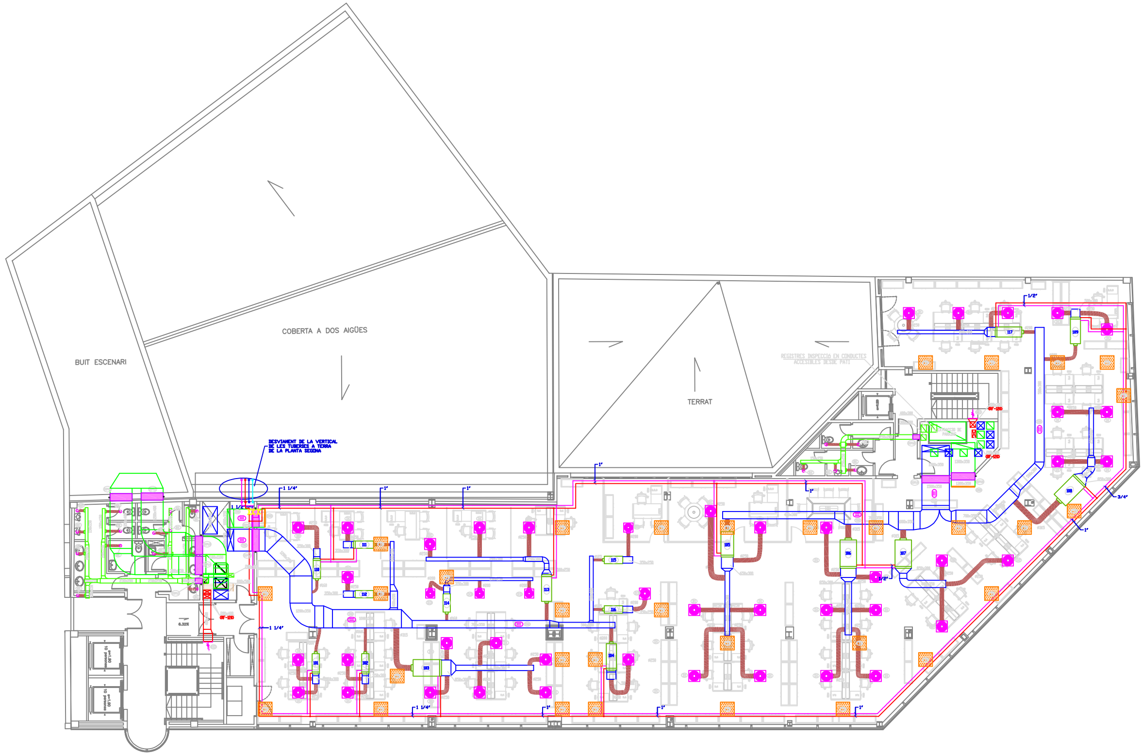
PLANTA 1a
