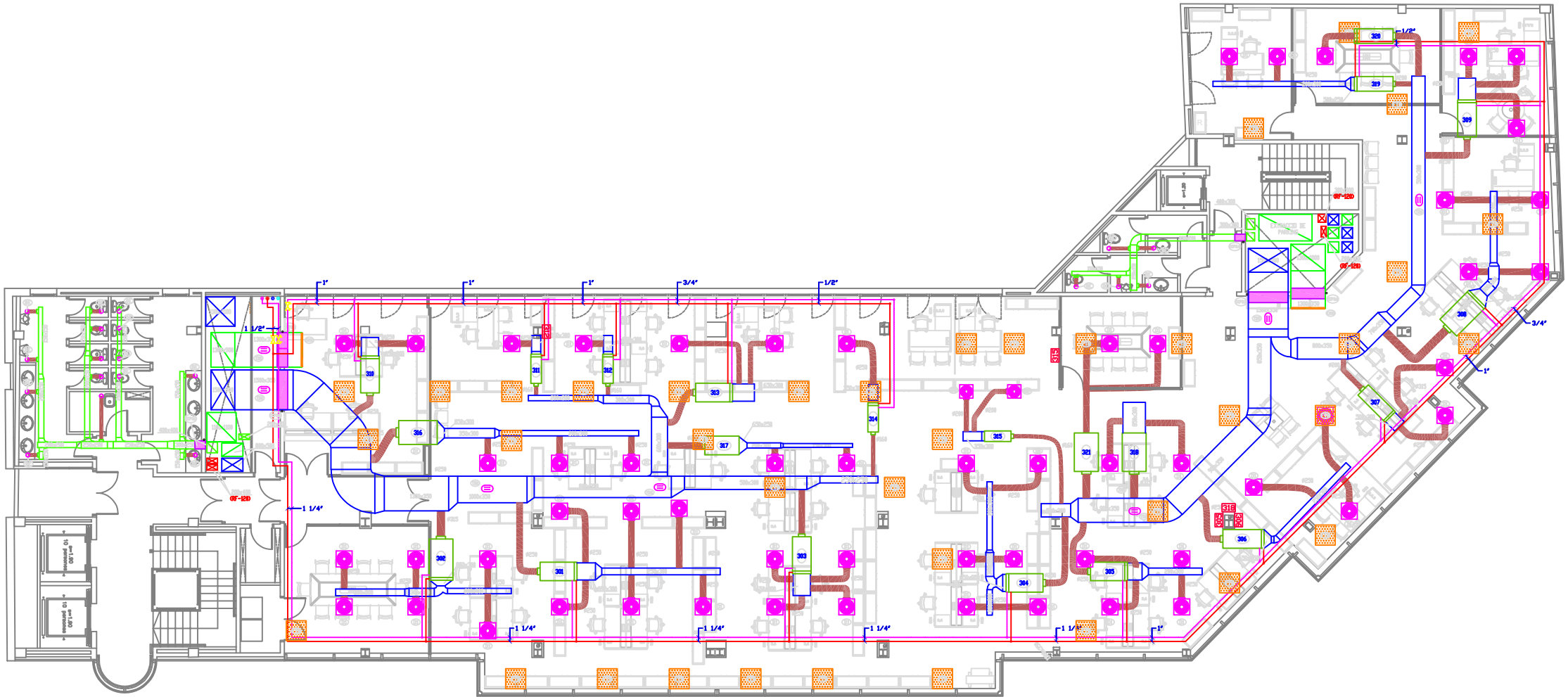
PLANTA 3a
