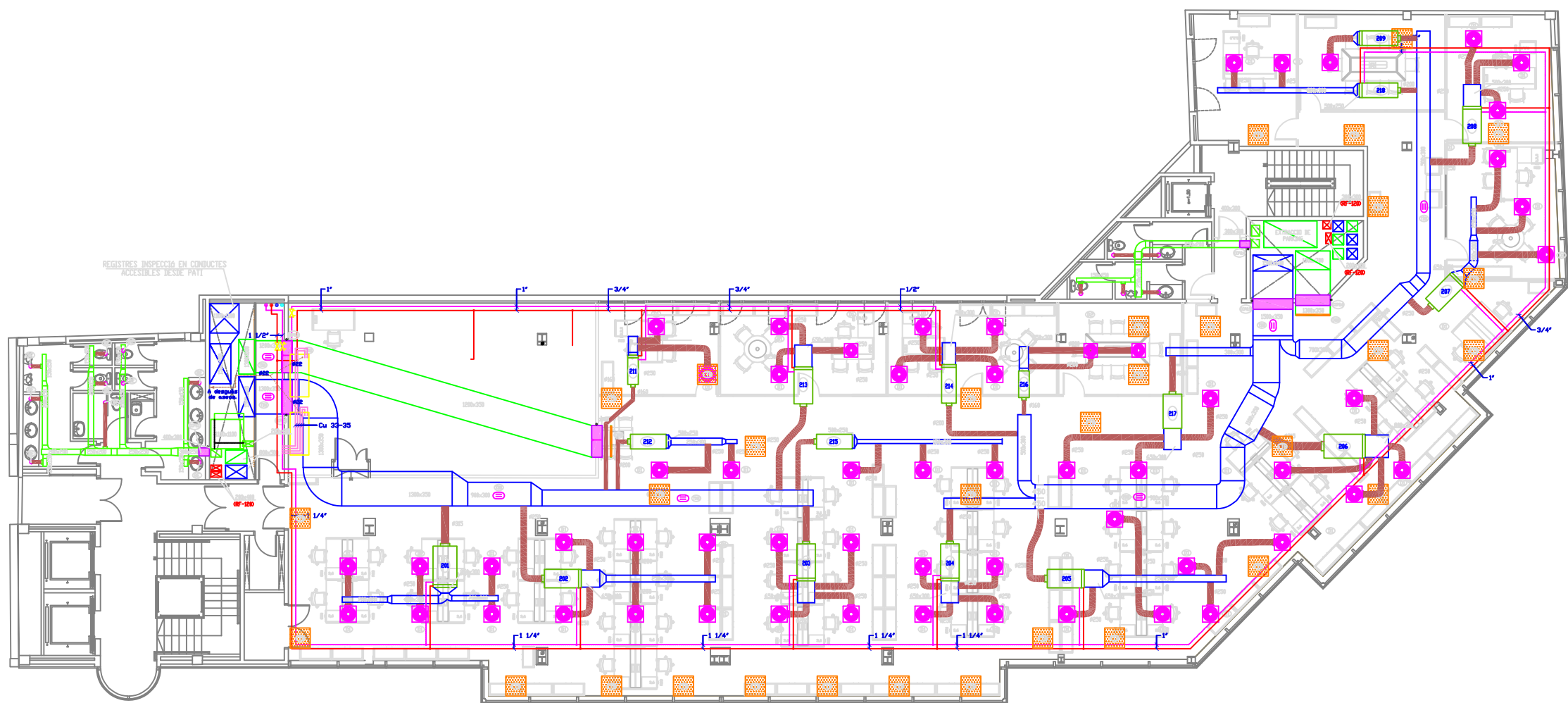
PLANTA 2a
