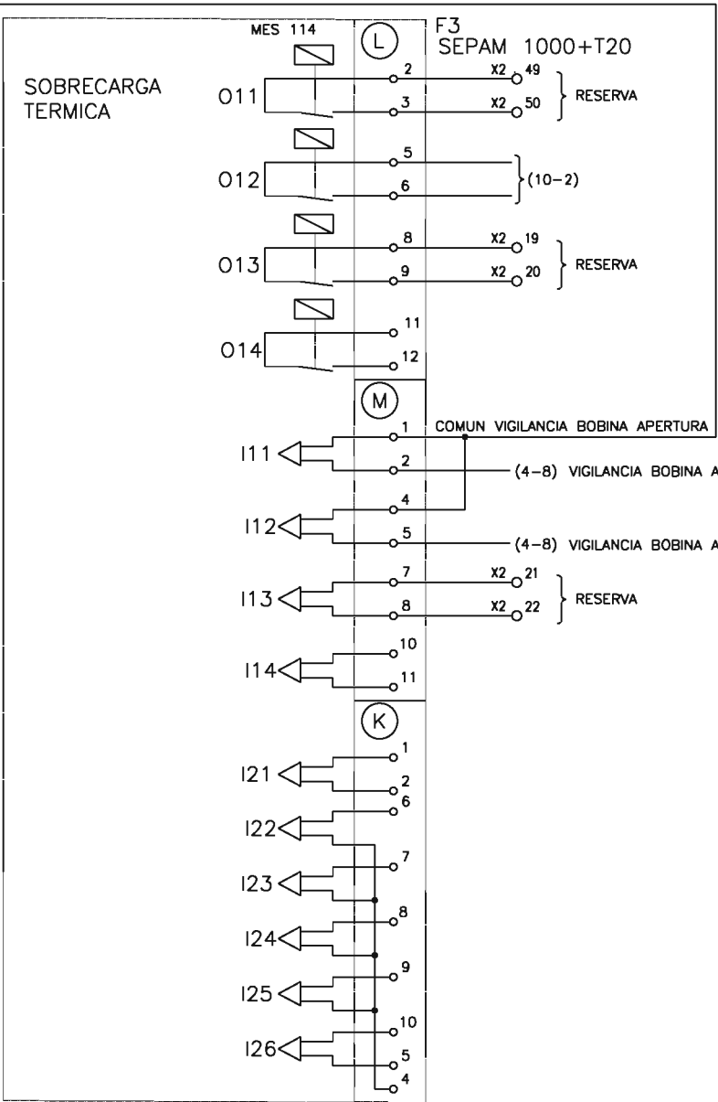
DETALLE CABLEADO DE CONTROL DEL RELE DE PROTECCION
