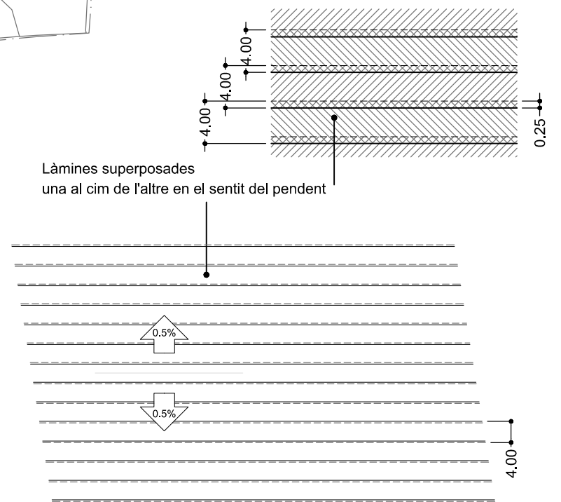
DETALL COL.LOCACIÓ LÀMINES DE PLÀSTIC
