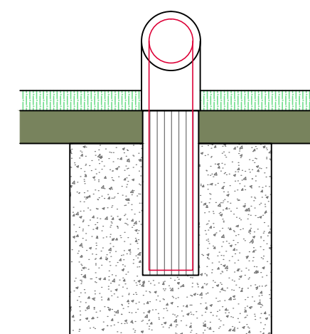
DETALL ANCORATGES TUB D'ACER GALVANITZAT
