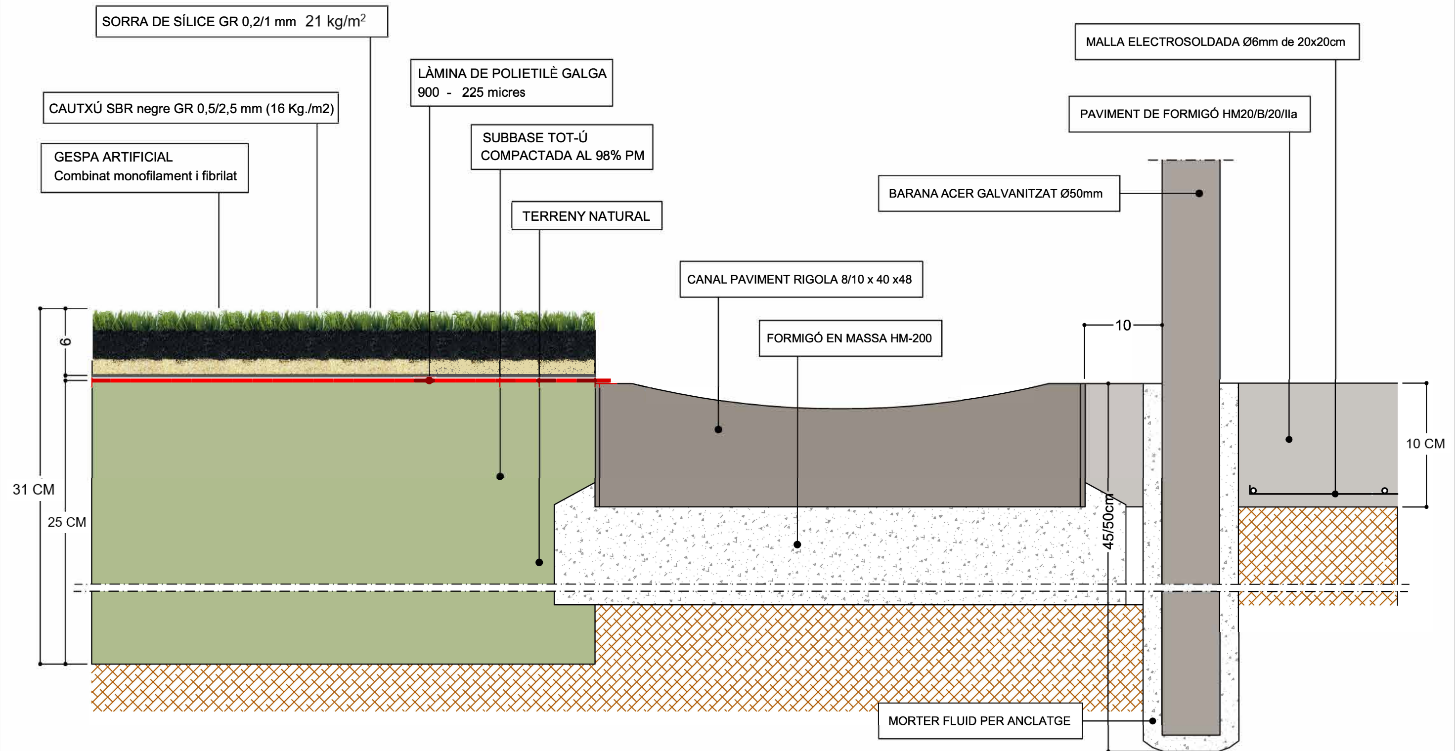
PERFIL CONSTRUCTIU GESPA ARTIFICIAL I FRANJA DE FOMIGÓ
