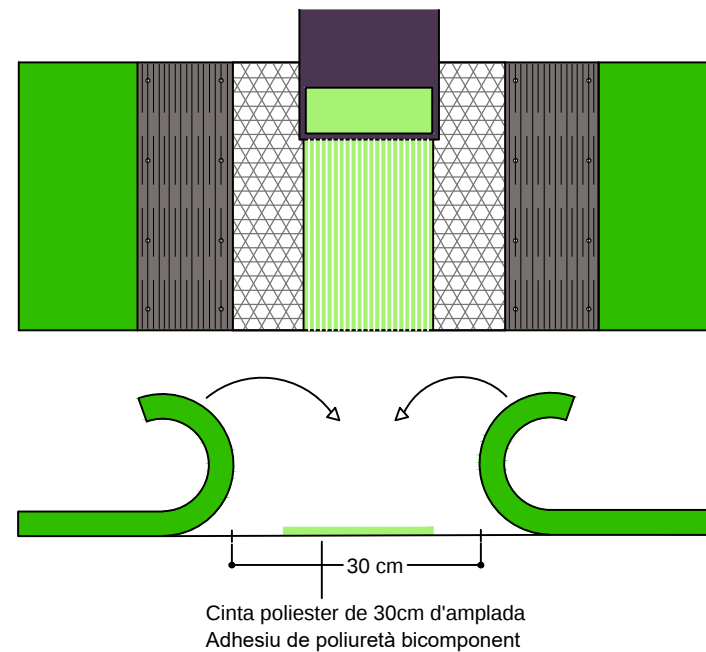
DETALL ENCOLAT JUNTES
