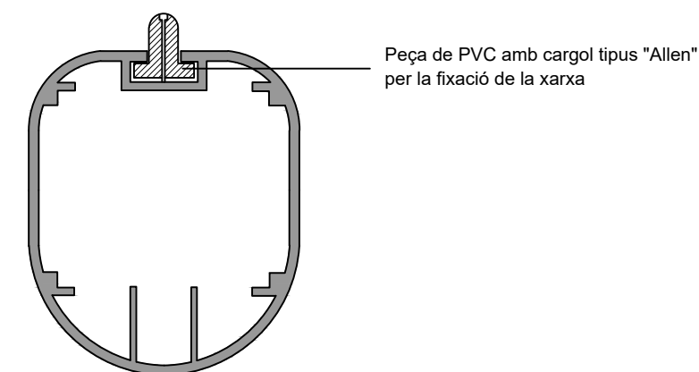
DETALL PERFIL D'ALUMINI DE PALS I TRAVESSER
