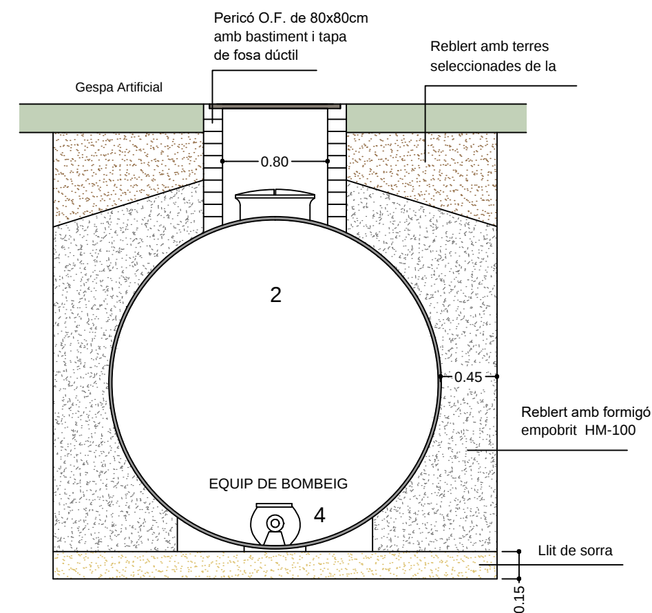
SECCIÓ TRANSVERSAL
