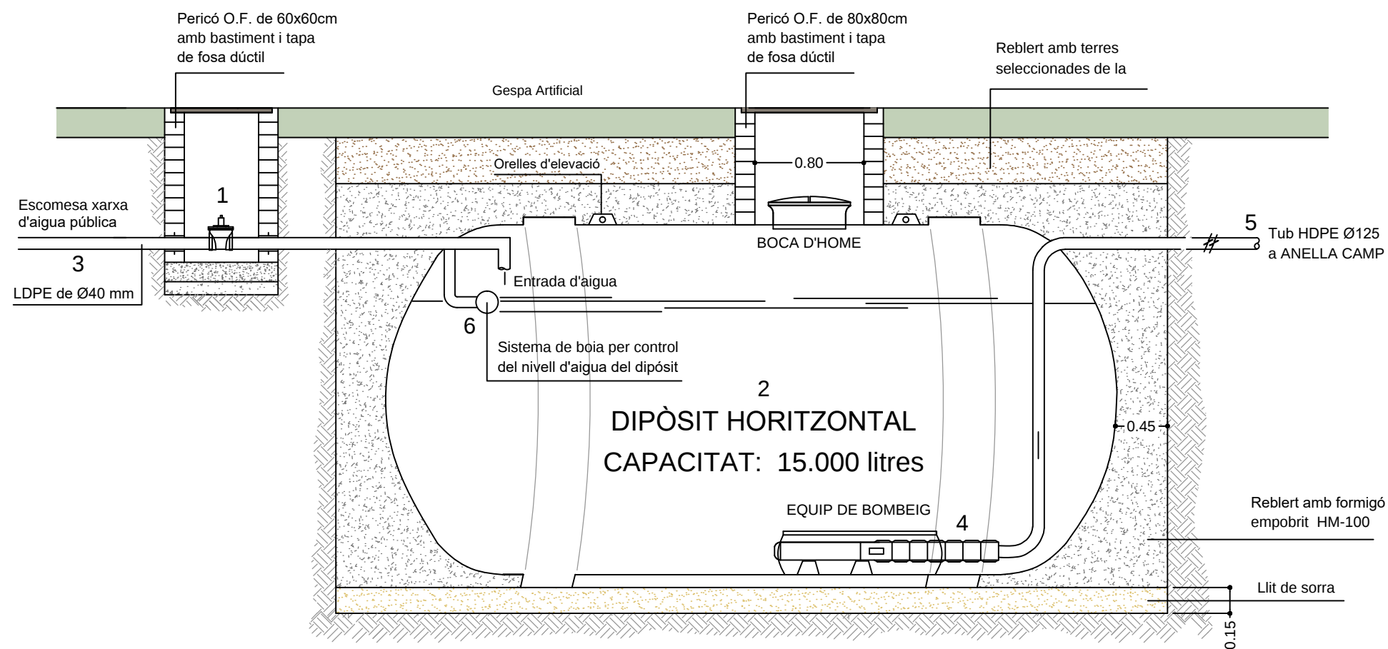
SECCIÓ LONGITUDINAL
