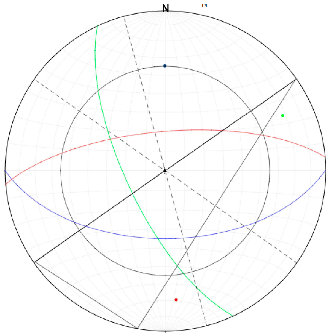
Projecció estereogràfica dels plans de diàclasis.
