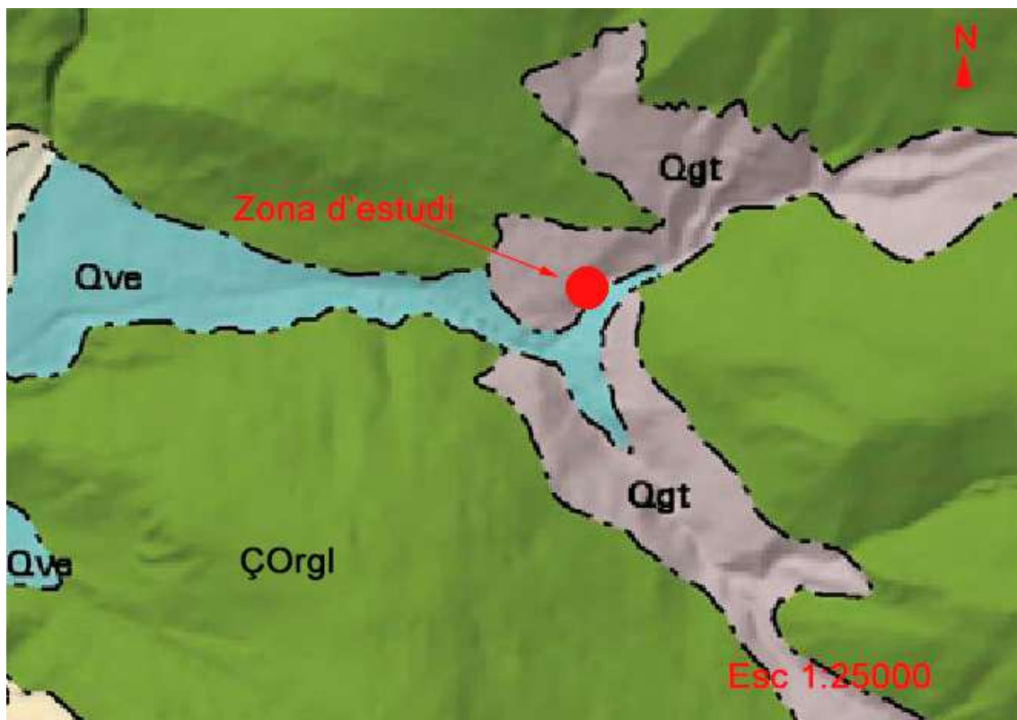
Situació geològica.
