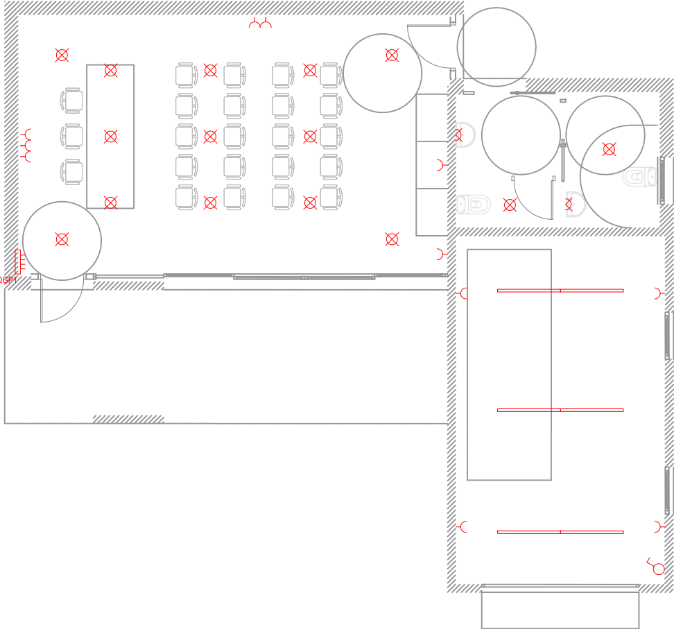
Instal·lació elèctrica
