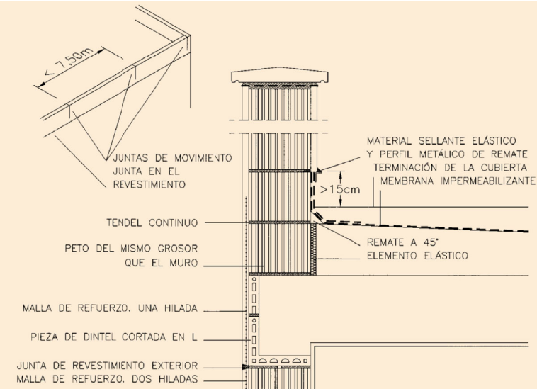
Detalls constructius tancament estructural de bloc ceràmic alleugerit
