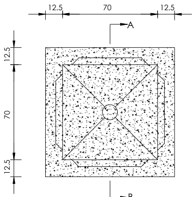
PLANTA
