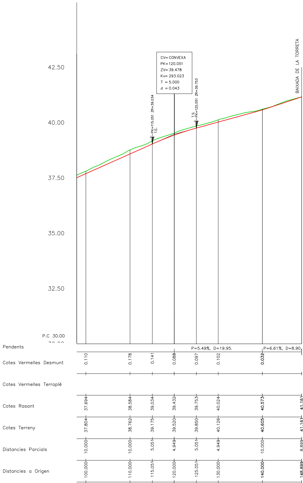
PERFIL LONGITUDINAL EIX CARRER DE DALT TRAM PK 0+100.00 A PK 0+148.889
