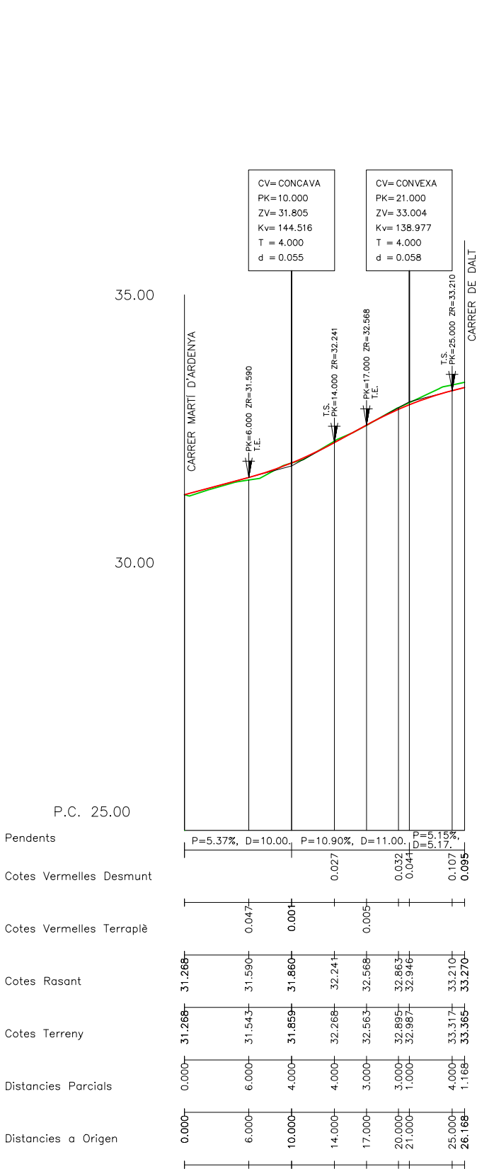
PERFIL LONGITUDINAL EIX CARRER DE L'HOSTAL
