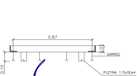
SECCIÓ A-A'
