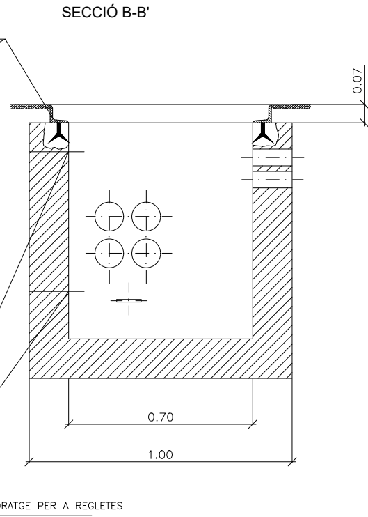
SECCIÓ B-B'
