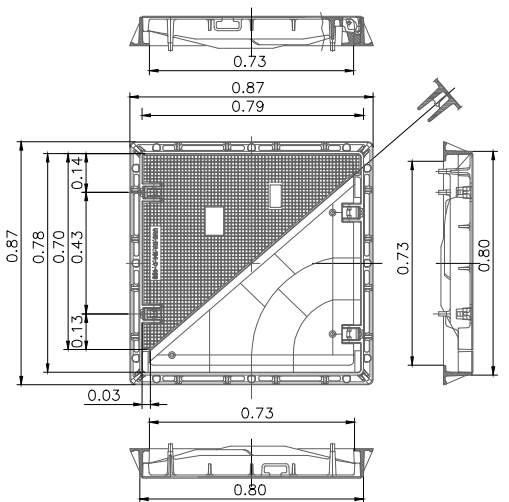
TAPA QUADRADA
