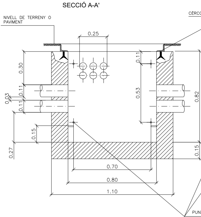
SECCIÓ A-A'
