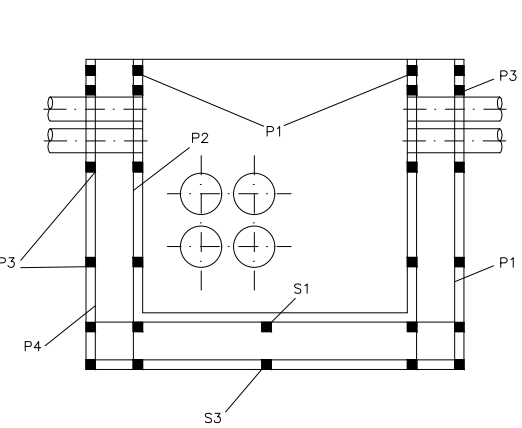
SECCIÓ B-B'
