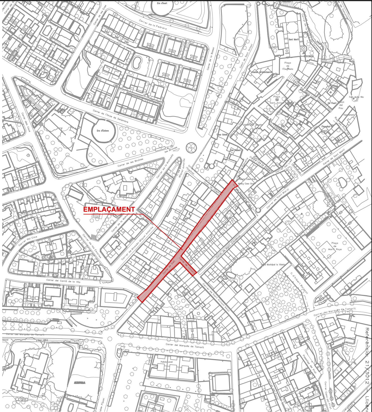
EMPLAÇAMENT ESCALA: 1/2.000
