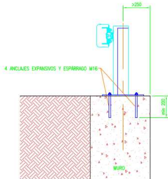
PROCEDIMIENTO EN CORONACIÓN DE MUROS O SOBRE OBRAS DE FÁBRICA (OPCIÓN B)
