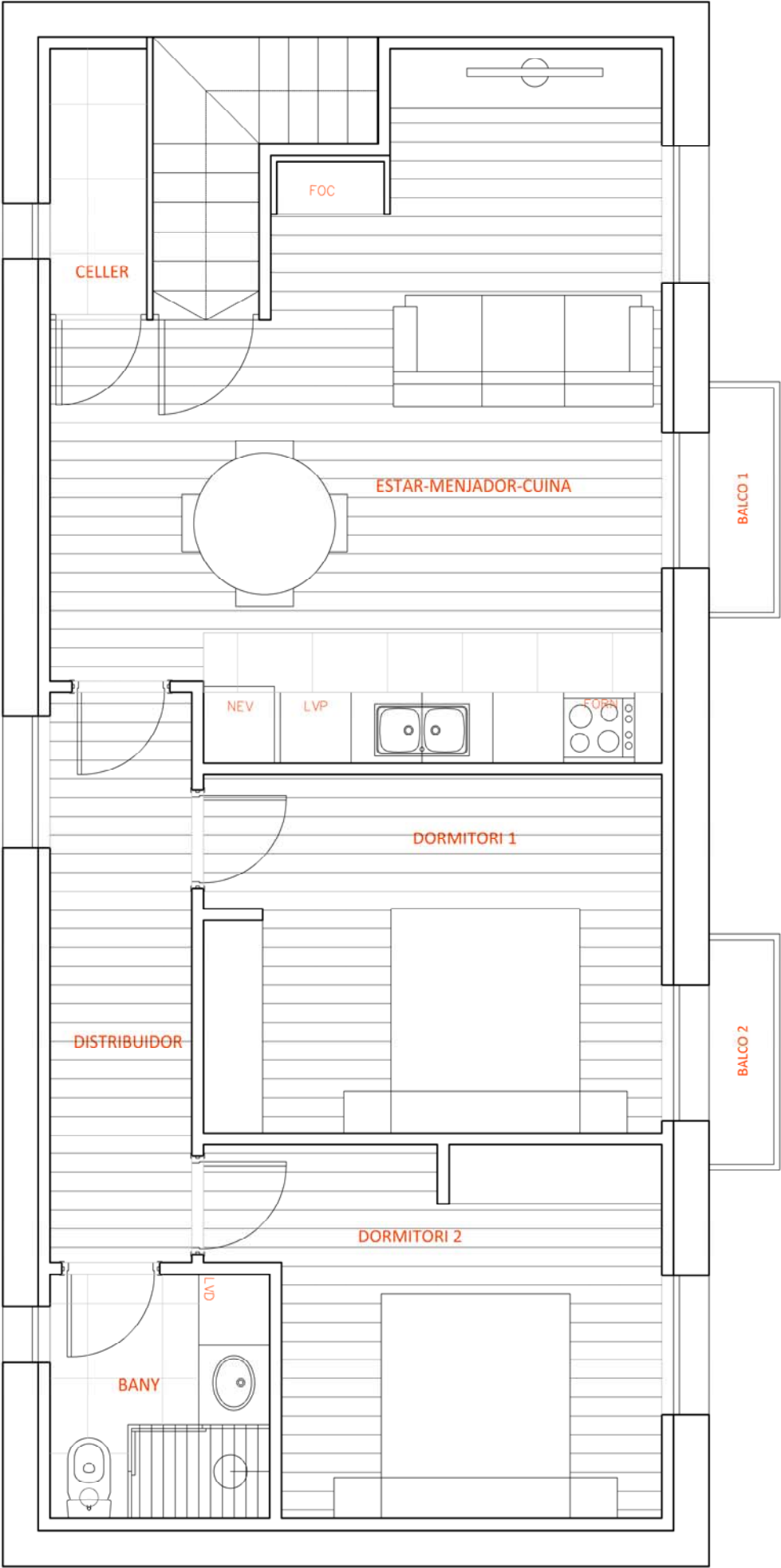
ESTAT MODIFICAT
