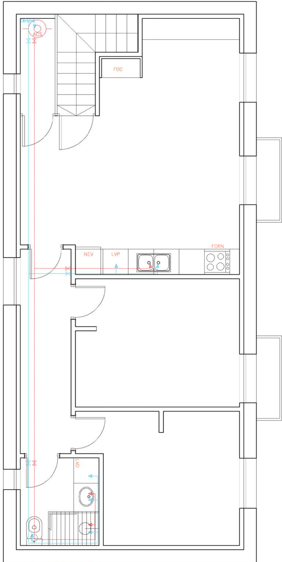
PLANOL FONTANERIA
