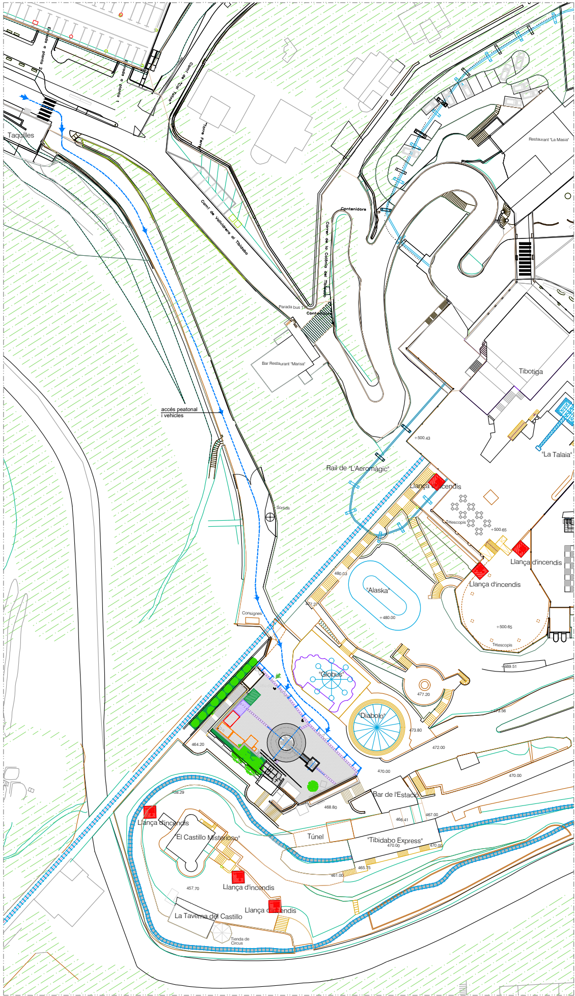
Situació i accessos a obra E 1:500
