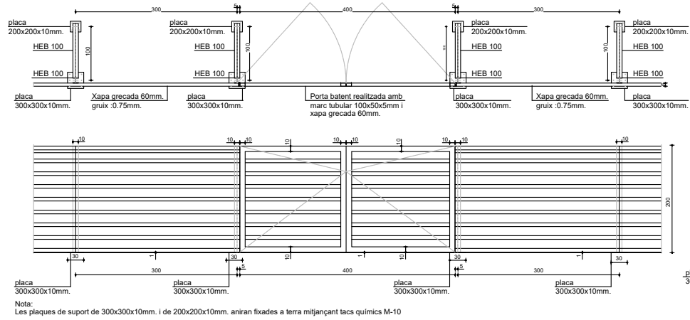
Planta i alçat tancament provisional d'obra E 1:50
