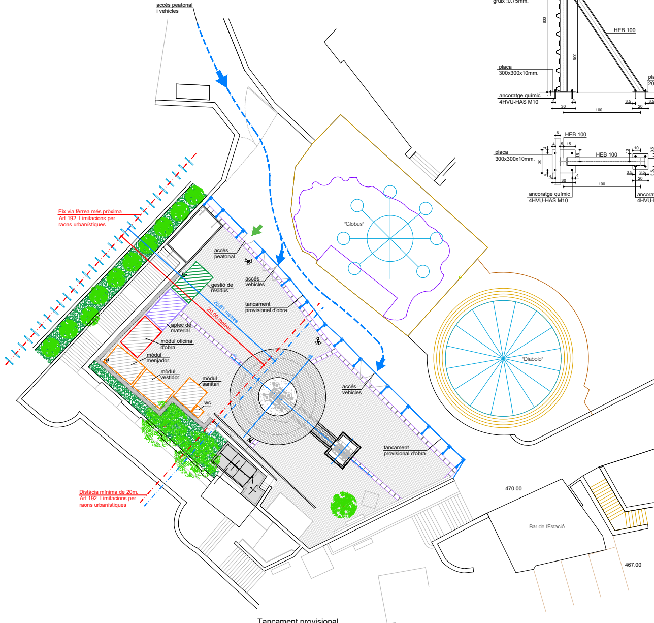
Tancament provisional Replanteig afectacions a obra E 1:200
