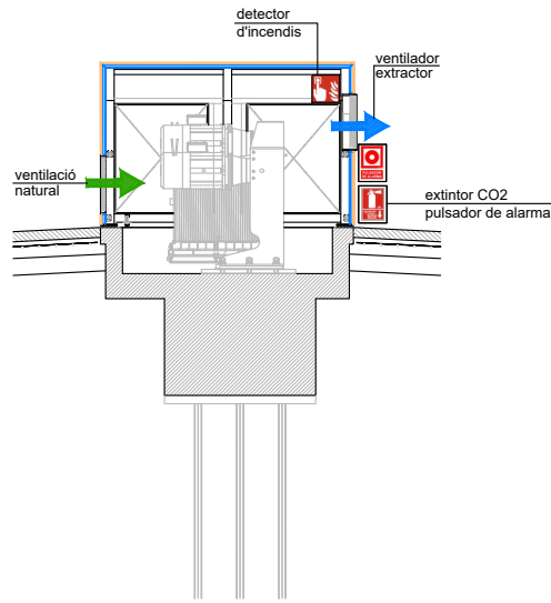
Secció transversal tancament winch E.1.50
