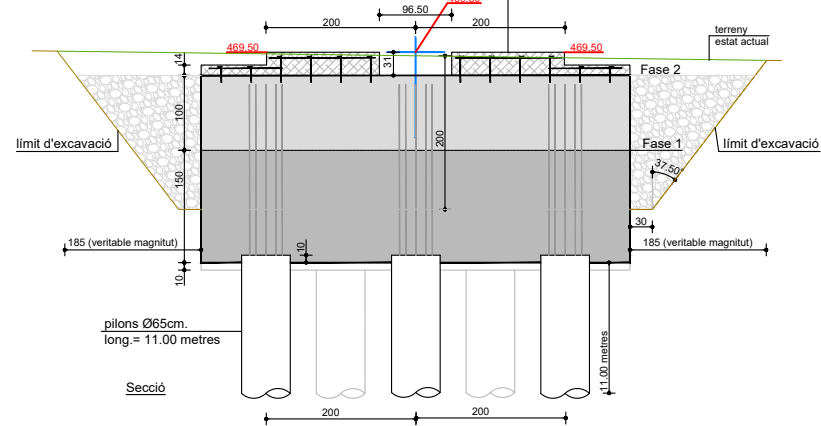
Definició geomètrica encep i límits d'excavació E.1.50
