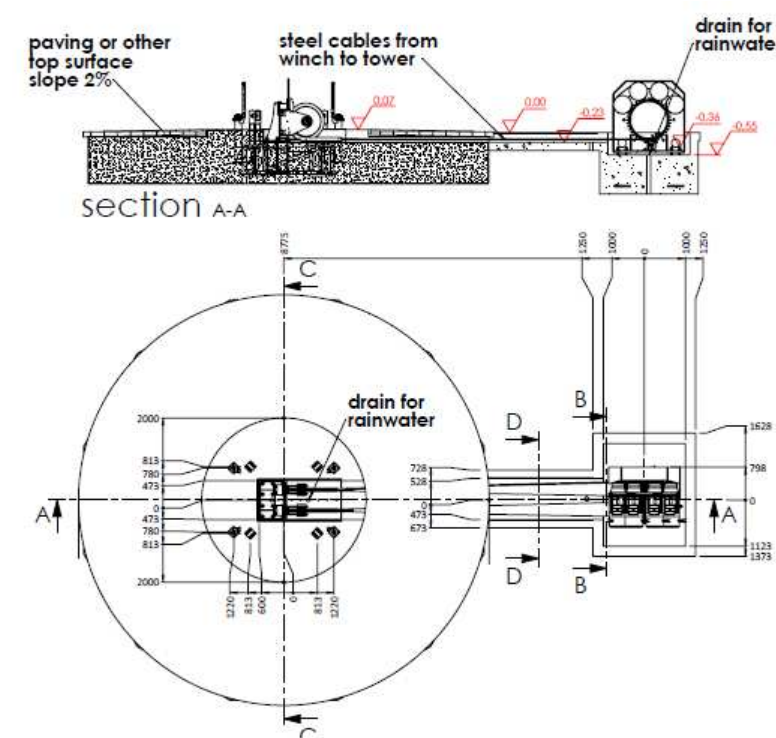
Imatge. Vista general conceptual de la instal·lació de l'atracció.
