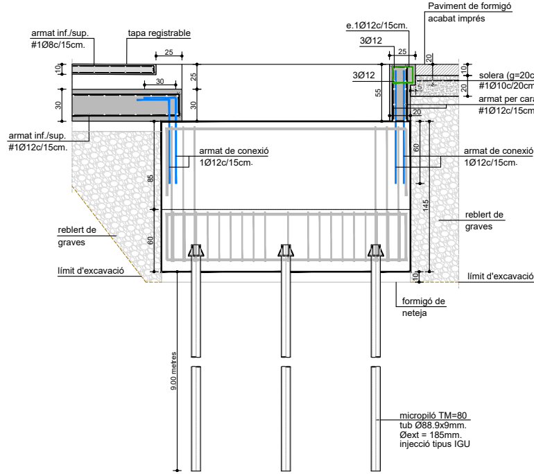
Detall 1. Secció X E 1.25
