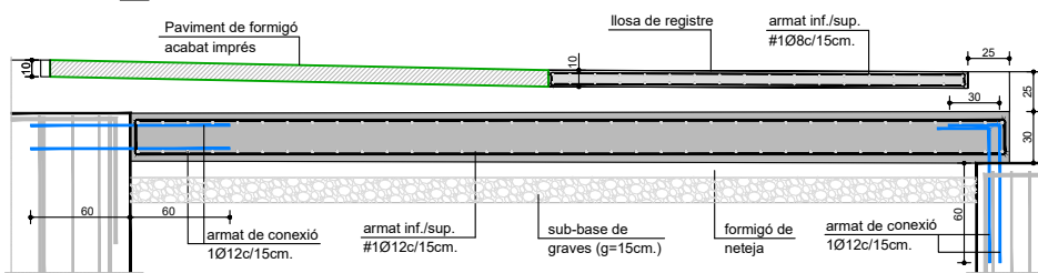
Detall 2. Secció V E 1.25
