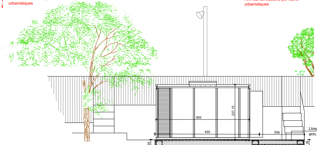
Secció longitudinal llosa fonaments caseta annexa E 1:50
