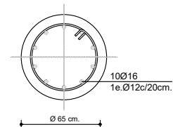
Secció pilons Ø 65cm. E.1.20
