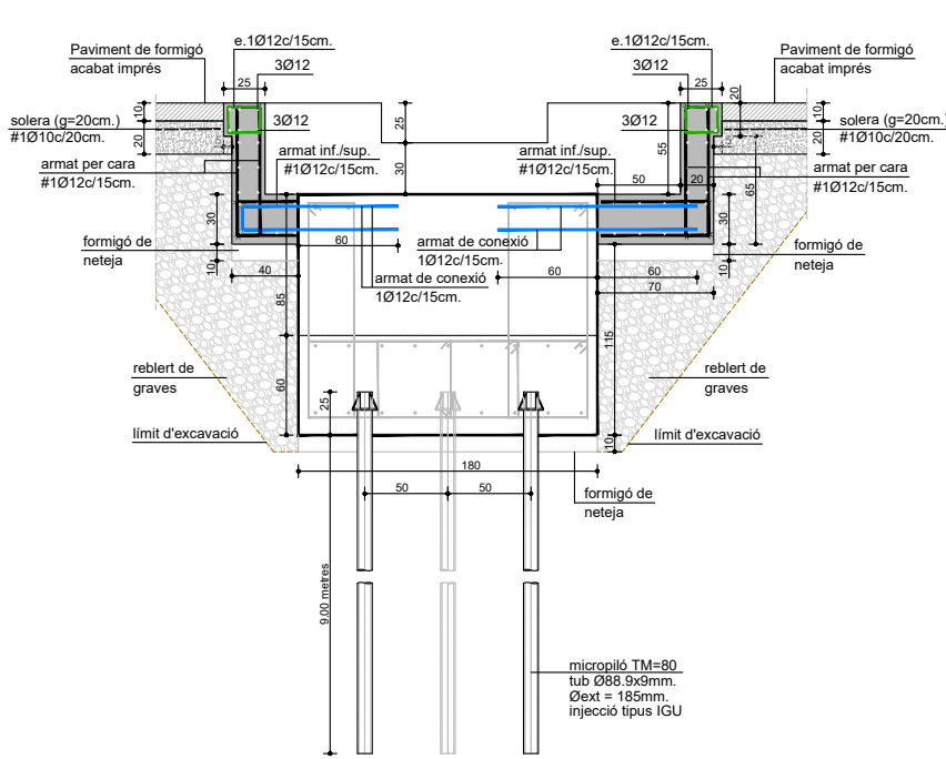
Detall 1. Secció Y E 1.25
