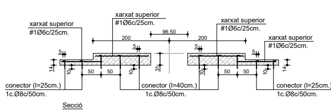
Definició geomètrica i d'armat de recobriments superior de formigó amb acabat imprès E.1.50
