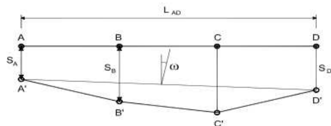
Definiciones básicas del movimiento de cimentaciones
