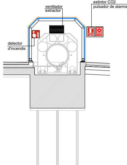
Secció longitudinal tancament winch E.1.50
