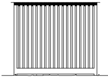
ALÇAT LATERAL DRETA
