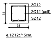
Secció Z2 E 1:20
