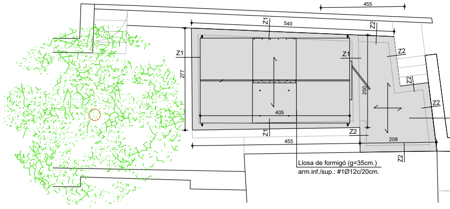
Replanteig llosa fonaments caseta annexa E 1:50
