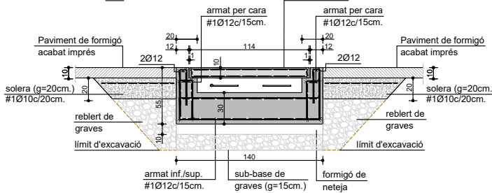
Detall 2. Secció Z E 1.25
