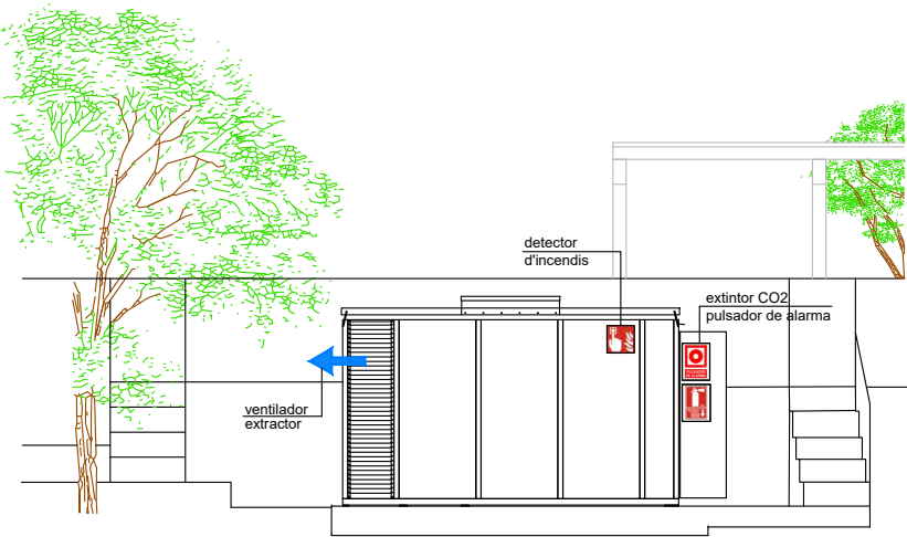
Alçat caseta annexa E.1.56
