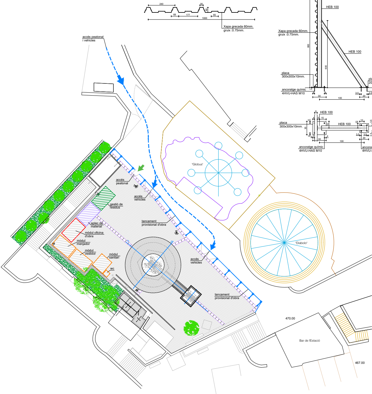
Tancament provisional Replanteig afectacions a obra E 1:200
