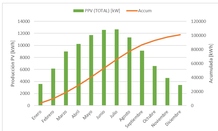
Figura 9. Producción mensual y anual de electricidad para la situación óptima y la integración real.
