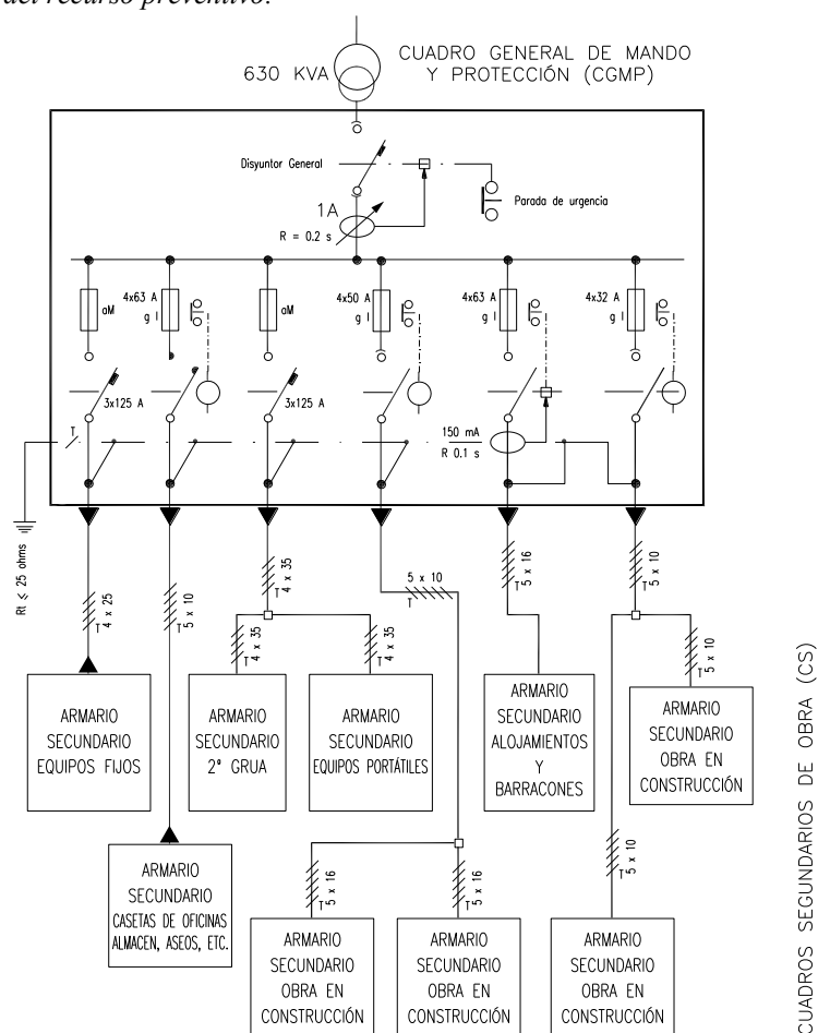
Figura 10. Esquema del recurso preventivo.
