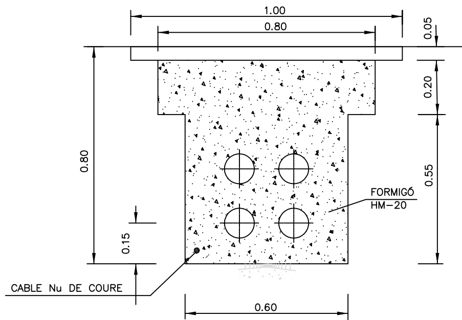
RASA CREUAMENT CALÇADA 4Ø110 P.E. CORRUGAT
