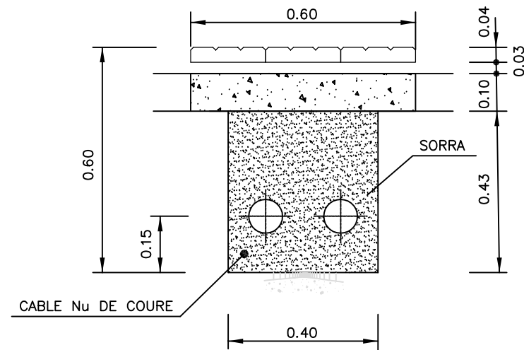
RASA SOTA VORERA 2Ø 90 P.E. CORRUGAT
