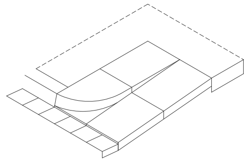
D02 GUAL DE VIANANTS DE FORMIGÓ PREFABRICAT
