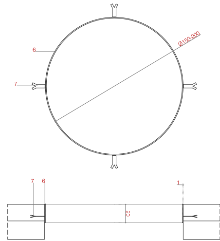
D03 ESCOCELL CIRCULAR D'ACER GALVANITZAT
