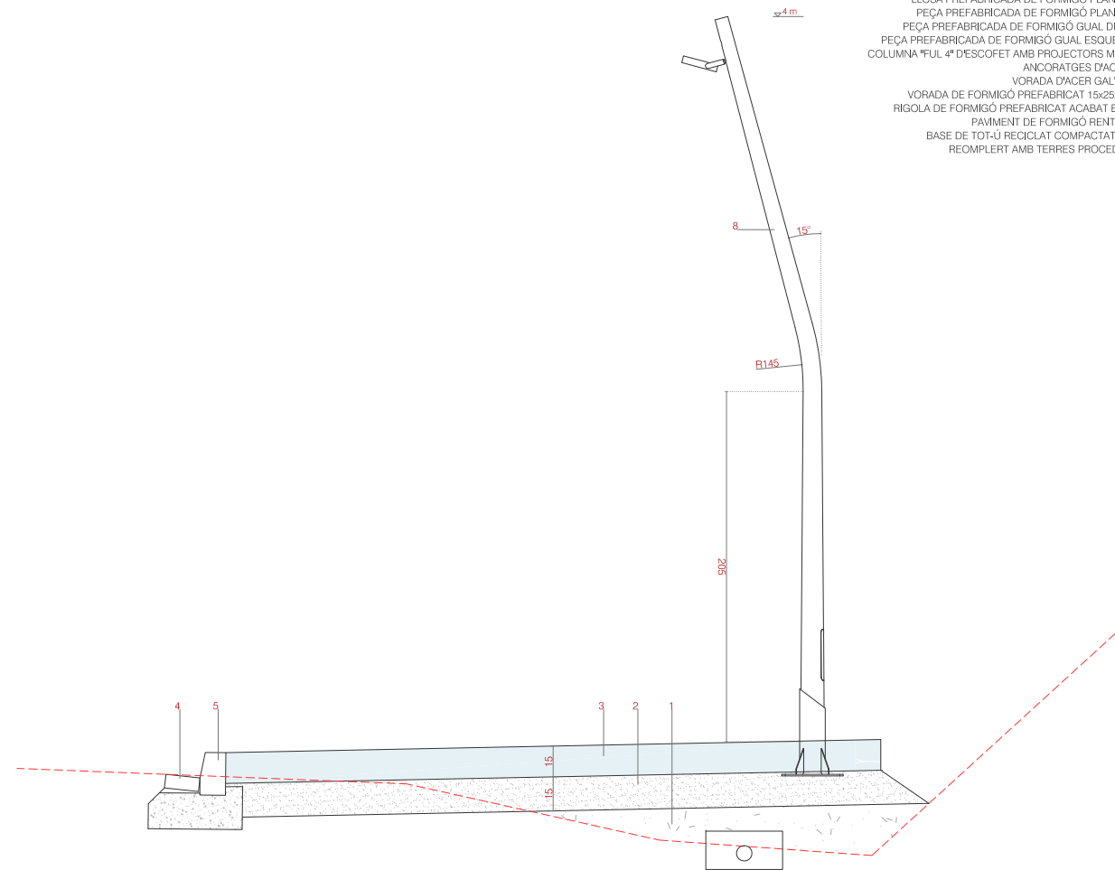
D05 SECCIÓ TIPUS
