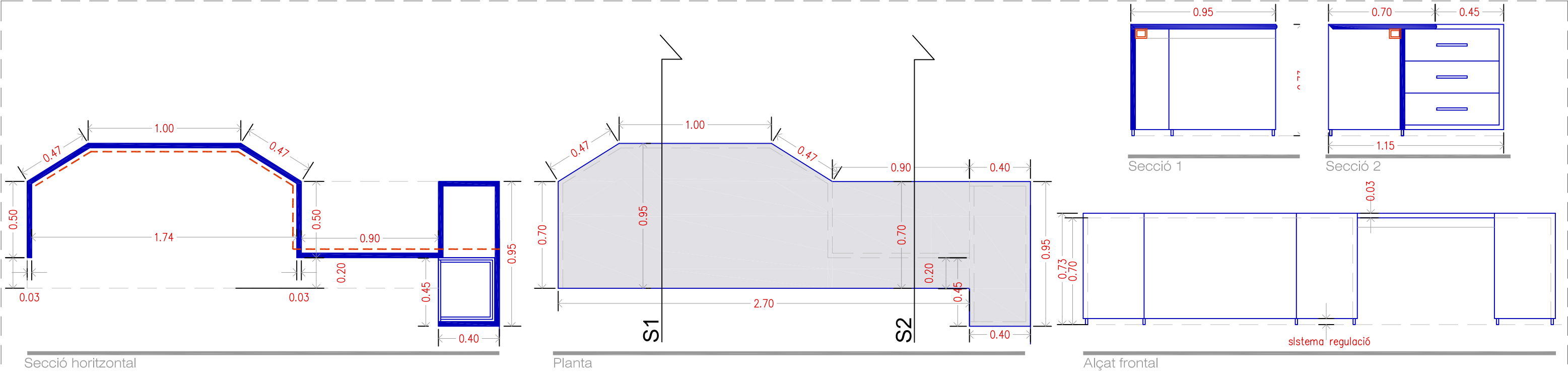
DETALL TAULELL ATENCIÓ AL PÚBLIC
