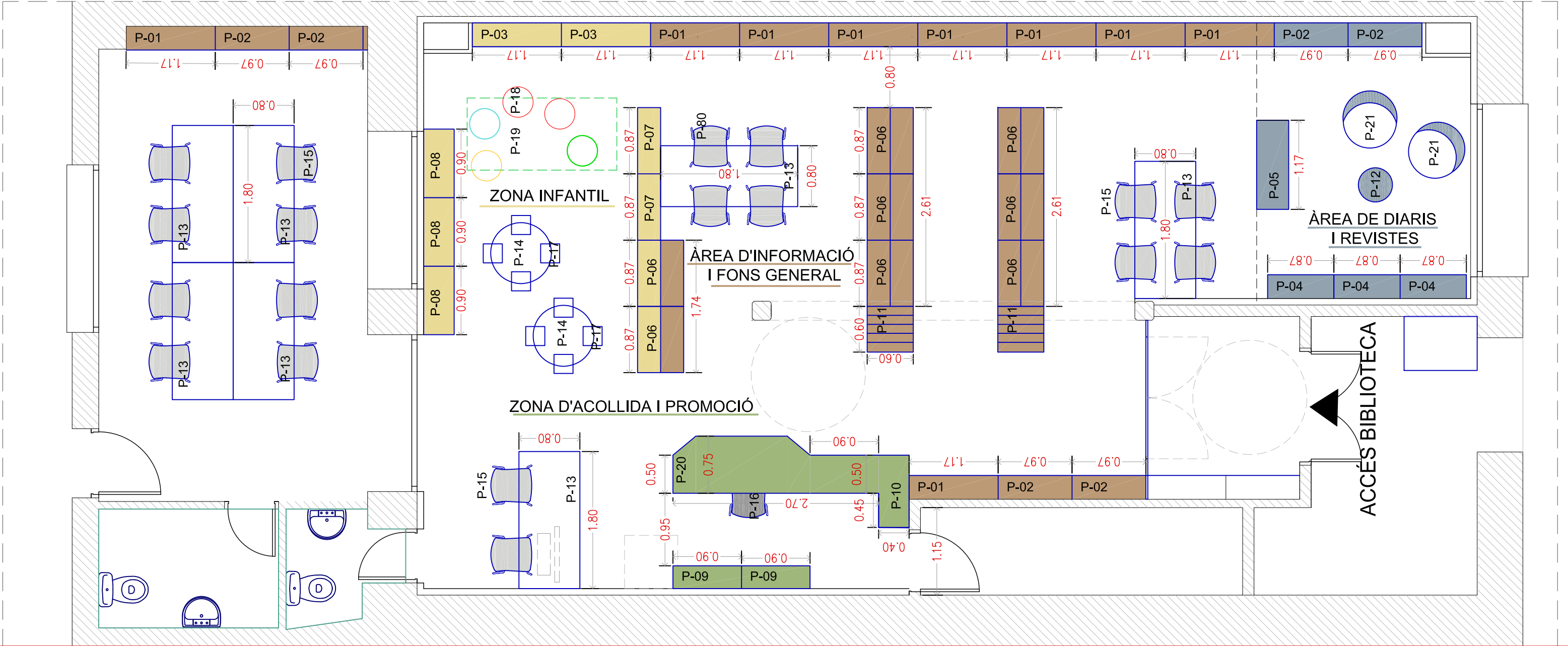
PLANTA MOBILIARI BIBLIOTECA D'ALBESA
