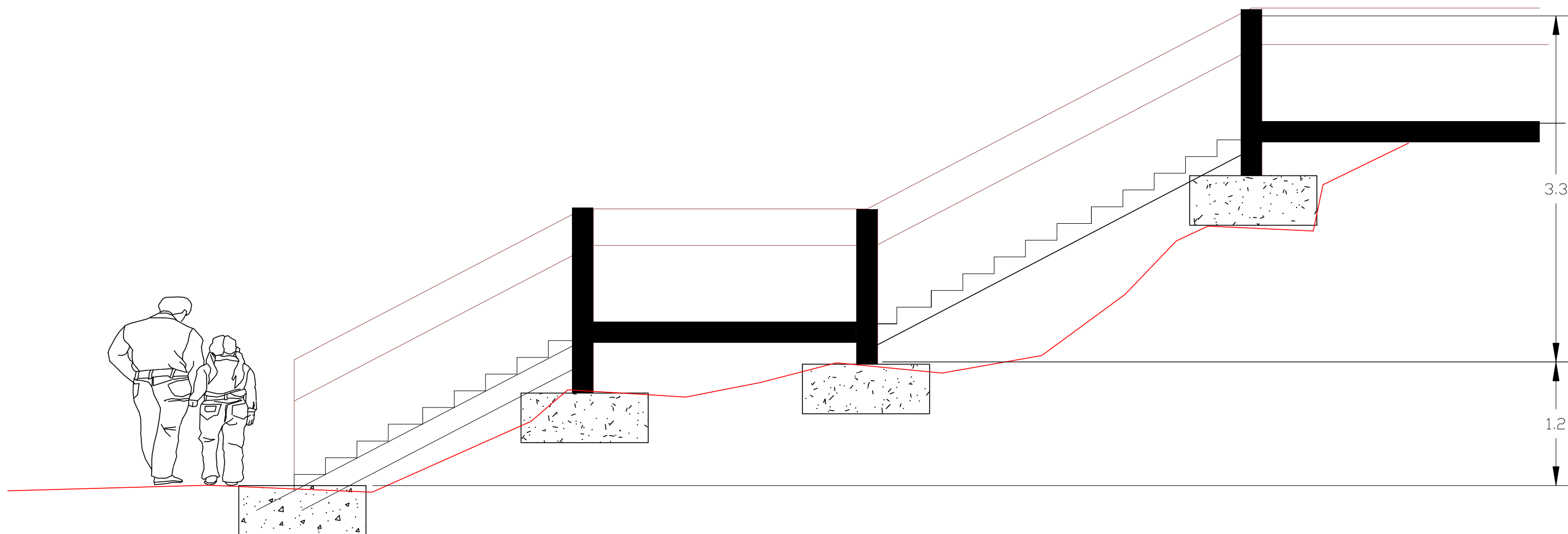
DETALL D'ESCALA DE FUSTA TRACTADA AMB AUTOCLAU D'UN METRE D'AMPLADA PER A SALVAR EL DESNIVELL EXISTENT
