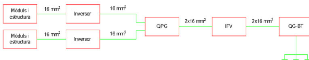
Fig. 6.3. Esquema general de la xarxa de preses de terra.
