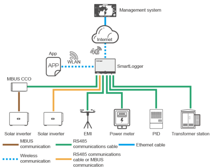
Fig. 6.1. Connexionat i funcionament del sistema de monitoratge.
