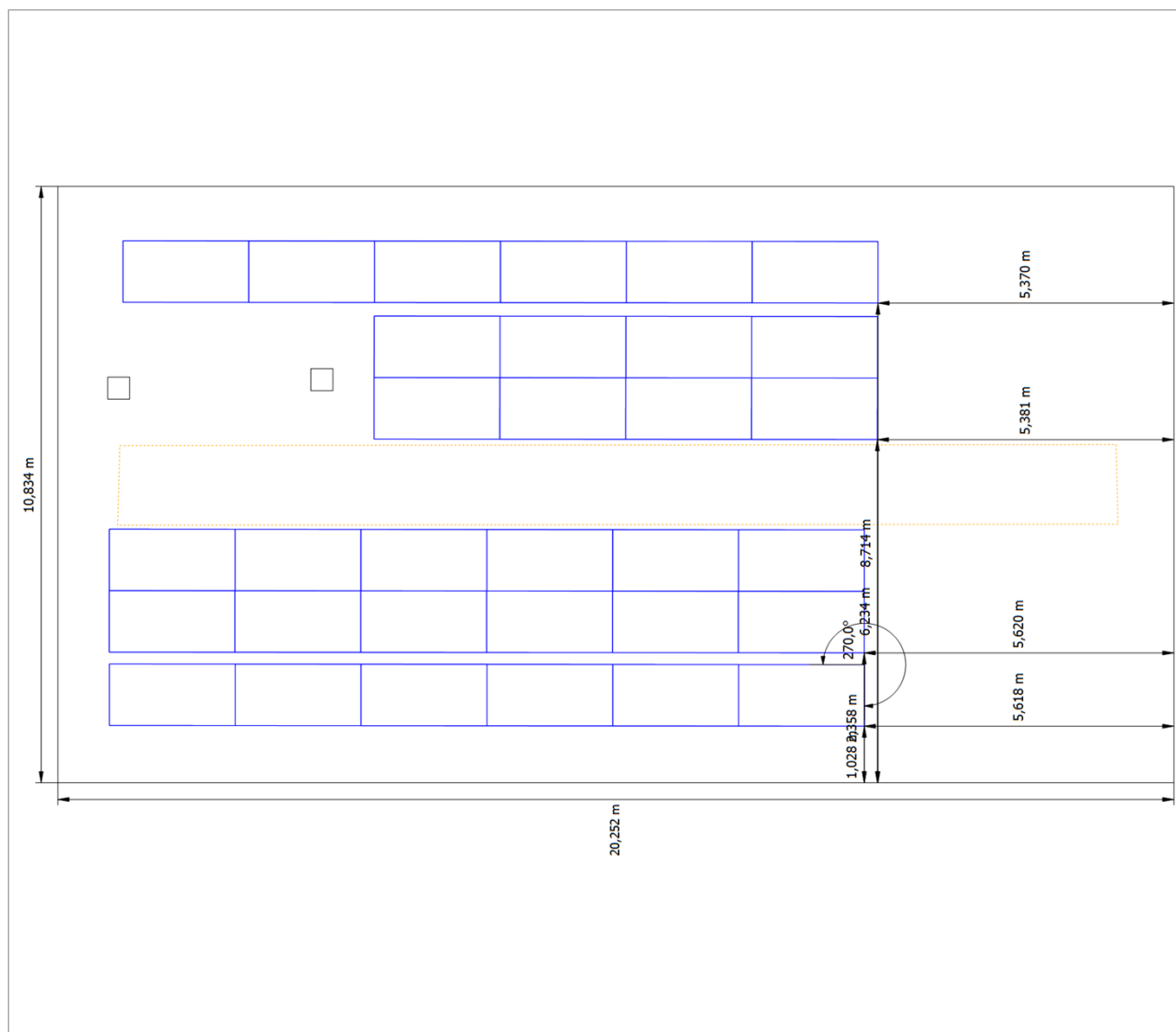
Figura: Edificio 03 - Superficie del tejado sur
