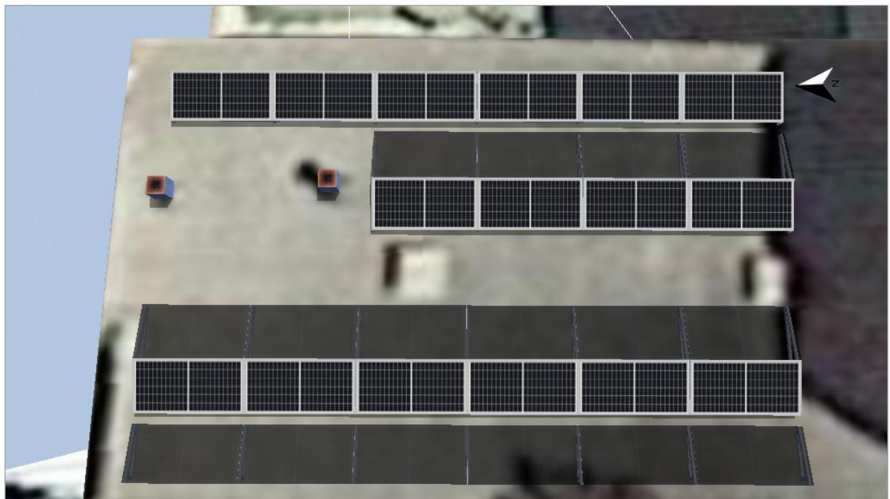
Figura: 2. Superficie fotovoltaica - Edificio 03-Superficie fotovoltaica Oeste
