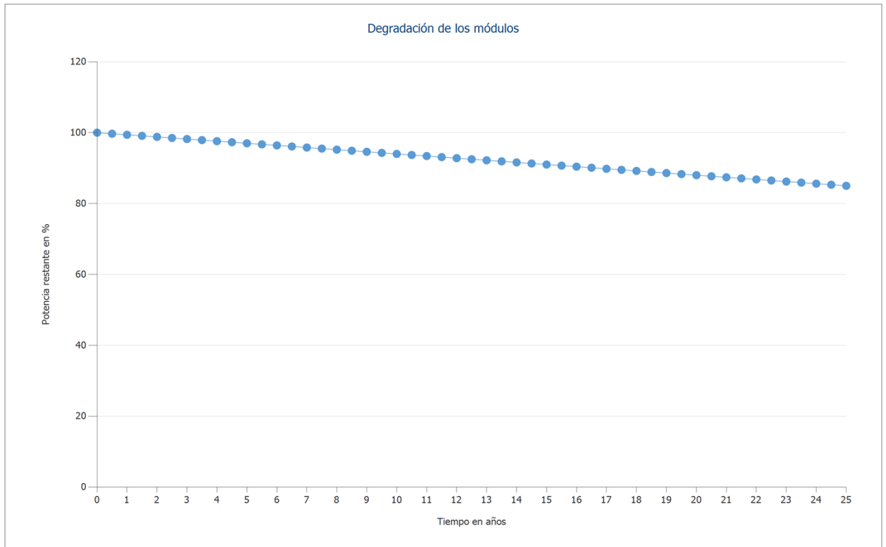
Figura: Degradación de los módulos, 2. Superficie fotovoltaica - Coberta baixa-Superficie a ocupar sur
