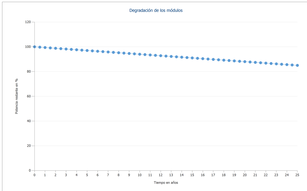
Figura: Degradación de los módulos, 1. Superficie fotovoltaica - Coberta alta-Superficie a ocupar norte
