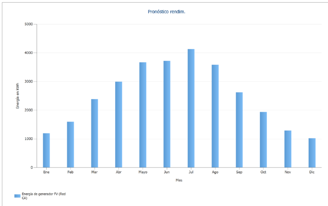
Il·lustració 6. Generació elèctrica anual
