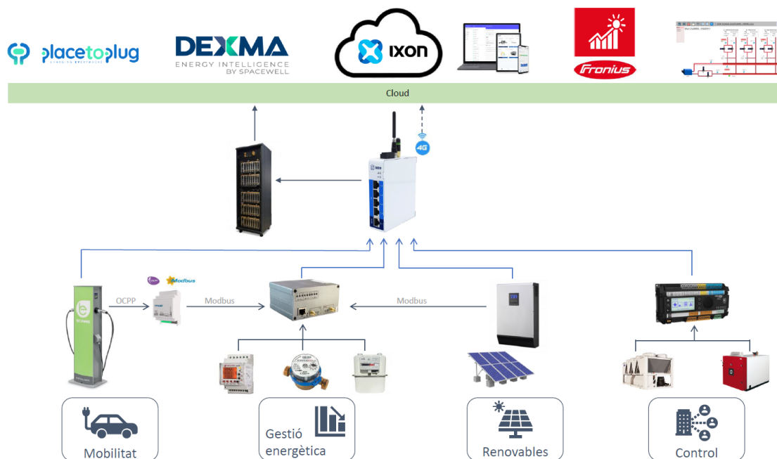
Il·lustració 9. Esquema de monitorització
