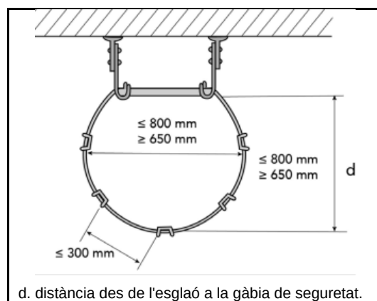
Figura 4. Distàncies lliures a l'interior d'una gàbia de seguretat
