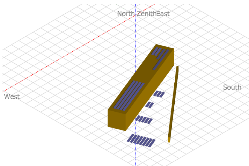
Il·lustració 5: Perspectiva del FV i
