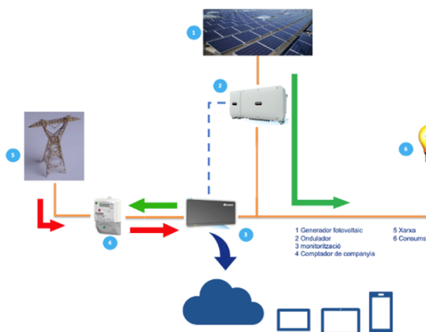
Il·lustració 4. Configuració bàsica proposada
