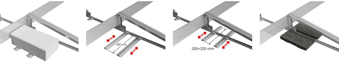
Ejemplo de contrapeso de hasta 400 mm de ancho sobre portalastre .
