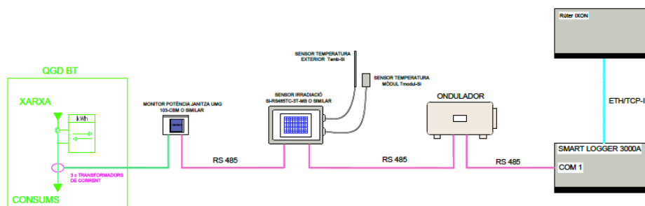
Il·lustració 7. Esquema bàsic de monitorització i comunicacions
