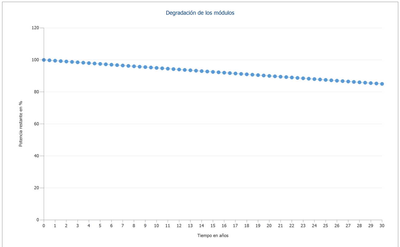
Figura: Degradación de los módulos, 3. Superficie fotovoltaica - Edificio 03-Superficie fotovoltaica Nordeste
