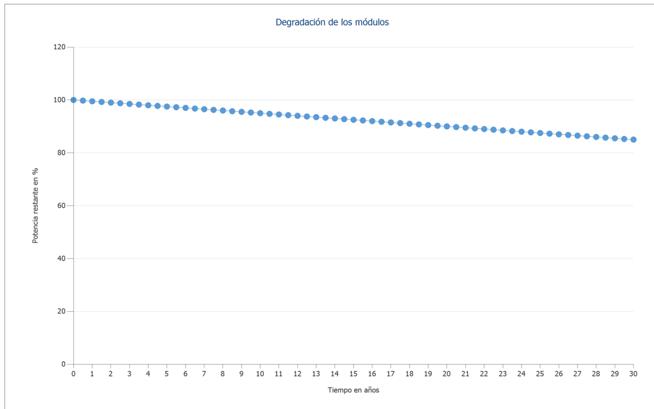
Figura: Degradación de los módulos, 1. Superficie fotovoltaica - Edificio 04-Superficie fotovoltaica Nordeste
