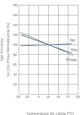
Isc, Voc y Pmax en función de la temperatura.
