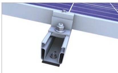
Fijación sobre el raíl corto en montajes horizontal
