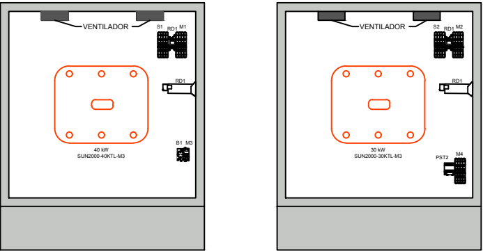
DETALL ARMARIS ONDULADORS I MUNTATGE INTERIOR QPCA
