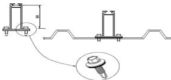
Il·lustració 7. Estructura de suport a la coberta
