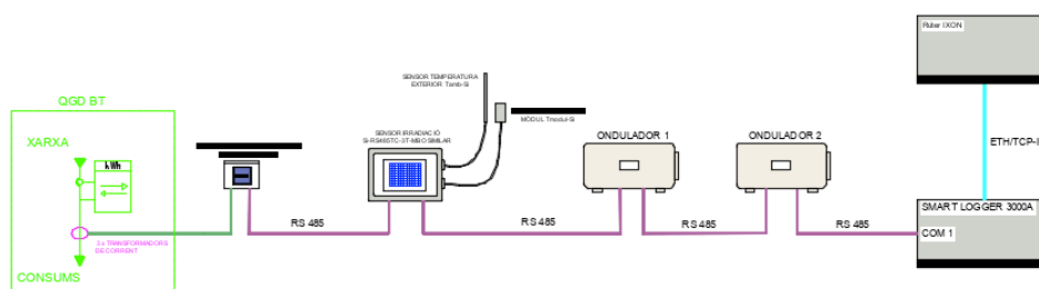
Il·lustració 6. Esquema bàsic de monitorització i comunicacions
