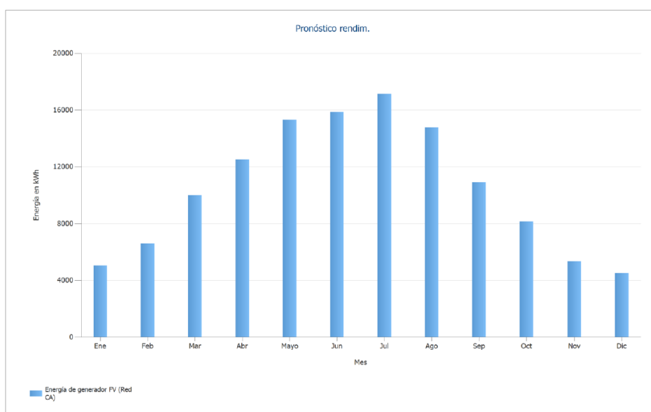
Il·lustració 6. Generació elèctrica anual
