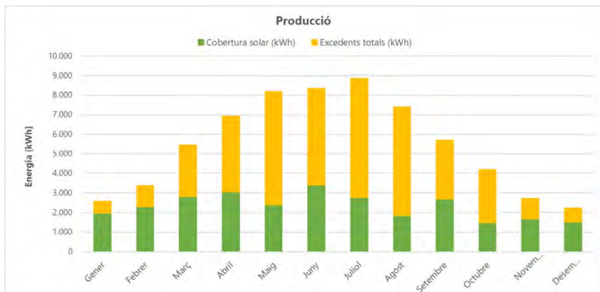
Fig. 7.4. Producció i excedents mensuals estimats.
