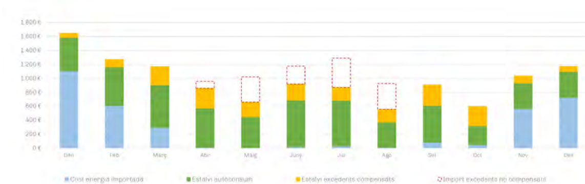
Fig. 7.5. Balanç energètic mensual estimat.
