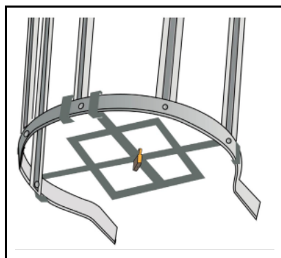
Figura 10. Mecanisme antiaccés.
