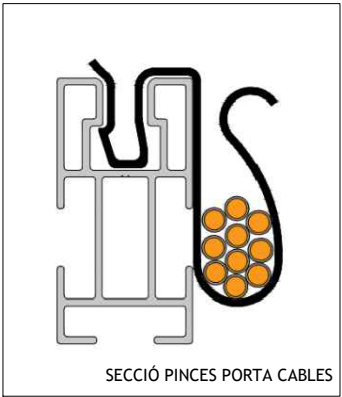
SECCIÓ PINCES PORTA CABLES
