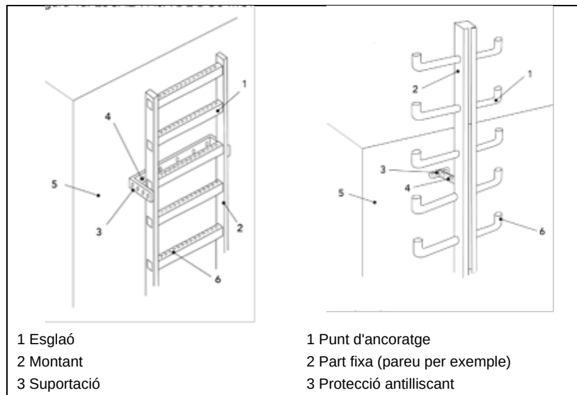
Figura 1a. Escalera fixa de dos muntants Figura 1b. Escalera fixa d'un sol muntant
