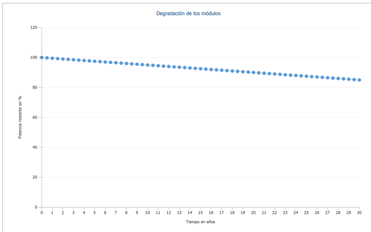
Figura: Degradación de los módulos, 1. Superficie fotovoltaica - Gimnàs-Superficie del tejado sur
