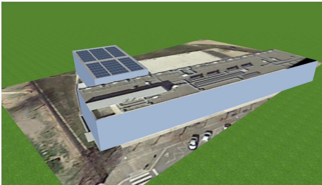
Il·lustració 5. Visualització 3D del camp fotovoltaic
