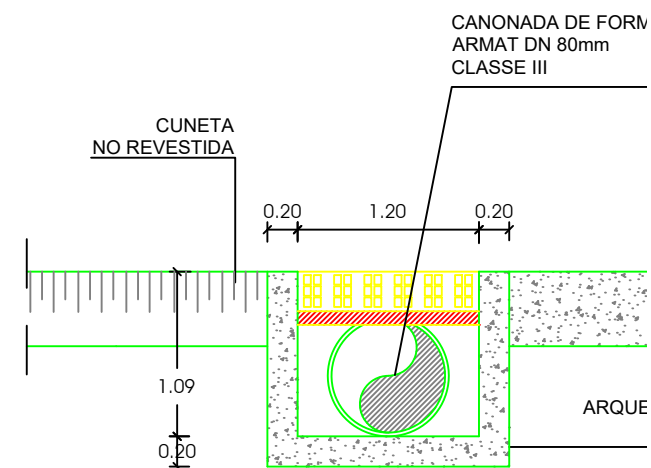
SECCIÓ C-C'
