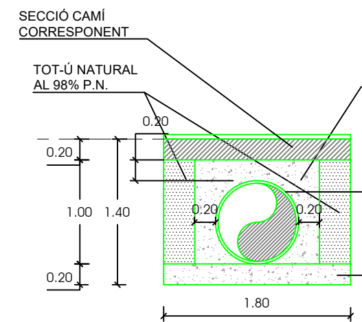
SECCIÓ B-B'
