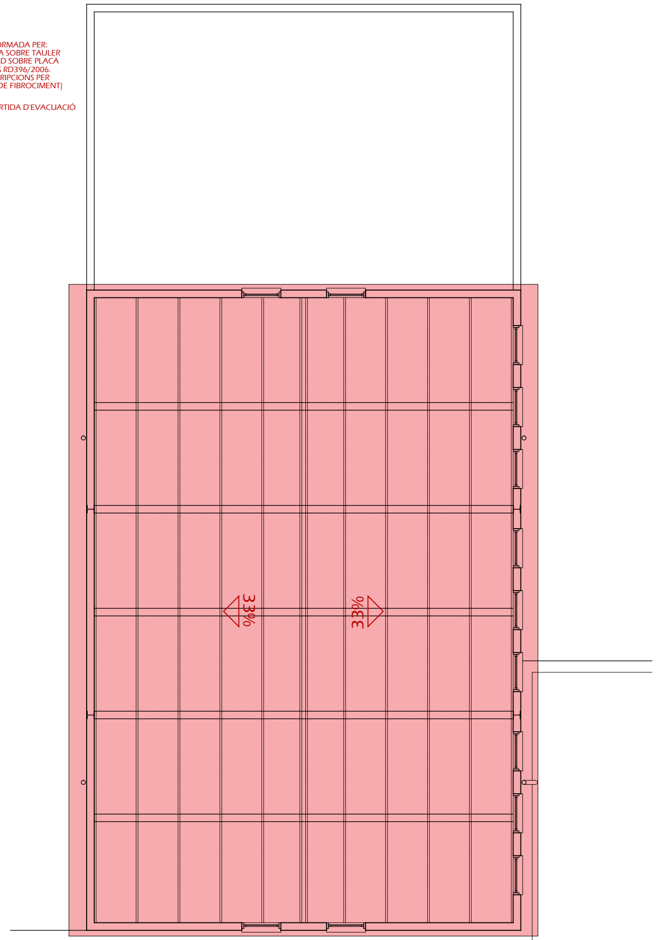
PLANTA COBERTA 1
