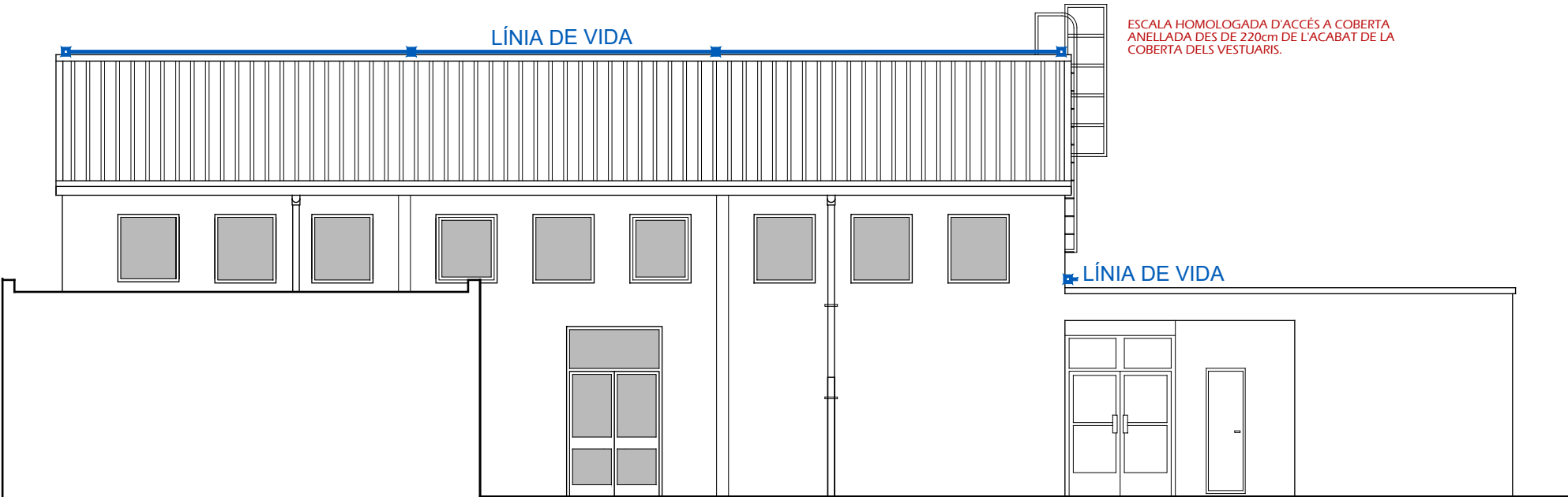
FAÇANA SUD
