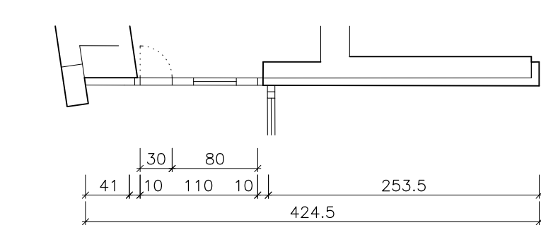
PLANTA E:1/50
