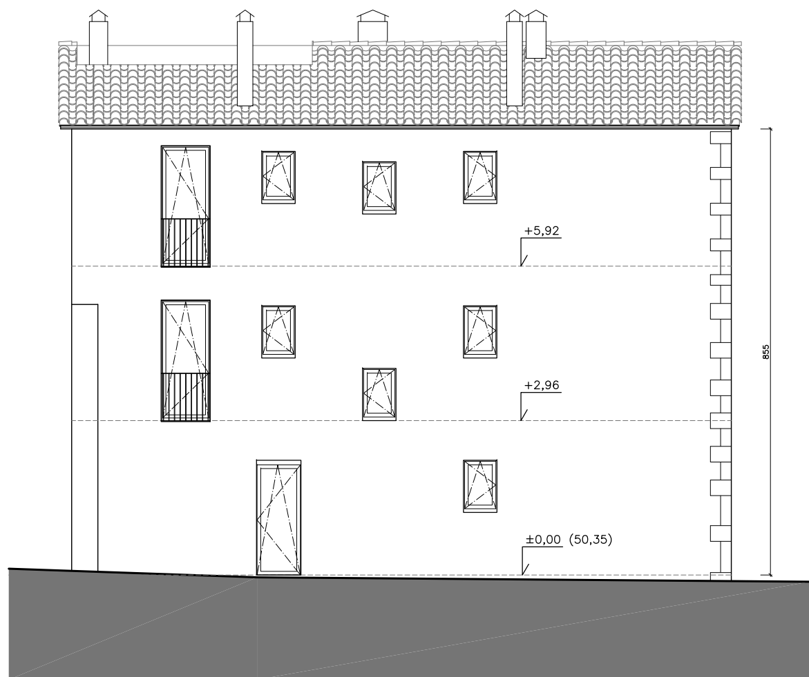
ALÇAT OEST E:1/100
