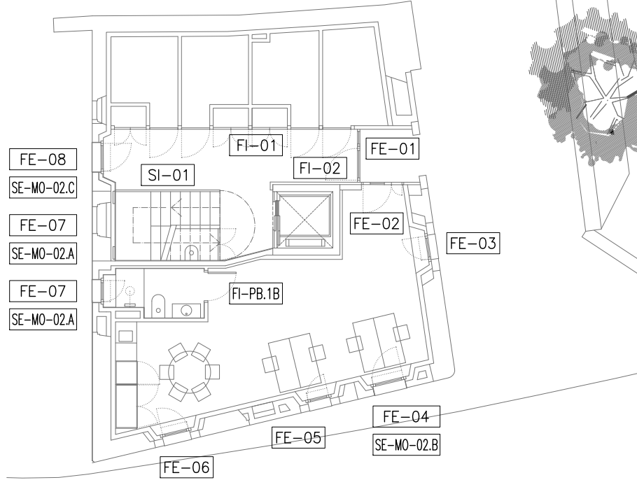
PLANTA BAIXA E:1/150
