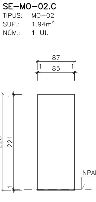
ALÇAT EXT. E:1/50
