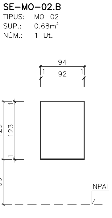
ALÇAT EXT. E:1/50
