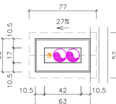
PLANTA E:1/25
