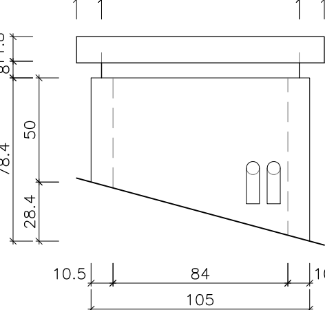
ALÇAT 1 E:1/25
