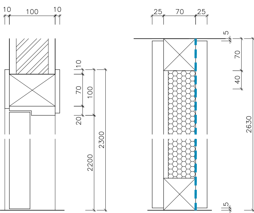
SECCIÓ VERTICAL V1-V1' E:1/5 SECCIÓ VERTICAL V2-V2' E:1/5
