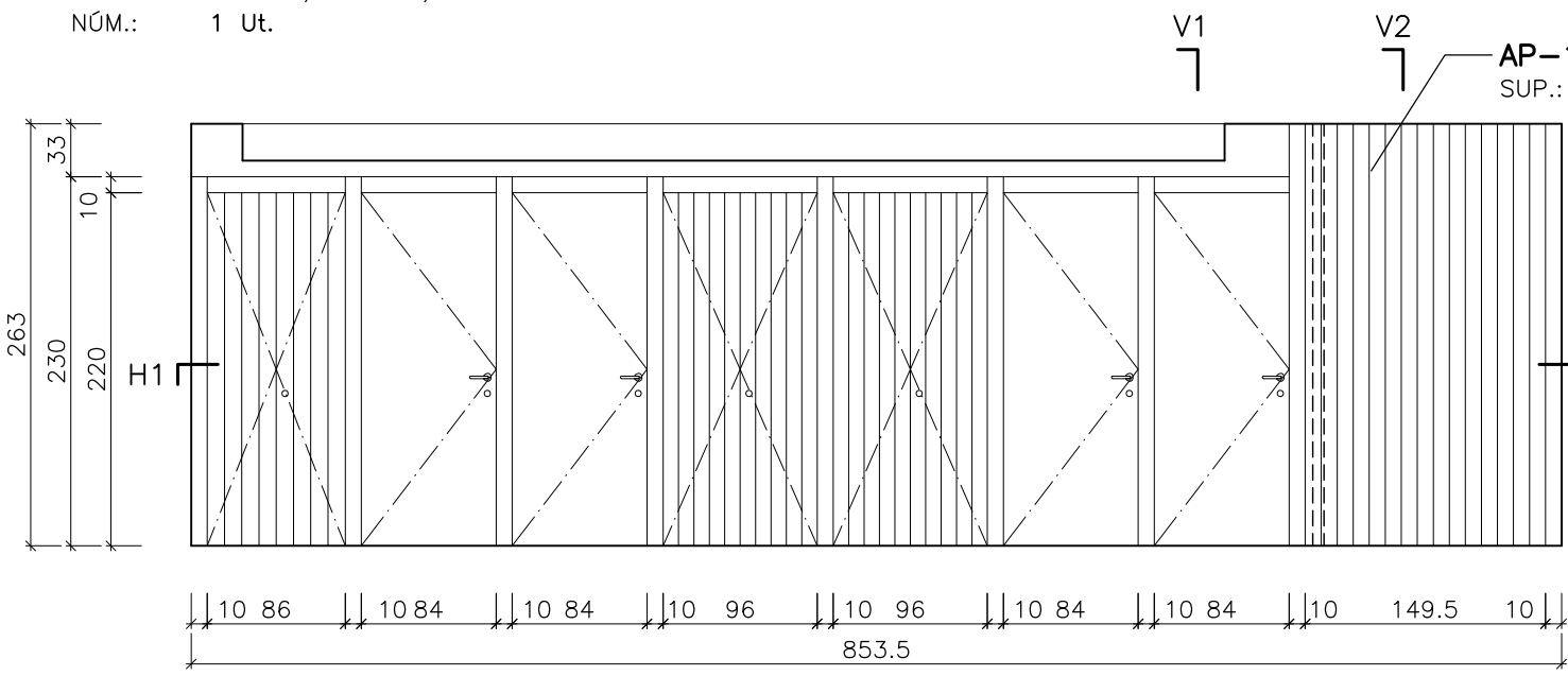
ALÇAT EXTERIOR E:1/50
