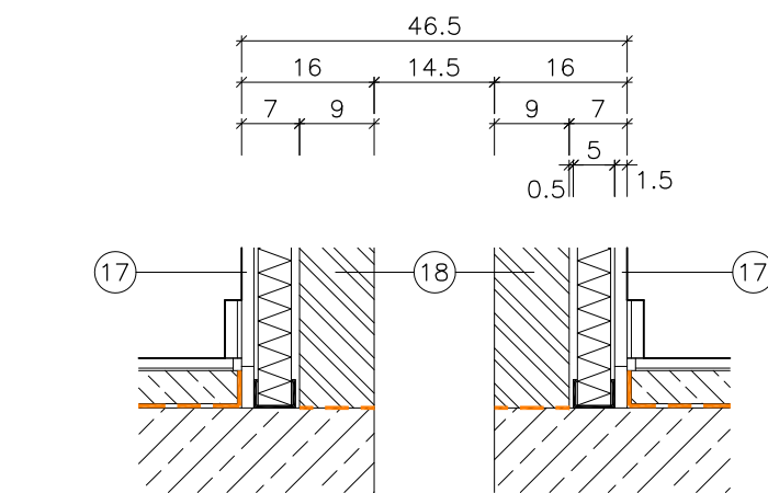
SECCIÓ F E:1/10 (SEPARACIÓ ENTRE HABITATGES)
