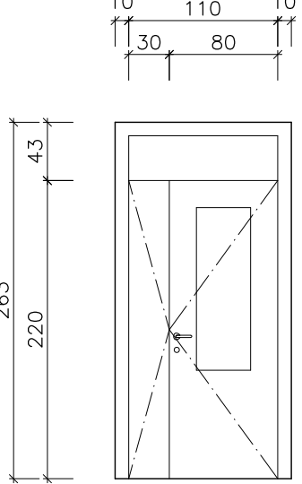
ALÇAT EXTERIOR E:1/50
