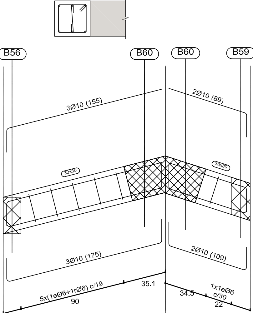
Pòrtic - 2
