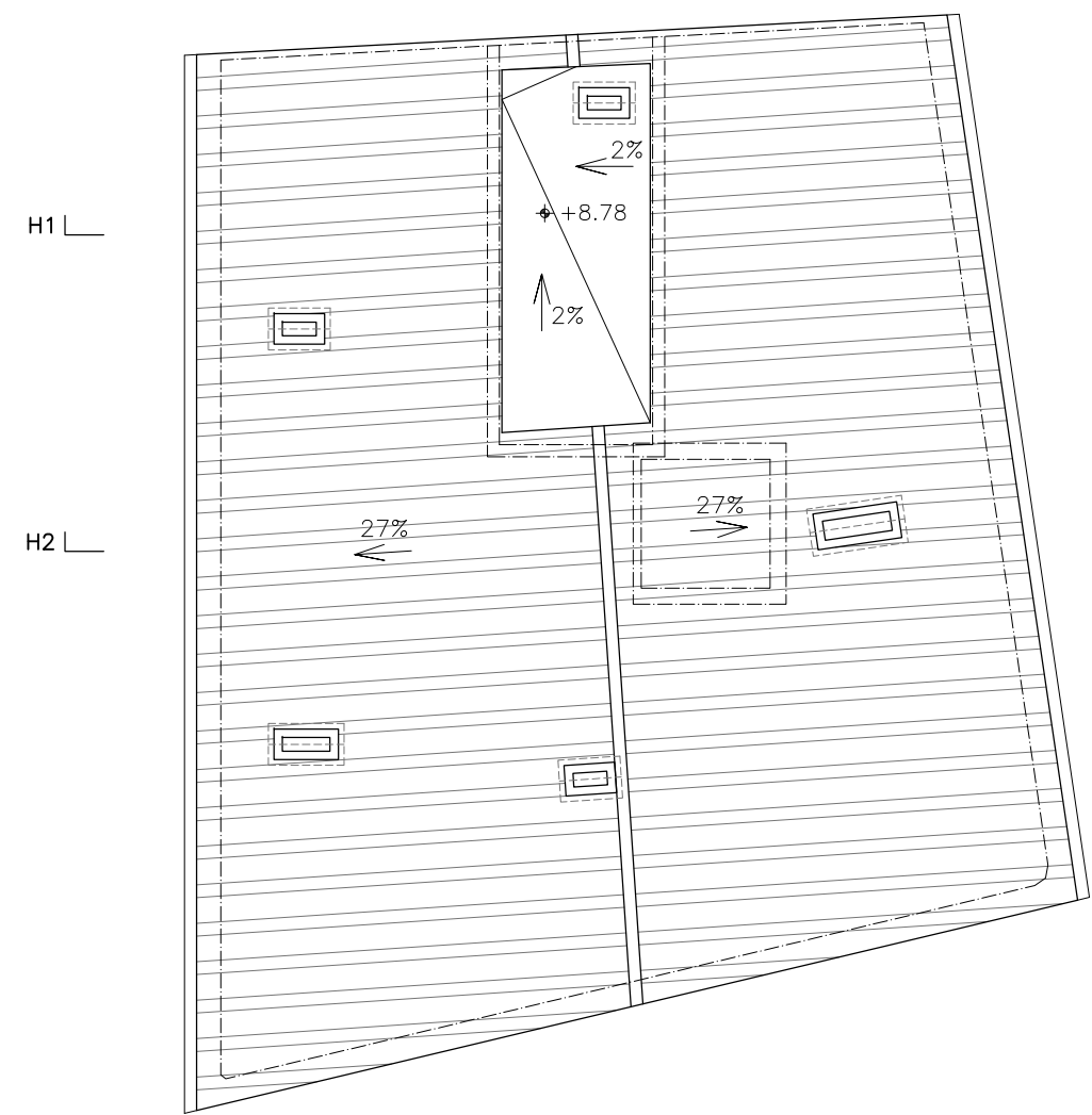
PROPOSTA PLANTA COBERTA E:1/100
