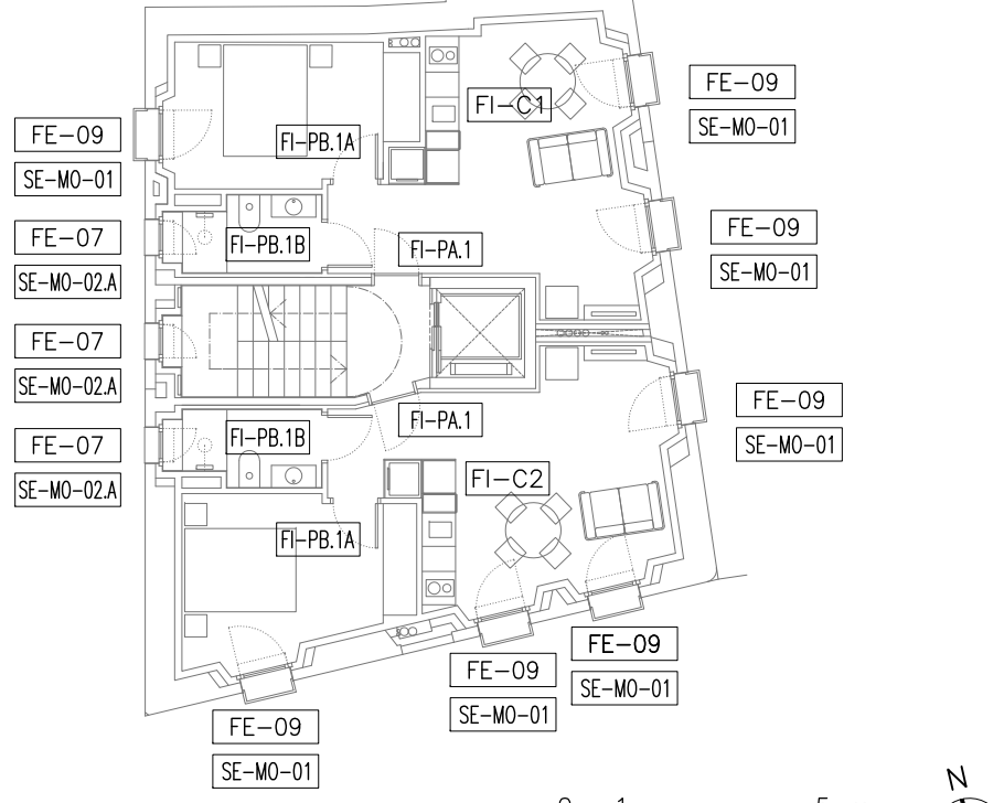
PLANTA PRIMERA E:1/150
