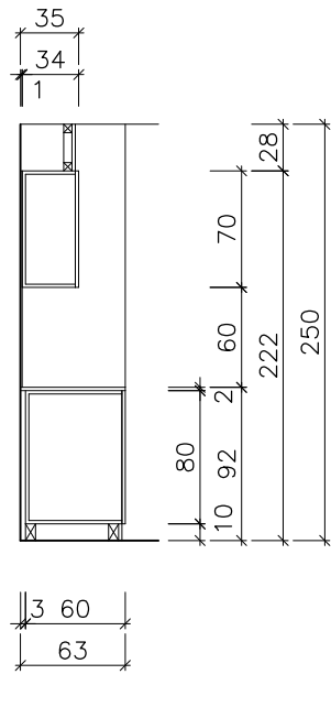
SECCIÓ C5-C5' E:1/50
