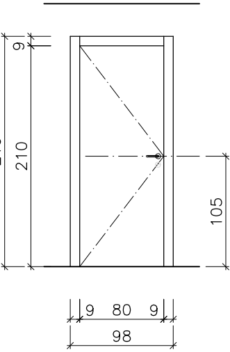
ALÇAT E:1/50
