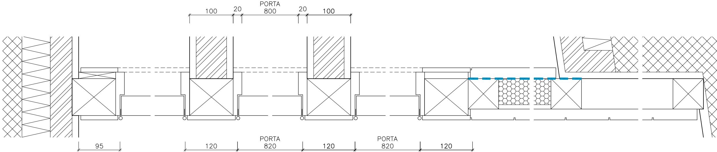
SECCIÓ HORIZONTAL H1-H1' E:1/5
