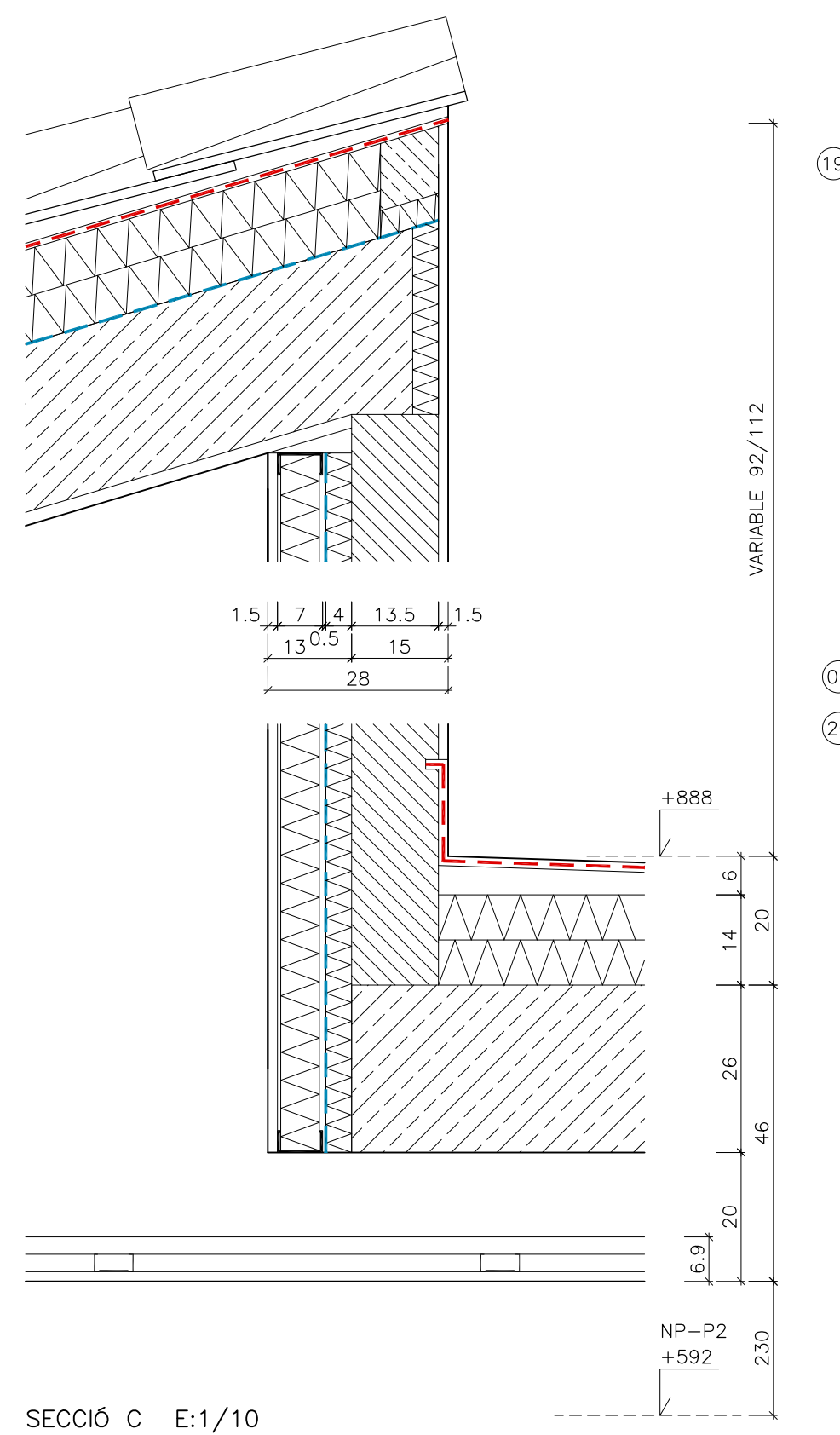
SECCIÓ C E:1/10
