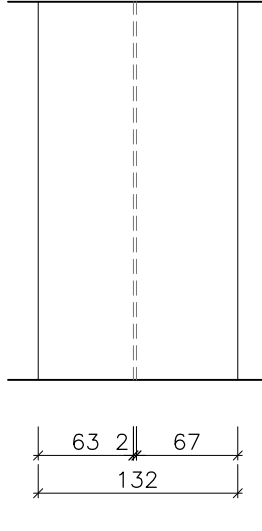
SECCIÓ C2-C2'
