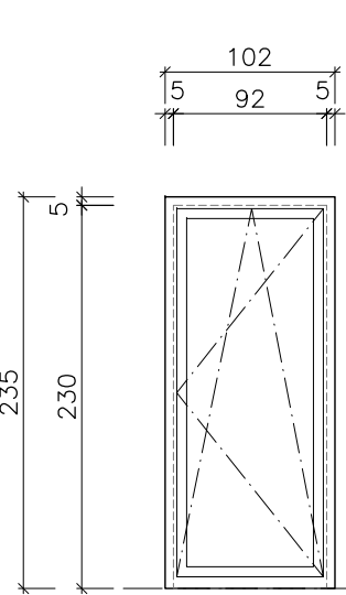
ALÇAT EXTERIOR E:1/50
