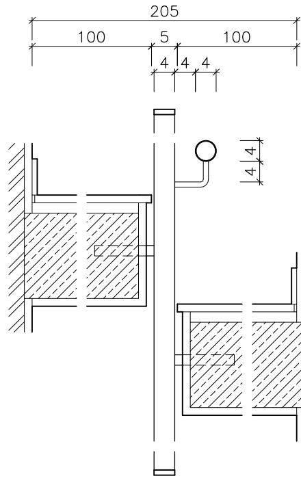
SECCIÓ TRANSVERSAL ESCALA E:1/10
