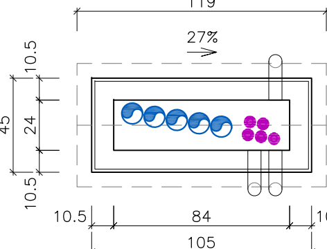
PLANTA E:1/25
