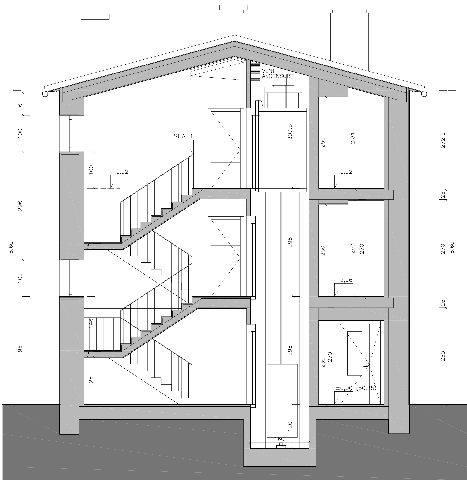
SECCIÓ H2 E:1/50
