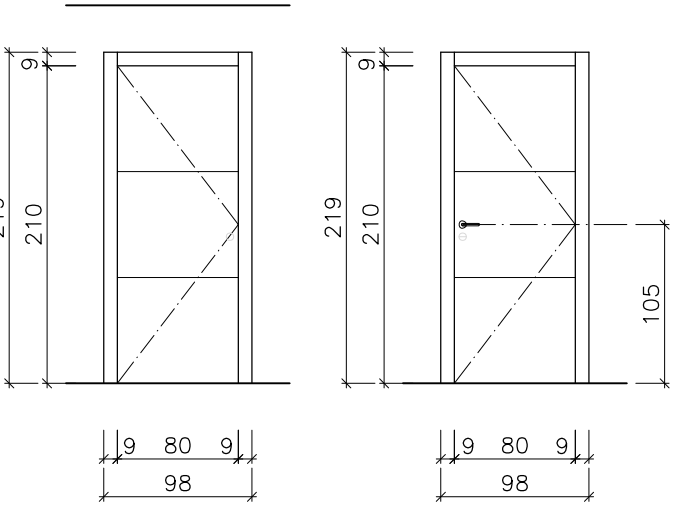
ALÇAT EXT. E:1/50 ALÇAT INT. HAB. E:1/50
