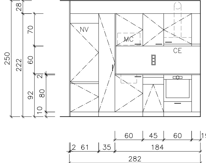
SECCIÓ C4-C4' E:1/50
