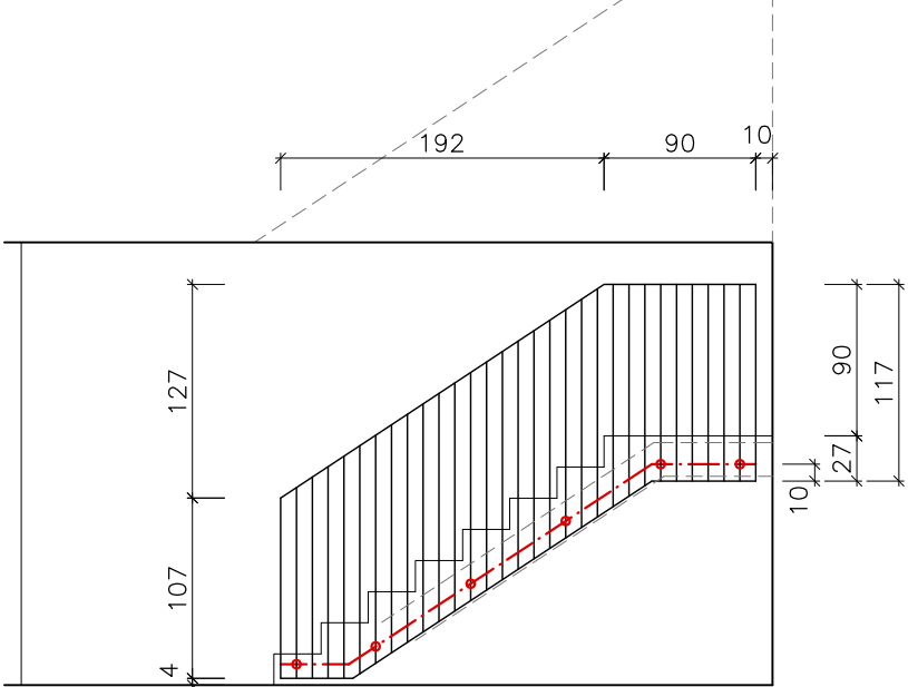
ALÇAT PRIMER TRAM E:1/50
