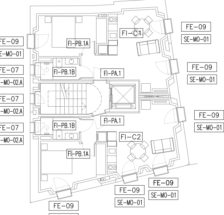
PLANTA PRIMERA E:1/150
