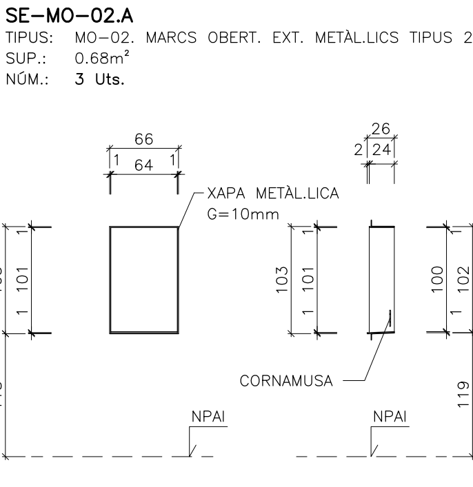
ALÇAT EXTERIOR E:1/50
