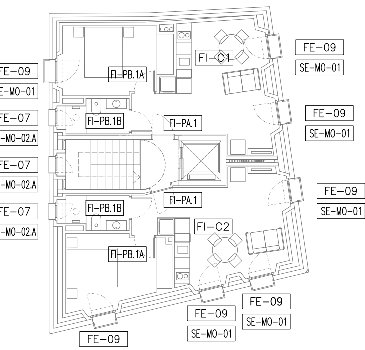
PLANTA SEGONA E:1/150
