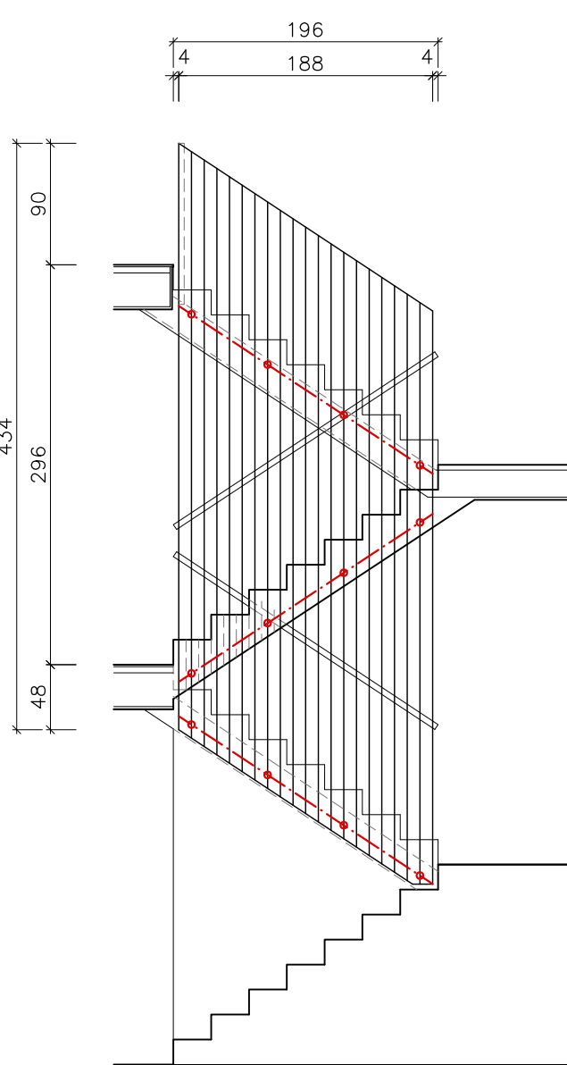
ALÇAT SEGON TRAM E:1/50
