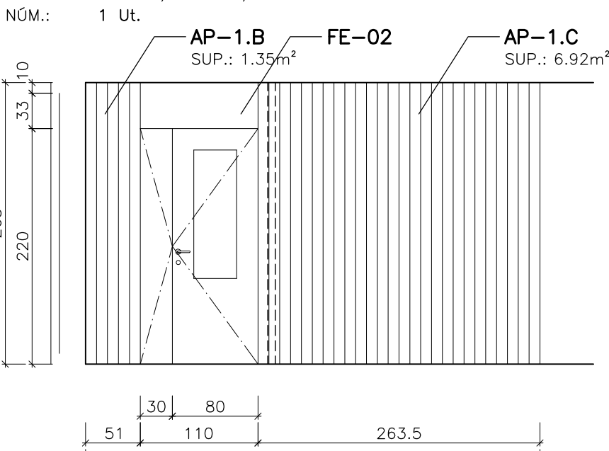
ALÇAT EXTERIOR E:1/50
