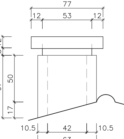
ALÇAT 1 E:1/25
