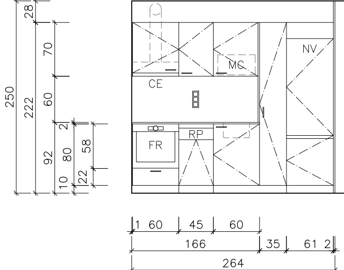
SECCIÓ C1-C1' E:1/50
