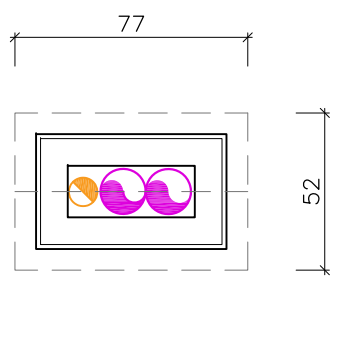
PLANTA E:1/25
