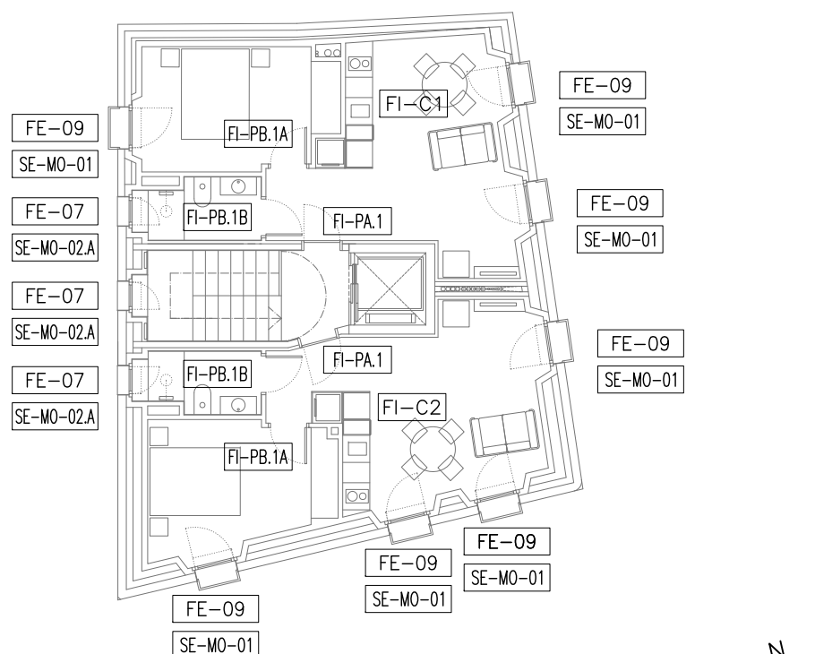
PLANTA SEGONA E:1/150
