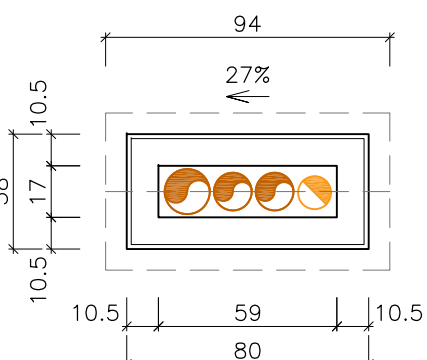
PLANTA E:1/25
