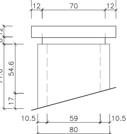
ALÇAT 1 E:1/25
