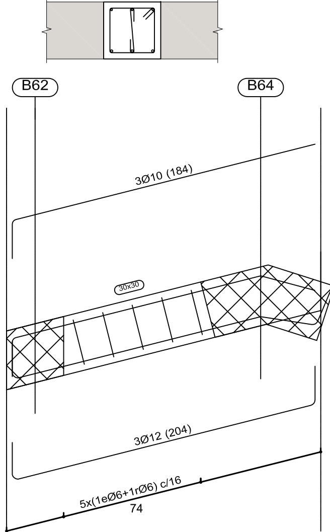
Pòrtic - 1
