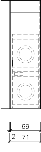
SECCIÓ C3-C3'
