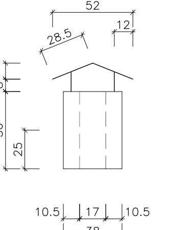
ALÇAT 2 E:1/25
