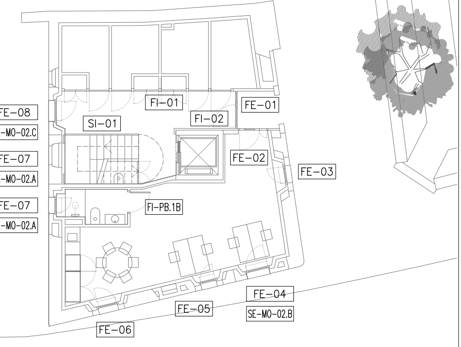
PLANTA BAIXA E:1/150
