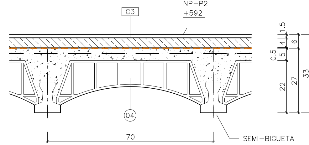
SECCIÓ E E:1/10 (TERRA PLANTA PRIMERA)
