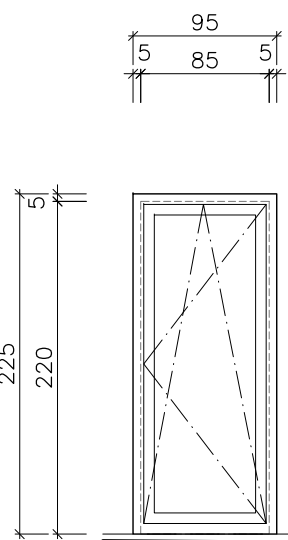
ALÇAT EXTERIOR E:1/50
