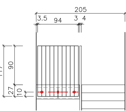
ALÇAT TRAM REPLÀ E:1/50
