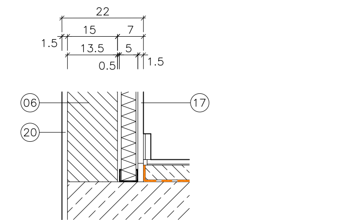
SECCIÓ G E:1/10 (SEPARACIÓ HABITATGES ESCALA)
