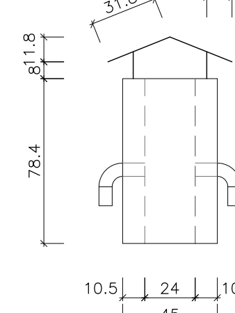
ALÇAT 2 E:1/25
