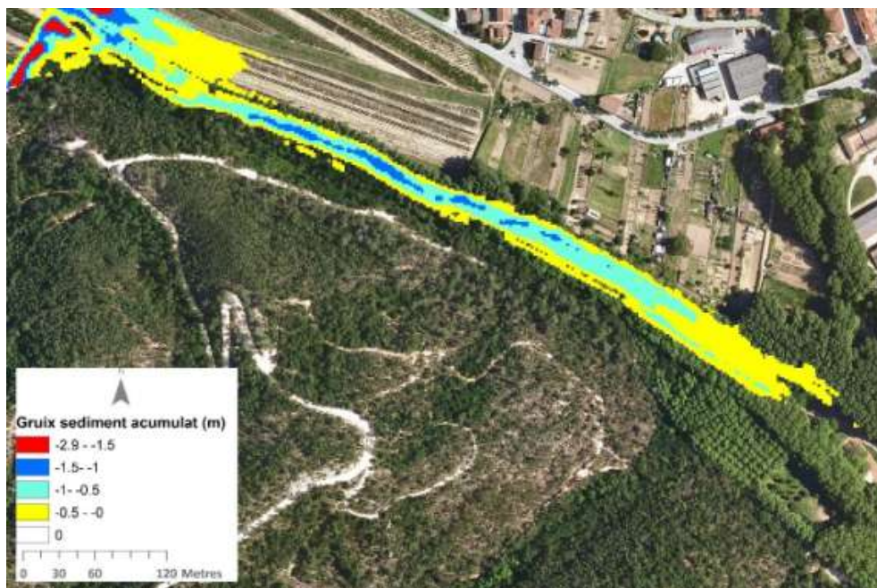
Figura 17. Estimació de la distribució del gruix de sediment acumulat a la llera en el tram d'estudi pel model hidràulic. El sediment acumulat presenta un gruix i distribució molt semblant a l'observat a camp (Figura 16).
