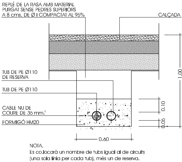
DETALL CONDUCCIÓ SOTA VIAL
