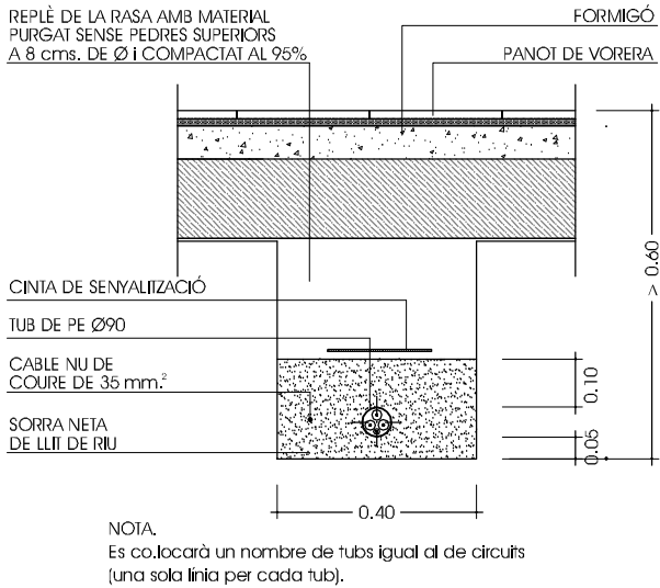
DETALL CONDUCCIÓ SOTA VORERA
