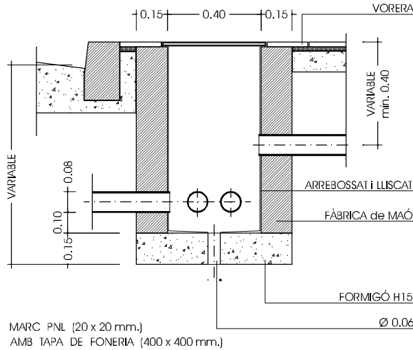
DETALL TRONETA TIPUS SECCIÓ
