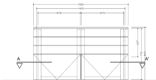
ALÇAT FRONTAL
