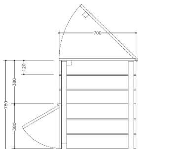
ALÇAT LATERAL
