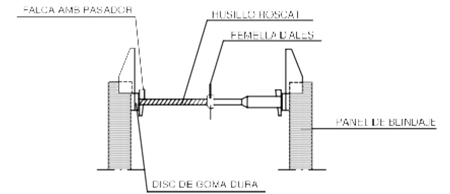
DETALL "A"
