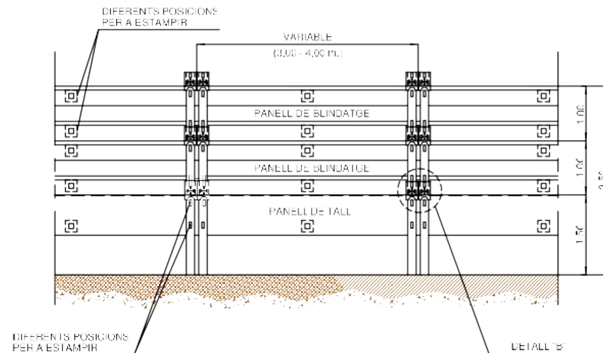
ALÇAT
