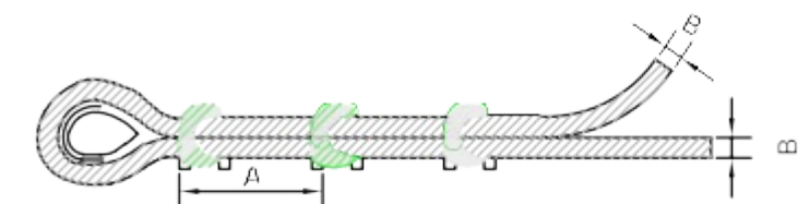
A= 6 a 8 vegades el diàmetre del cable B
