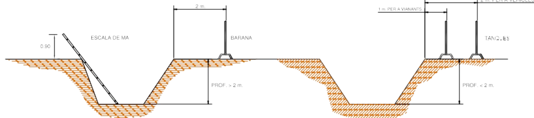
COL·LOCACIO DE TANCAMENT EN RASES
