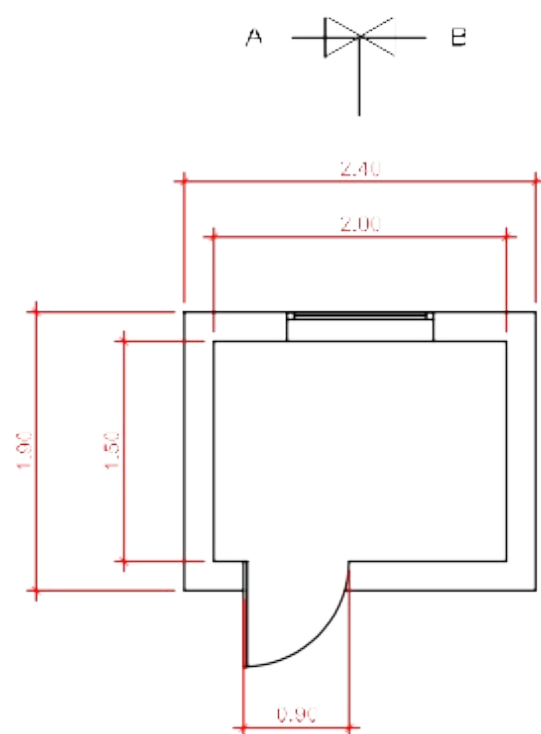
PLANTA
