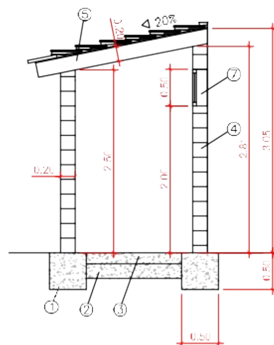
SECCIÓ A-B
