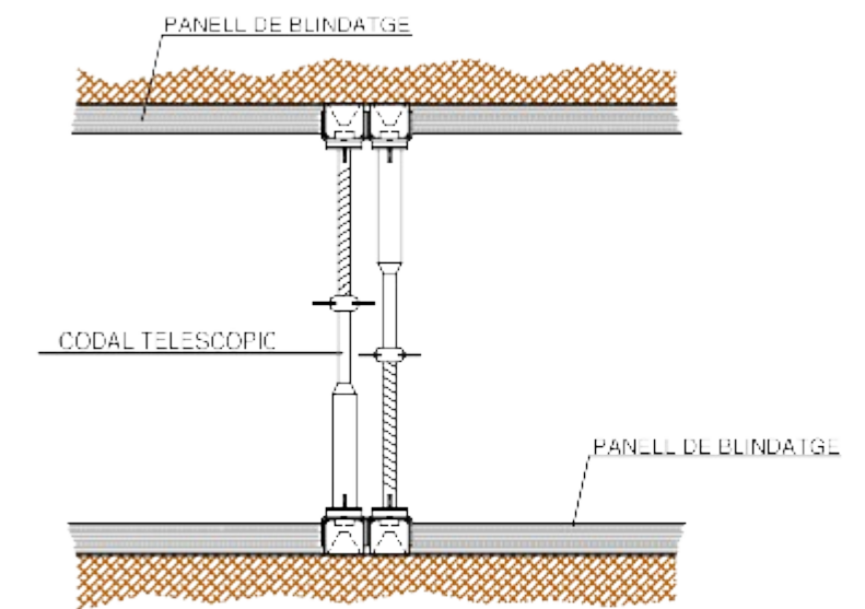
DETALL "C"
