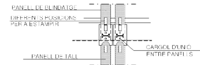
DETALL "B"
