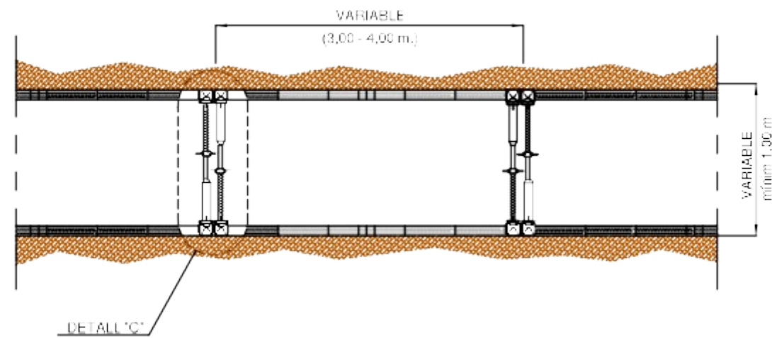
PLANTA
