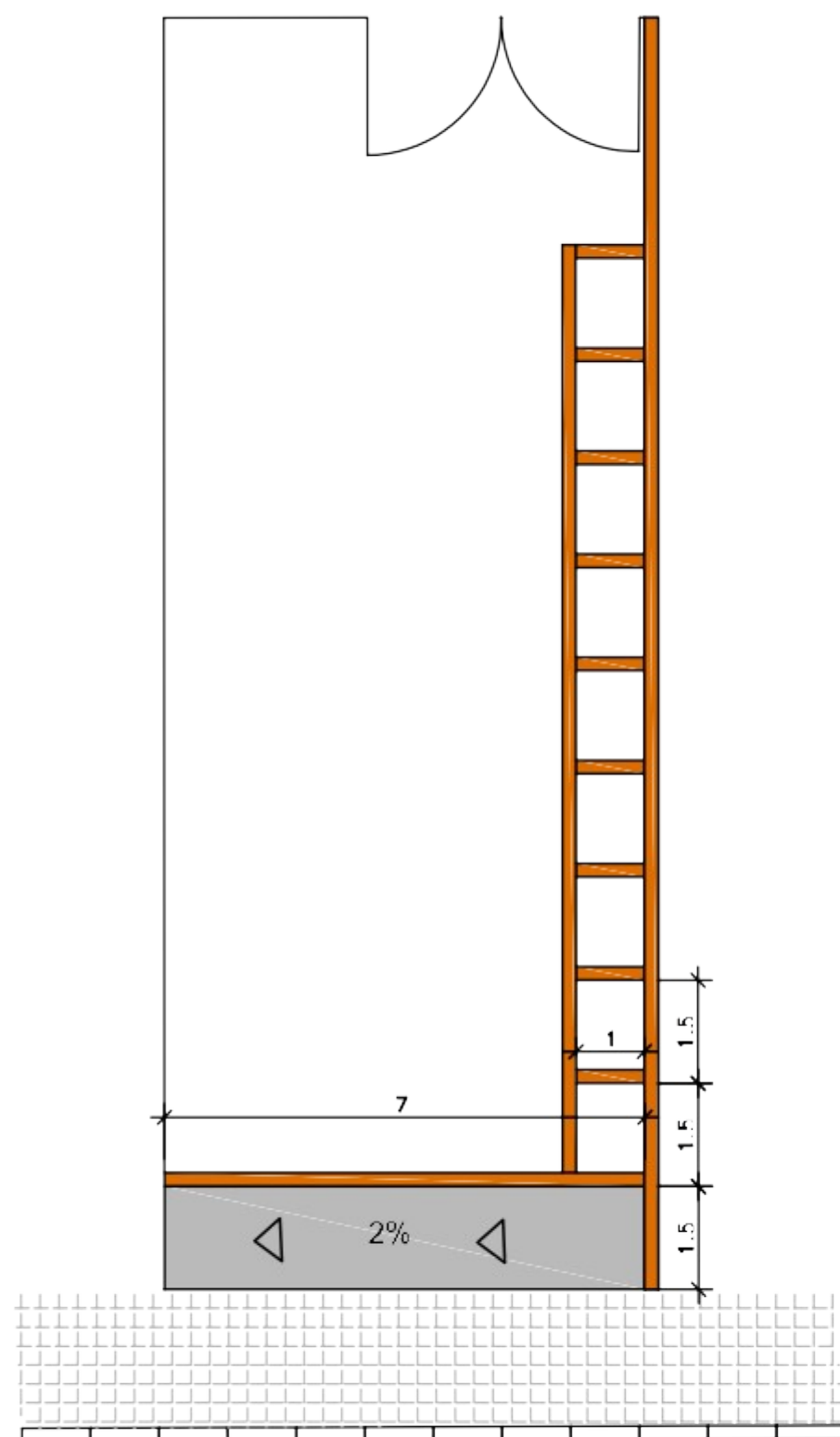
PLANTA
