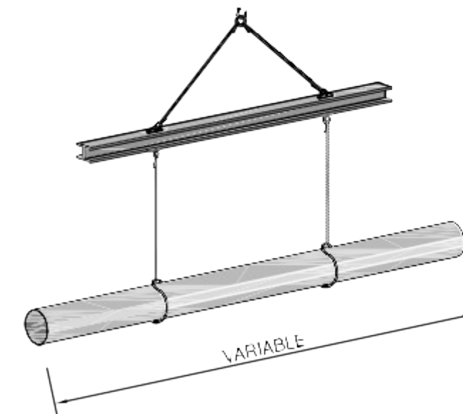
COL·LOCACIO DE LES GRAPES EN CABLES DE CARREGUES
