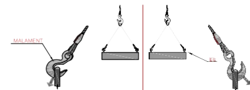
GANXO AMB OJAL (OBERTURA EXTERIOR DE LA CARREGA)
