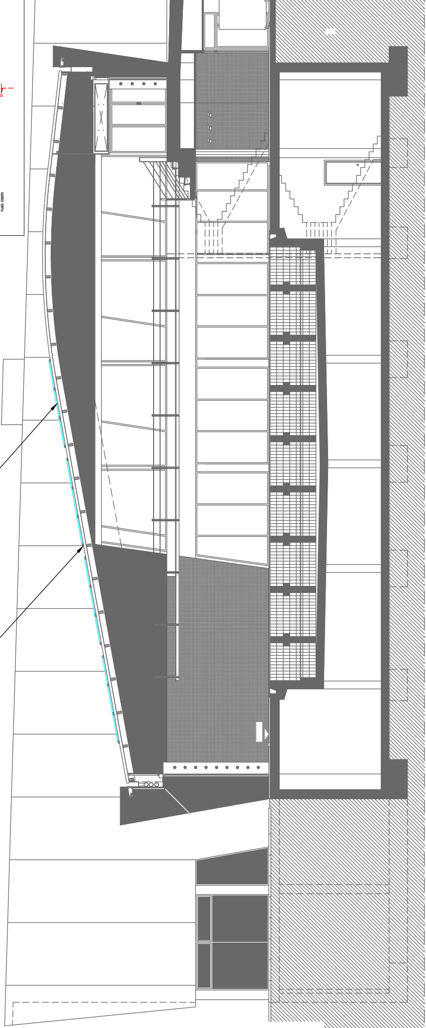
SECCIÓ TRANSVERSAL B-B'
