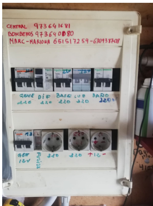
Quadro instal·lació elèctrica interior
