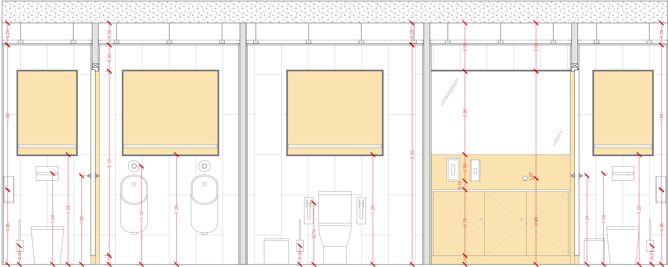
ALÇAT 14
