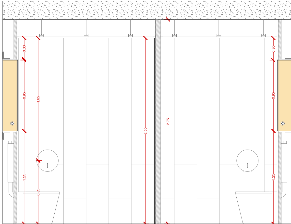
ALÇAT 10
