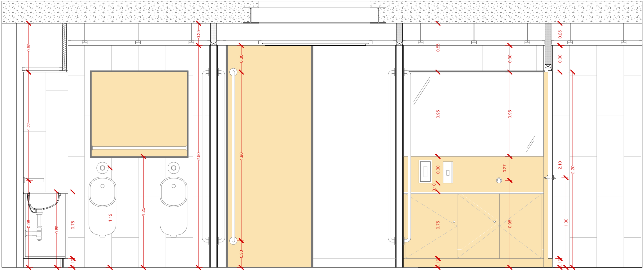
ALÇAT 12
