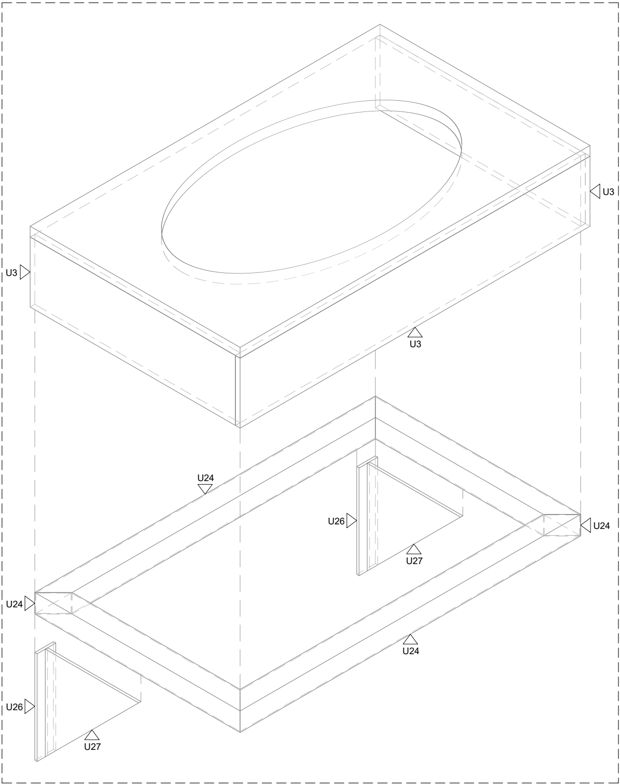
DETALL 09.5
