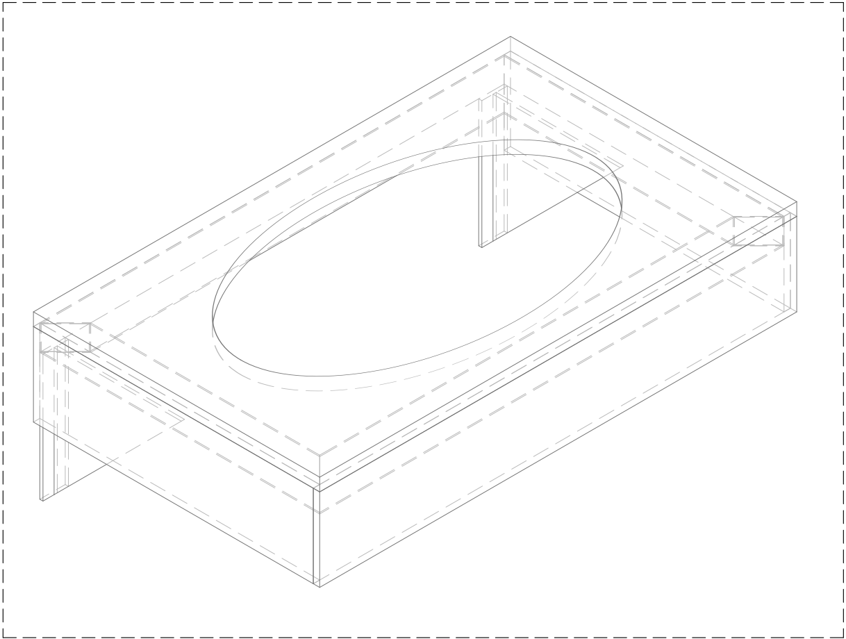
DETALL 09.4
