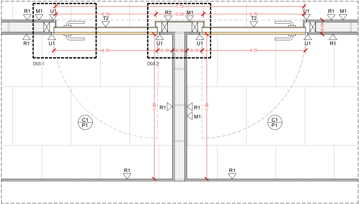
DETALL 03
