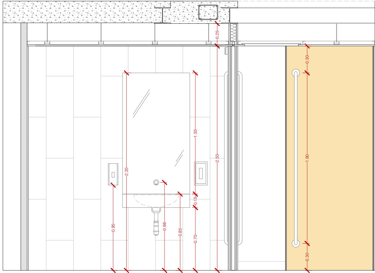
ALÇAT 06
