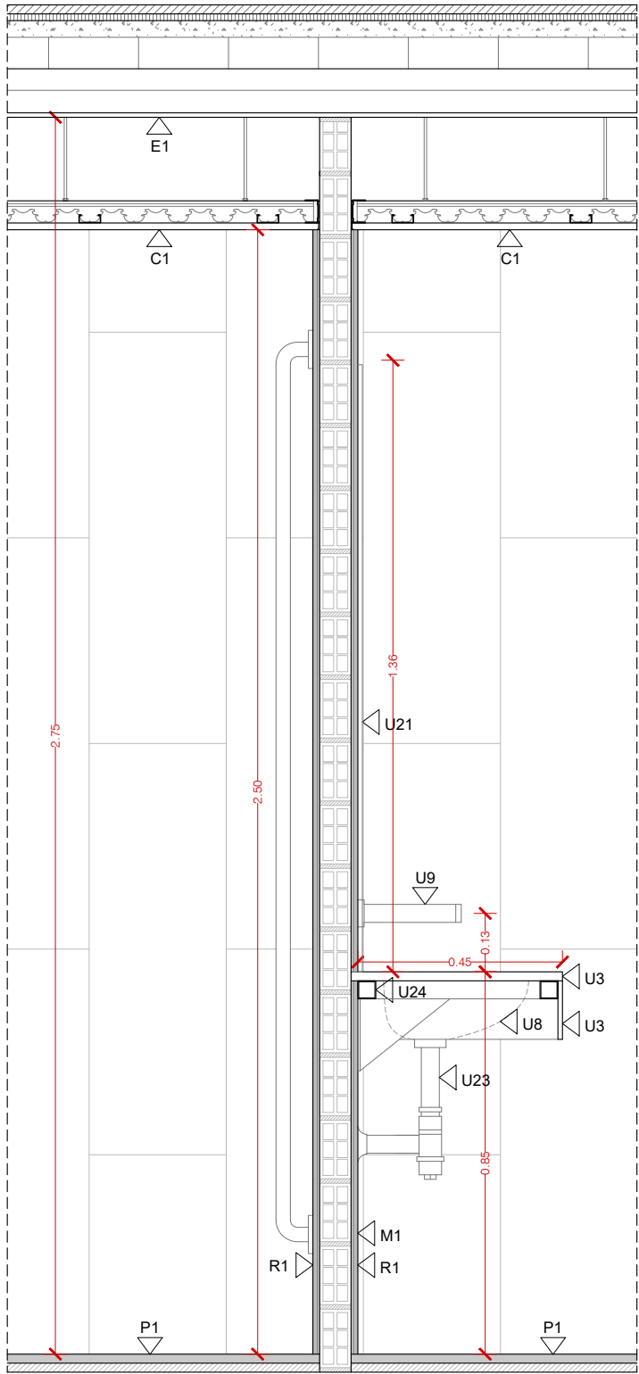
DETALL 09
