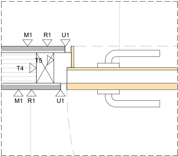
DETALL 02.1
