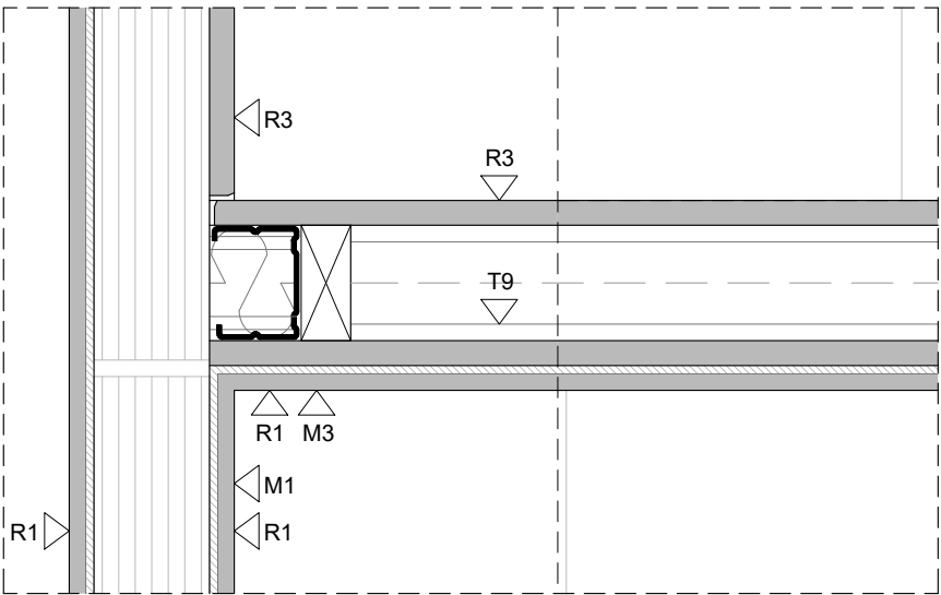
DETALL 04.1
