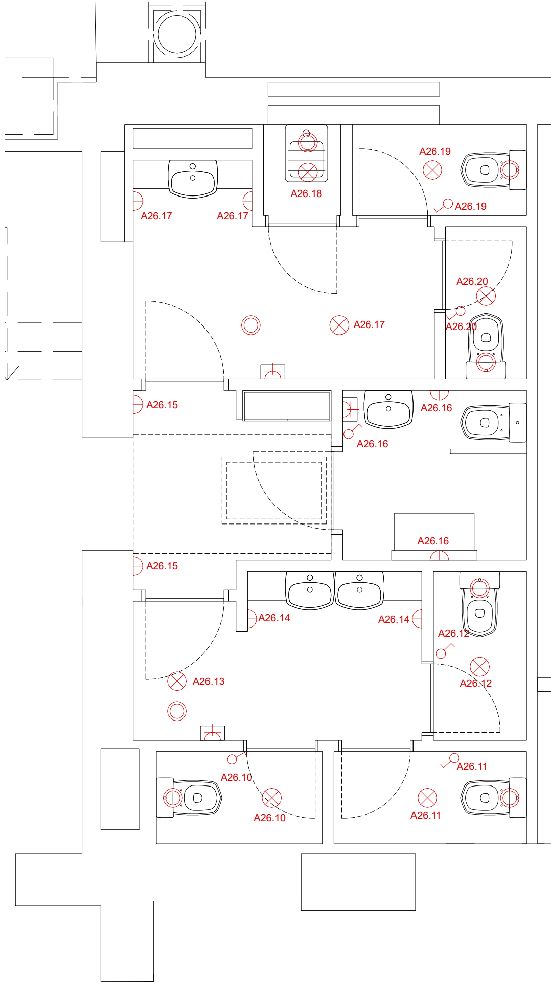
PLANTA INSTAL·LACIONS ELÈCTRICA I D'ENLLUMENAT
