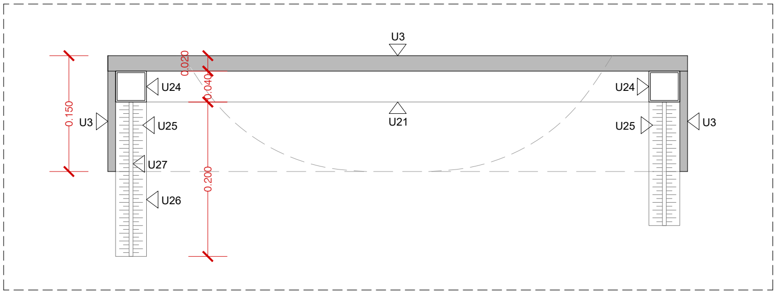
DETALL 09.2
