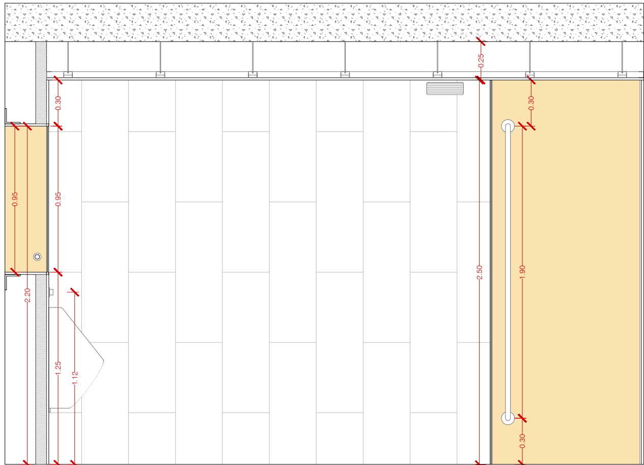
ALÇAT 04
