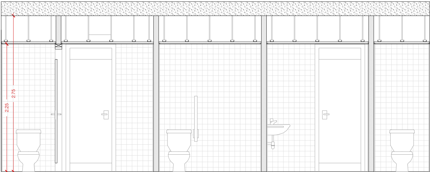
SECCIÓ LONGITUDINAL SL2
