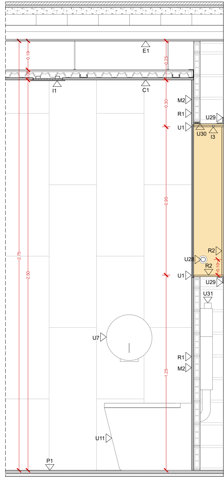
DETALL 05
