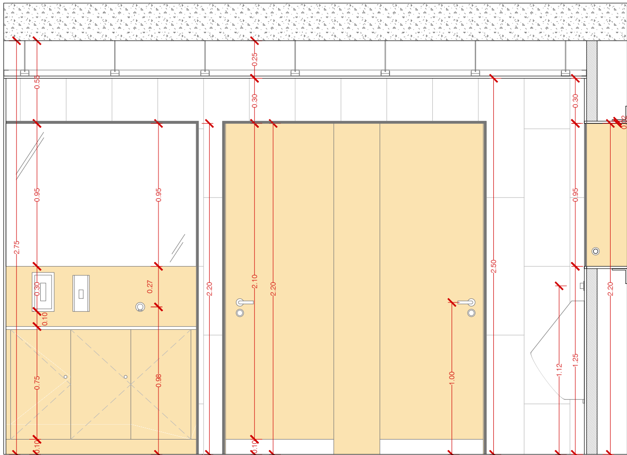
ALÇAT 03
