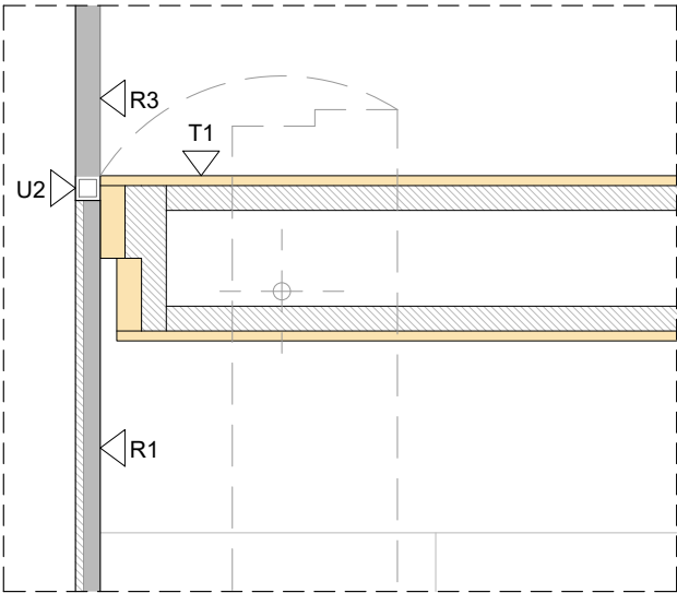
DETALL 02.1
