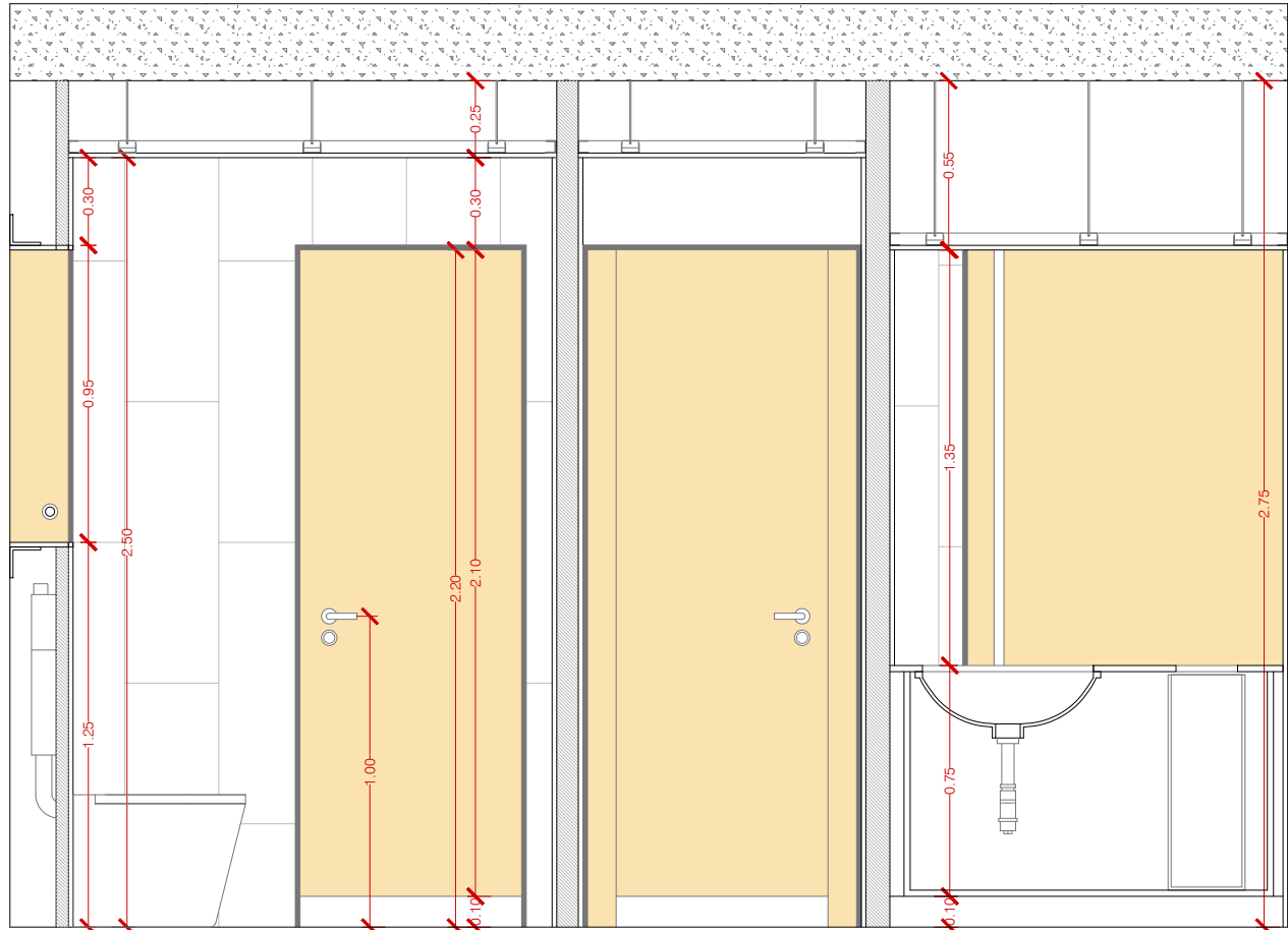
ALÇAT 02
