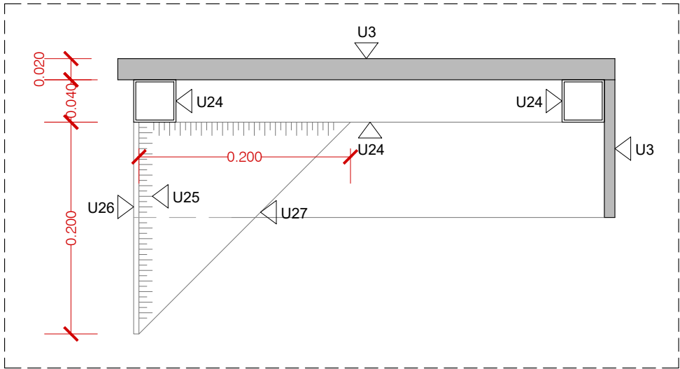
DETALL 09.3
