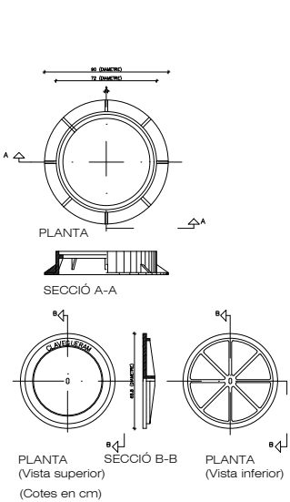
Tapa circular de registre amb marc circular
