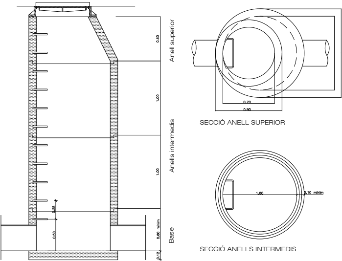
Pou de registre circular prefabricat Ø 1m
