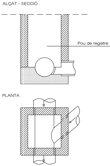
Unió tipus de conductes
