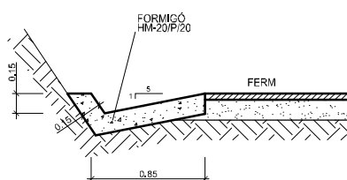
DETALLS CUNETA ESCALA 1/50
