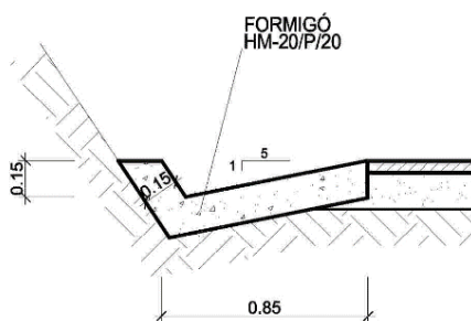
Figura 1. Detall cuneta.
